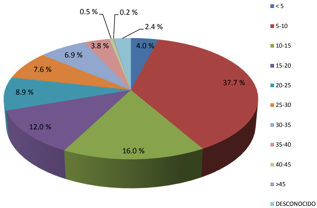
Figura 3.19 Gráfica de la longitud de claro máximo de los puentes en el estado de Guanajuato (IMT Y SOP)
