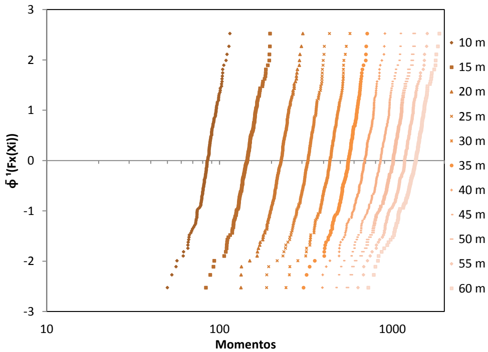
Figura 3.100 Gráfica de distribución de probabilidad lognormal para momentos considerando presencia múltiple y un carril de circulación para caminos secundarios
