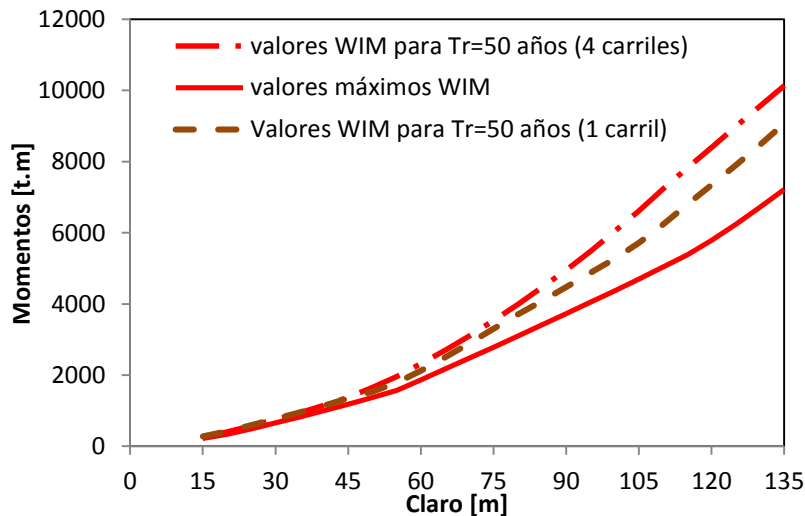
Figura 3.67 Gráficas comparativas entre los valores calculados para el periodo de retorno de 50 años de los elementos mecánicos (a) cortantes y b) momentos) considerando presencia múltiple para uno y cuatro carriles
