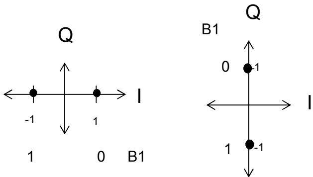
Figura 3-3 Constelación de la modulación BPSK.
