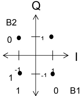
Figura 3-4 Constelación de la modulación QPSK.
