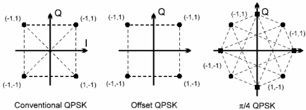
Figura 13. Modalidades de QPSK
