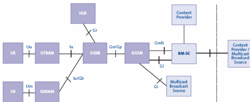
Figura 50. Nodos involucrados en la arquitectura MBMS
