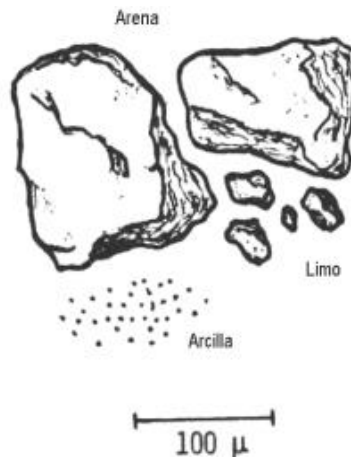
Figura 27. Comparativa del tamaño granulométrico para la identificación de suelos
