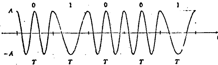
Señal FSK
