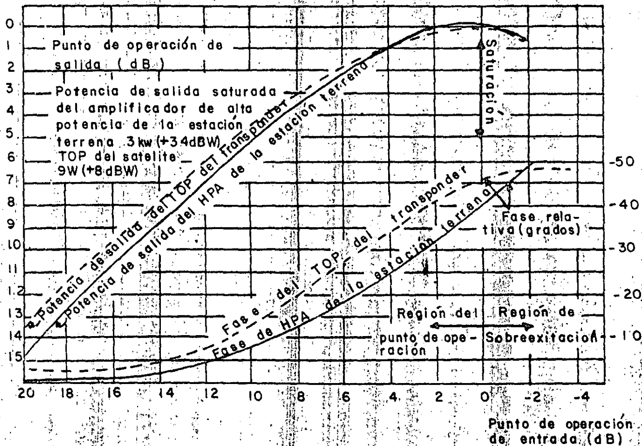
Fig (19) Características de amplitud y fase de un HPA de una estación terrena típica y el TOP del transponder de un satélite empleado en el sistema INTELSAT -V-TDMA 6/4 GHz.
