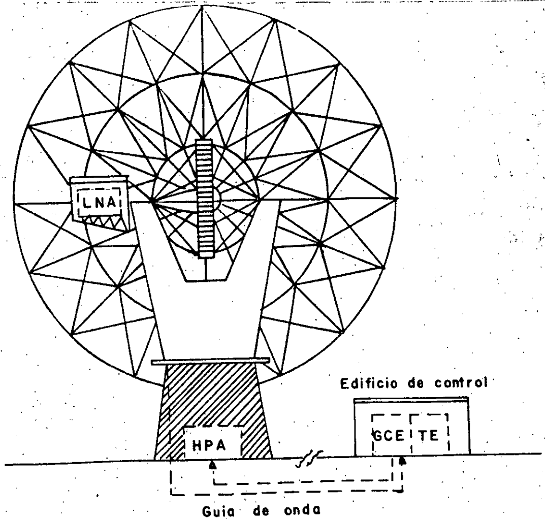
Fig. 3 Estación terrena de gran tamaño que emplea una antena tipo Cassegrain.
