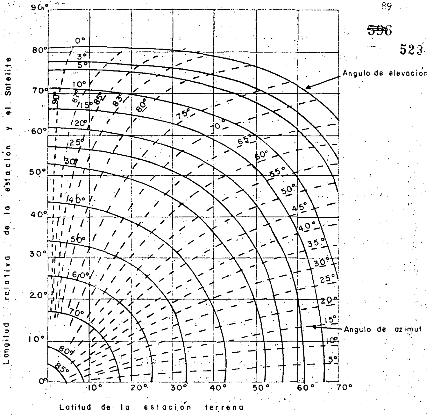
Fig. 22. Gráfica para obtener los ángulos de elevación y azimut de un satélite.
