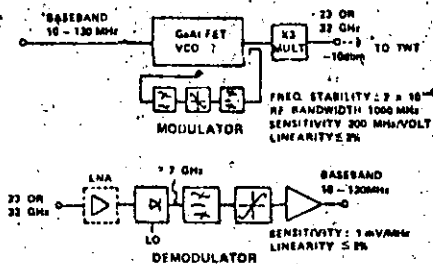
Fig. 4. ISL modem.
