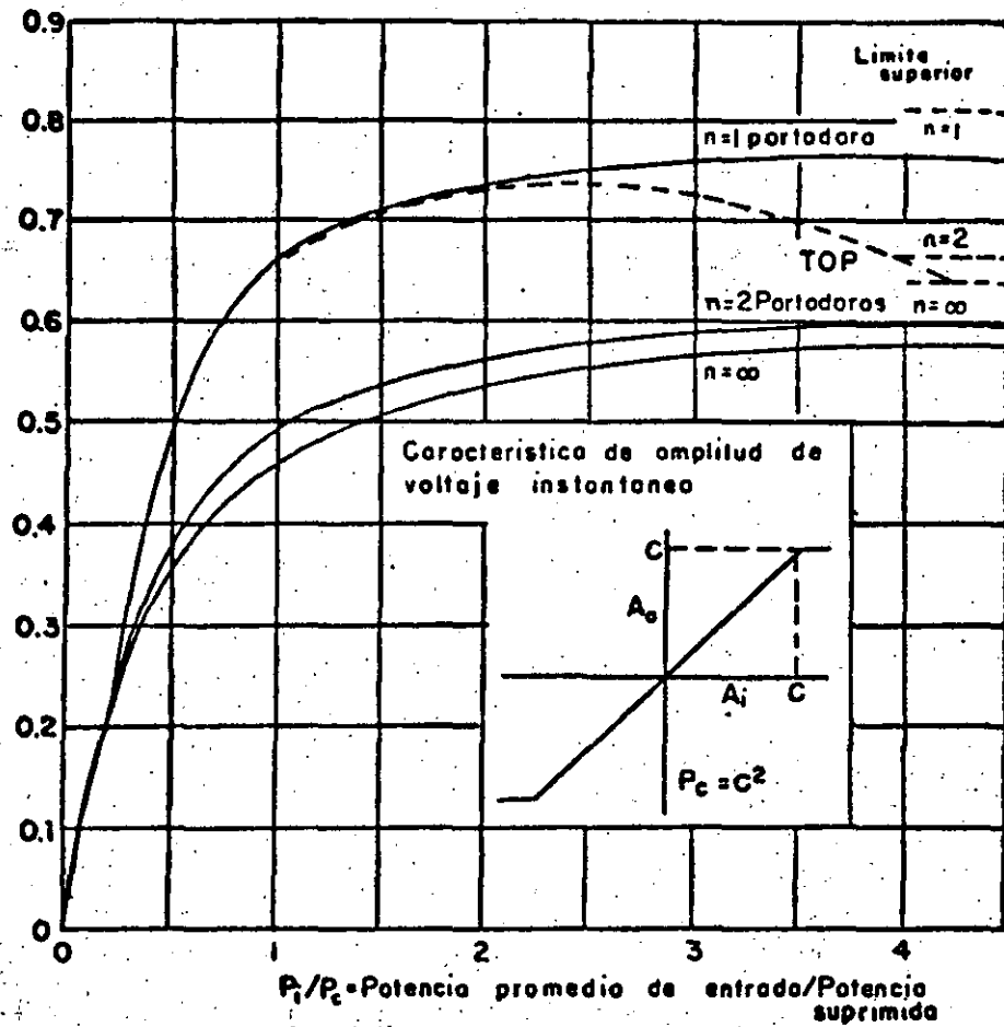
Fig. (4.11) Características de transferencia de la potencia no distorsionada de un amplificador no lineal con la representación de un limitador ideal de las características de amplificación de voltaje instantaneo, para la transmisión de una y varias portadoras.
