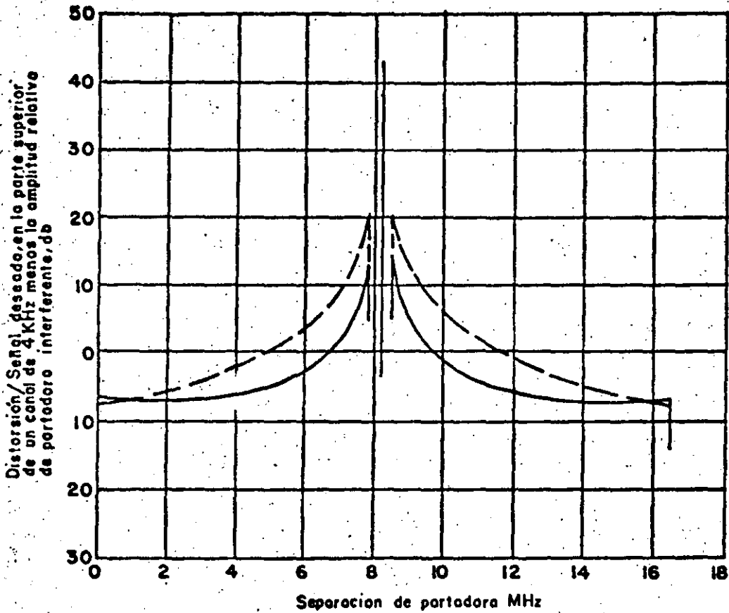
Fig. (4.9) Comparación de la distorsión debido a una portadora interferente no modulada en un sistema de 1800 canales con preénfasis (línea continua) y sin preénfasis (línea discontinua). La gama de separación de portadoras es de 0 a dos veces la máxima frecuencia modulante
