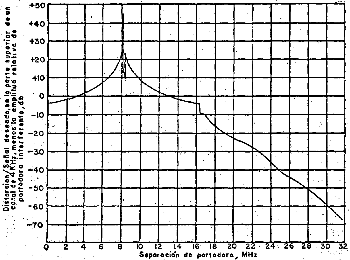
Fig. (4.7) Distorsión debida a una portadora interferente modulada en un sistema de 1800 canales (se -- supone una característica de limitación ideal y no se emplea preénfasis)
