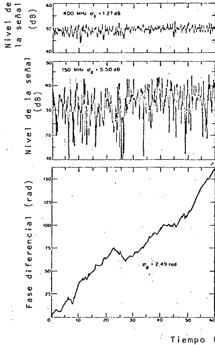
Fig. 29 Nivel de la señal y fluctuaciones de fase para un intervalo de observación de 1 min.
