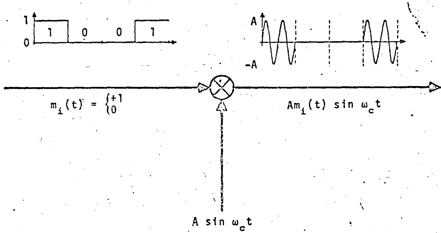
FIGURA N° 18 MODULACION ASK
