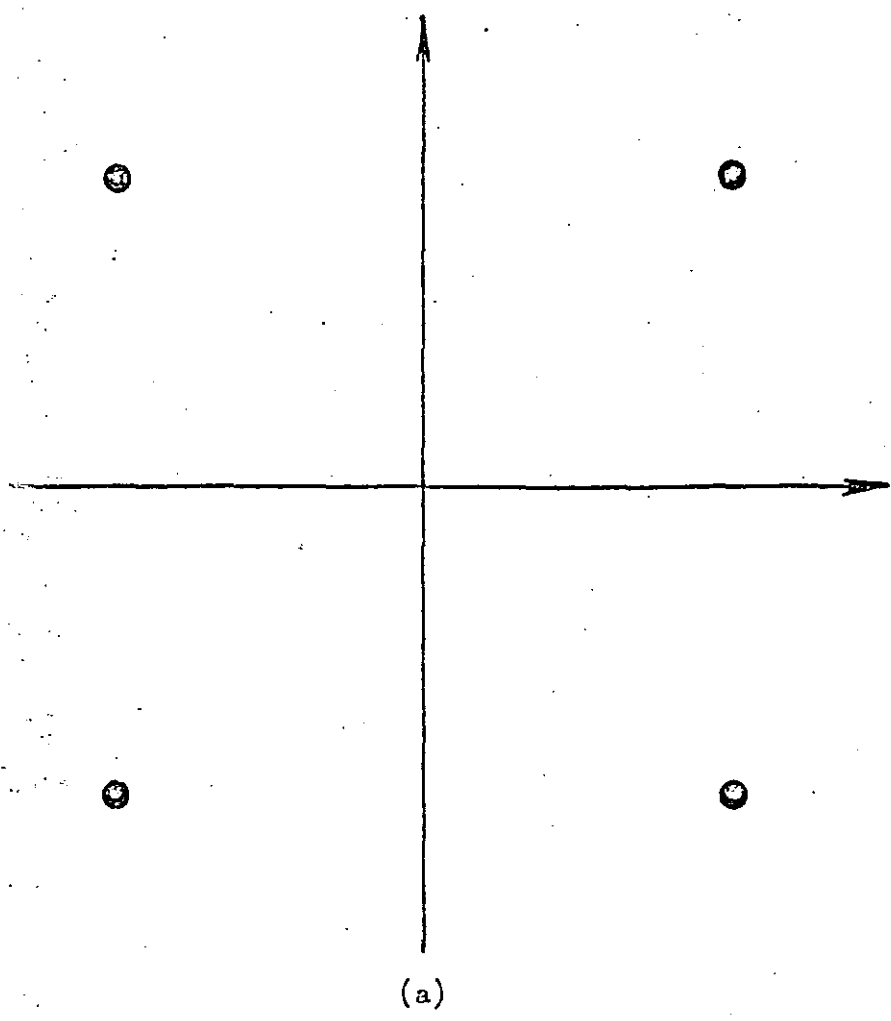
FIGURA No. 27 CONFIGURACION DE SEÑALES QPSK.
