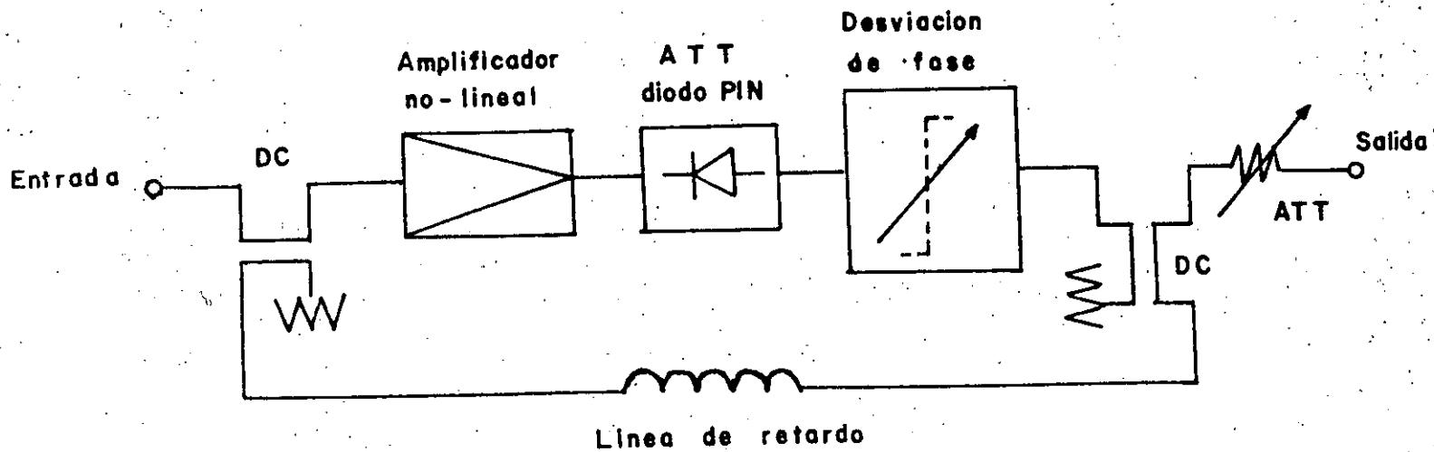
FIG. 9.- Configuración típica de un generador de distorsiones no lineal.
