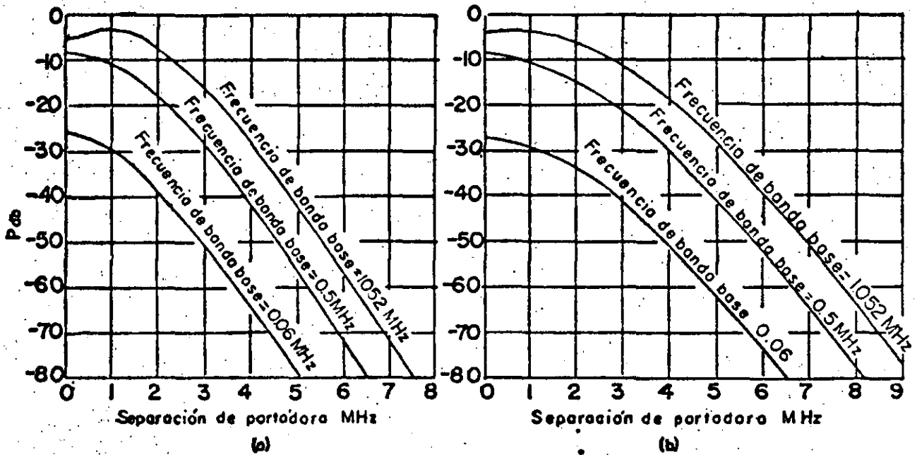
Fig. (4.1) Distorsión debido a una portadora interferente en un sistema de 240 canales telefónicos con un limitador ideal. La razón distorsión/señal es P + 20 \log_{10} r dB. (a) Portadora sin modular (b) Portadora modulada
