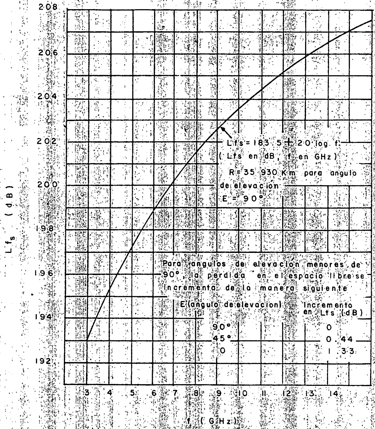
Fig. (21) Pérdida por trayectoria en el espacio libre.
