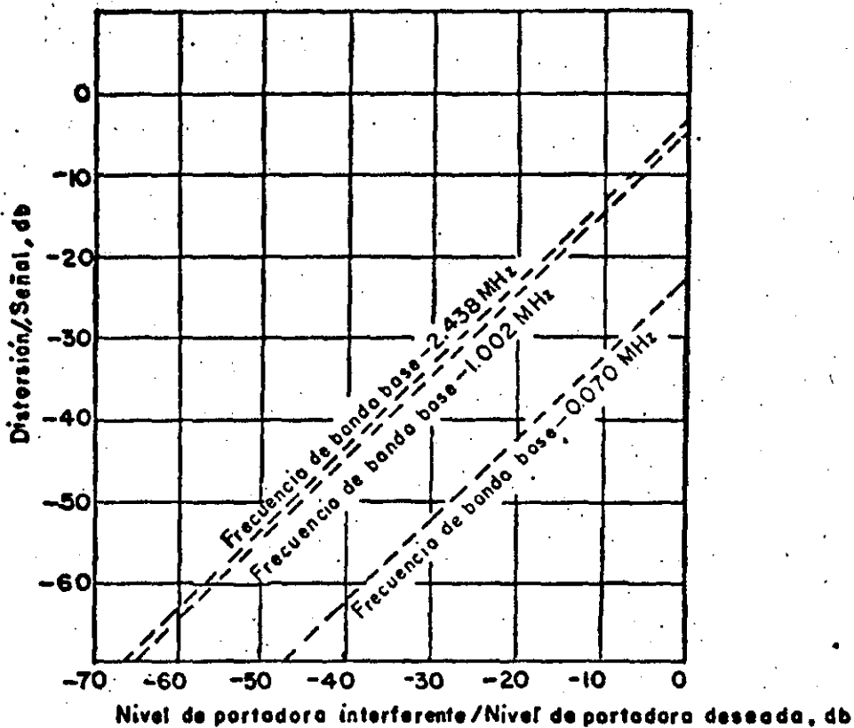
Fig. (4.3) Variación del nivel de distorsión medido con un nivel de portadora interferente para un sistema de 600 canales. La separación frecuencia de la portadora es de 0 Hz. La portadora interferente está sin modular.
