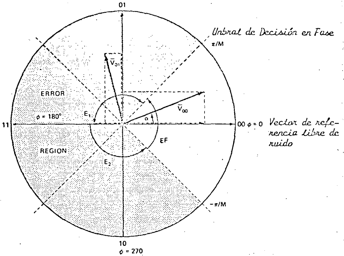
FIGURA N° 42 Región de Error en Demoduladores Coherentes. iii 4ary. PSK.
