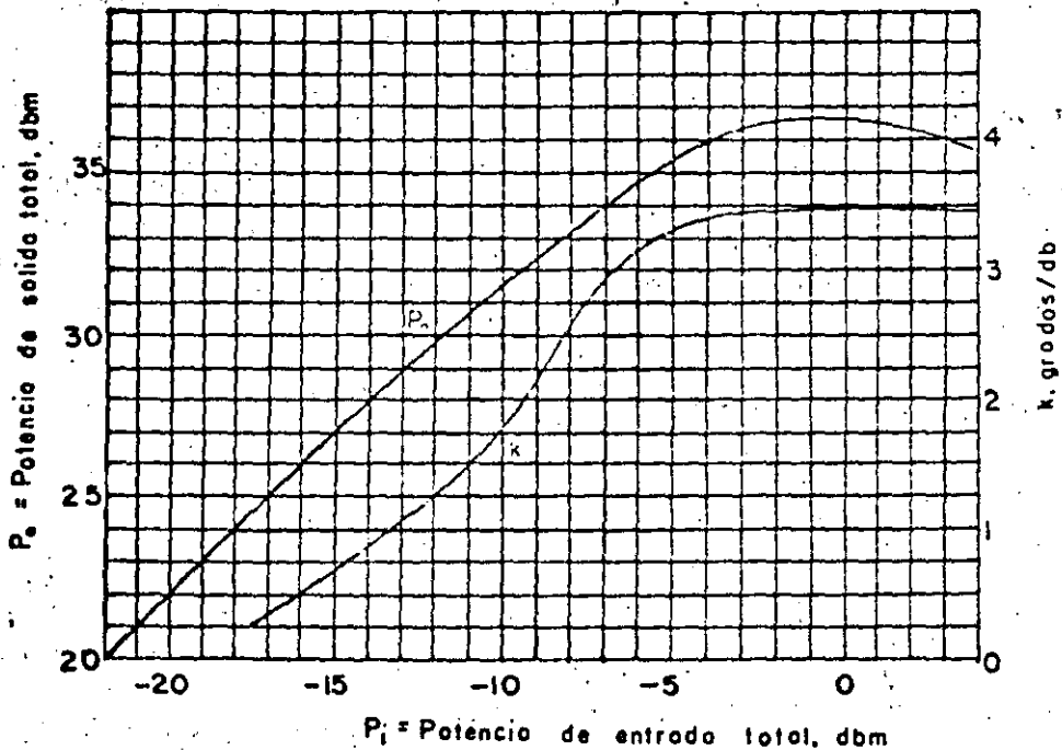
Fig. (4.10) Características de transmisión de una sola potencia de portadora y factor de conversión AM/PM para un potencial de hélice de 1525 volts.
