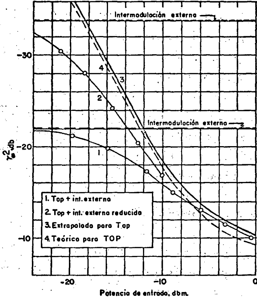
Fig. (4.17) Razón de intermodulación teórica en función de las medidas para una entrada de ruido aleatorio plano
