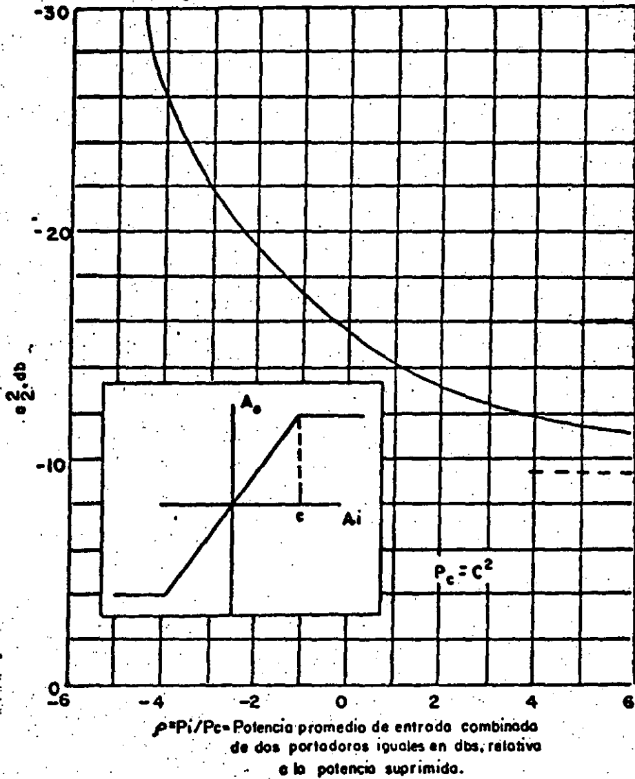
Fig. (4.12) Productos de intermodulación de tercer orden de las frecuencias 2f_1 - f_2 y 2f_2 - f_1 para dos portadoras de entrada de igual amplitud
