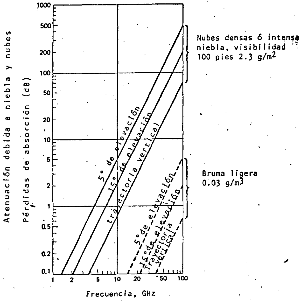
Típica absorción debida a niebla, bruma y nubes.
