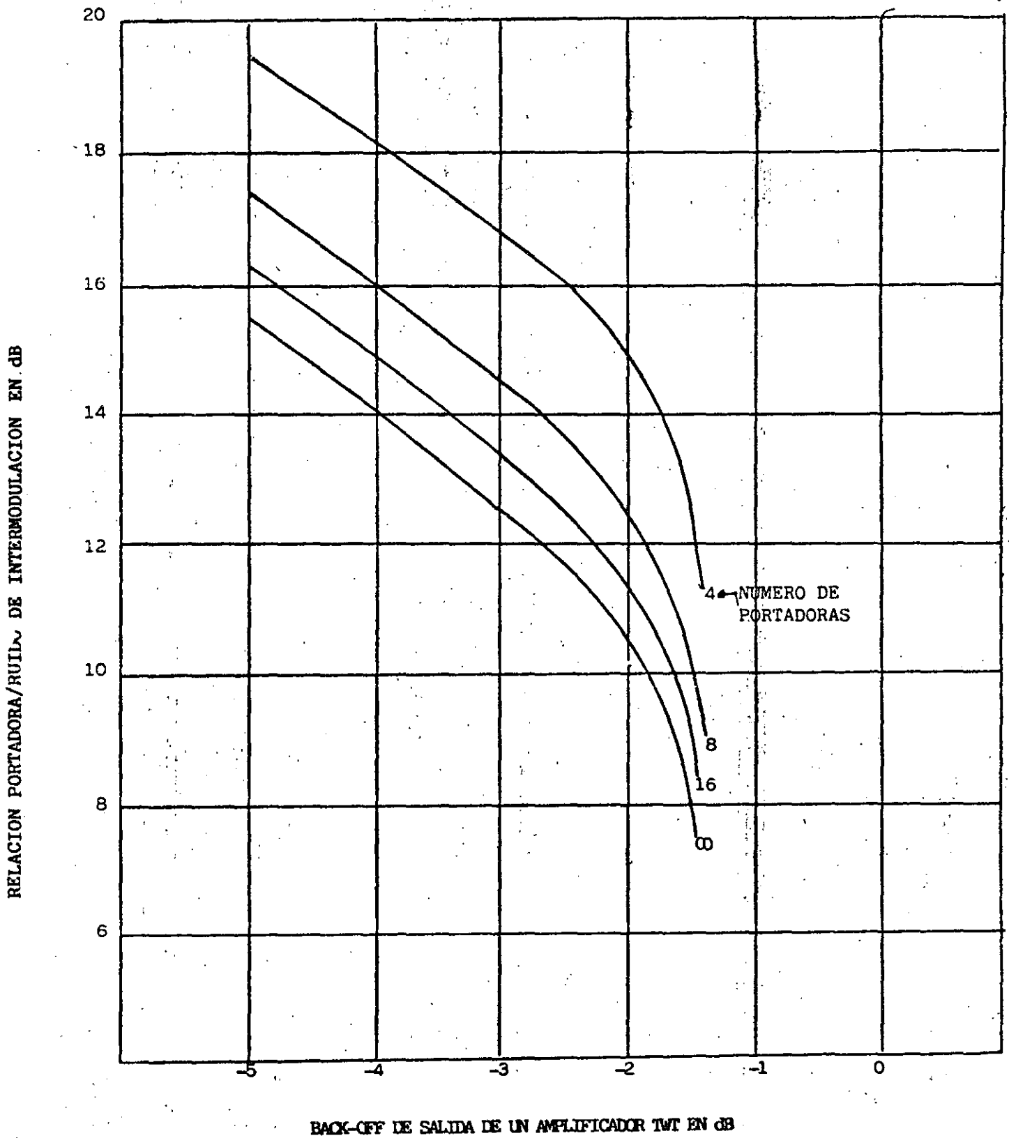
FIG. 1 RELACION PORTADORA/RUIDO DE INTERMODULACION EN FUNCION DEL BACK-OFF PARA UN AMPLIFICADOR TWT TIPICO
