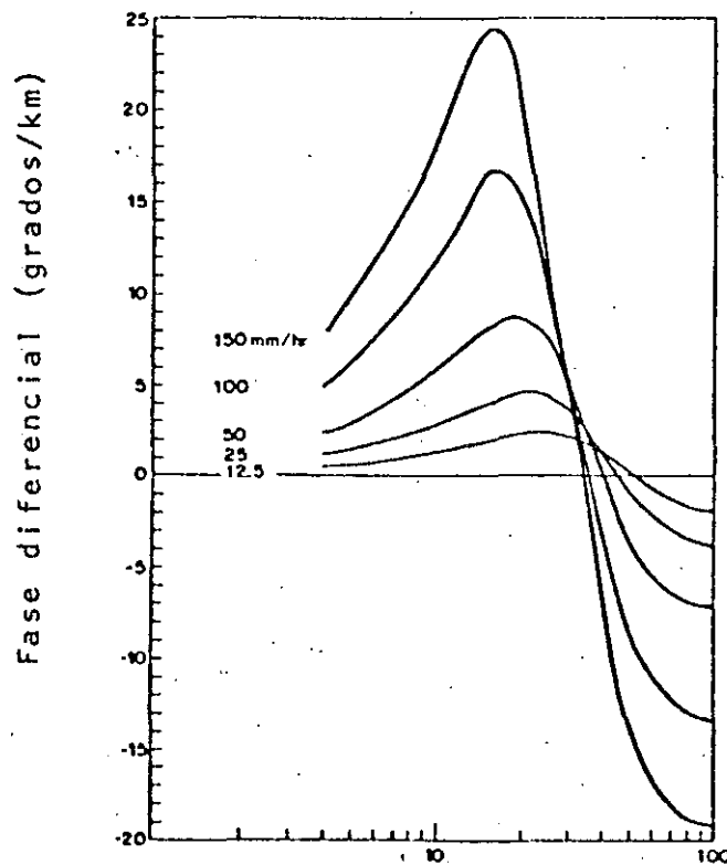
Fig. 34 Atenuación y fase diferencial entre polarizaciones I y II para varias intensidades de precipitación.
