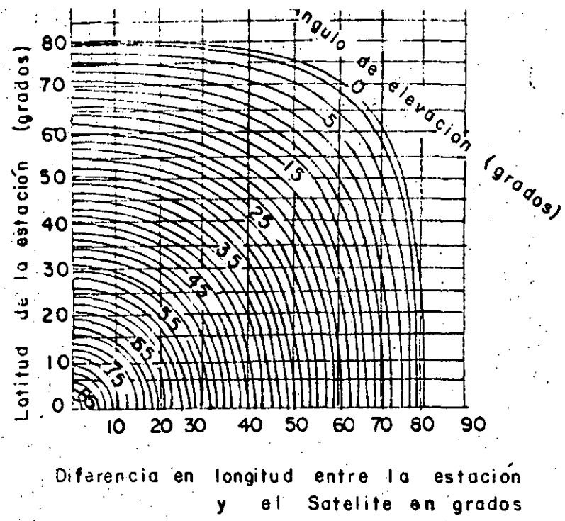
Fig. 20. Gráfica para obtener el ángulo de elevación.
