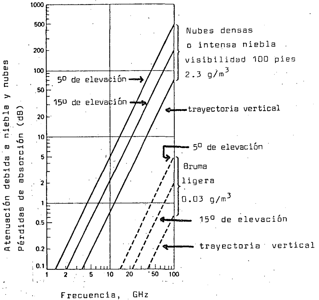
Típica absorción debida a niebla, bruma y nubes
