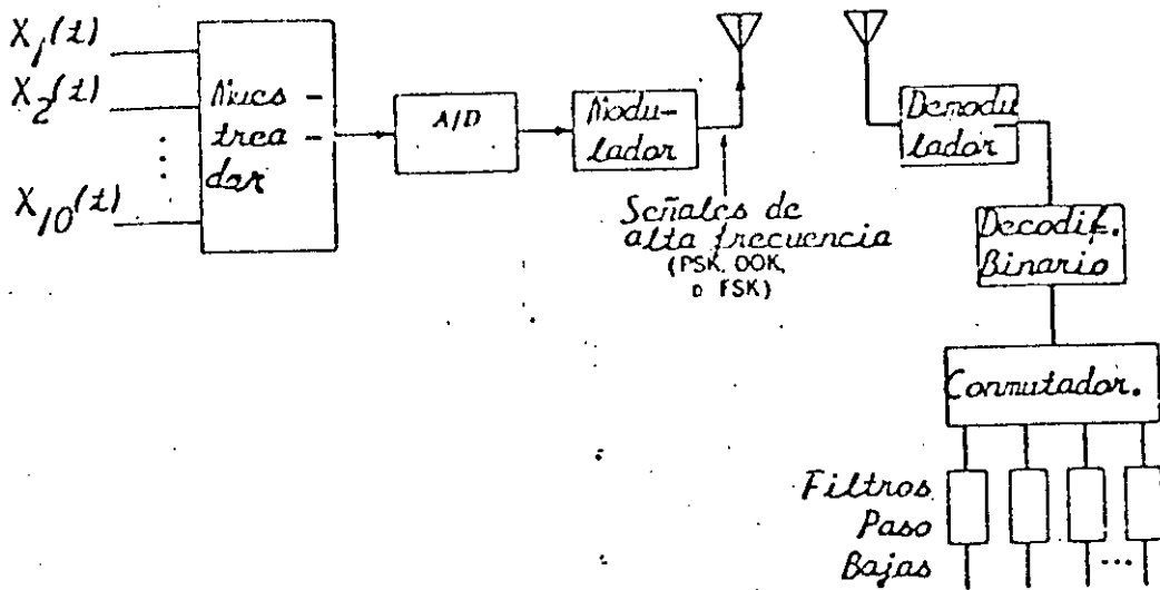
FIGURA N° 26 a: Sistema PCM Completo
