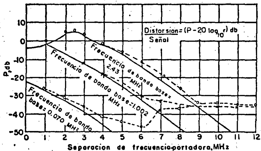
Fig. (4.4) Variación del nivel de distorsión medido con una separación de la frecuencia portadora para un sistema de 600 canales. El nivel de la portadora interferente sin modular es mucho menor que el nivel de la portadora deseada.
