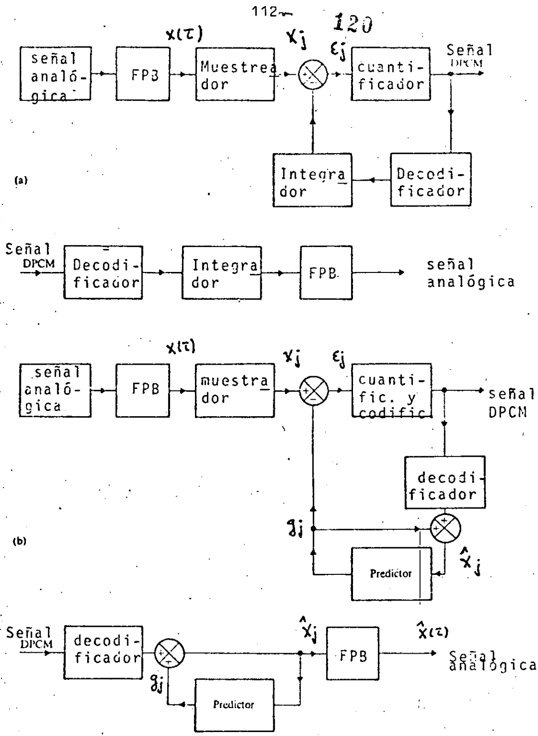
FIGURA N° 15 DIAGRAMA EN BLOQUES DEL SISTEMA PCM DIFERENCIAL: a) Transmisor y receptor de un sistema PCM simple; b) Transmisor y receptor de un sistema PCM con predictor.
