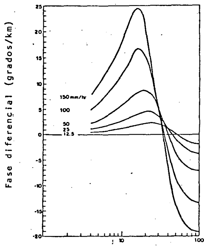
Fig. 34 Atenuación y fase diferencial entre polarizaciones I y II para varias intensidades de precipitación.
