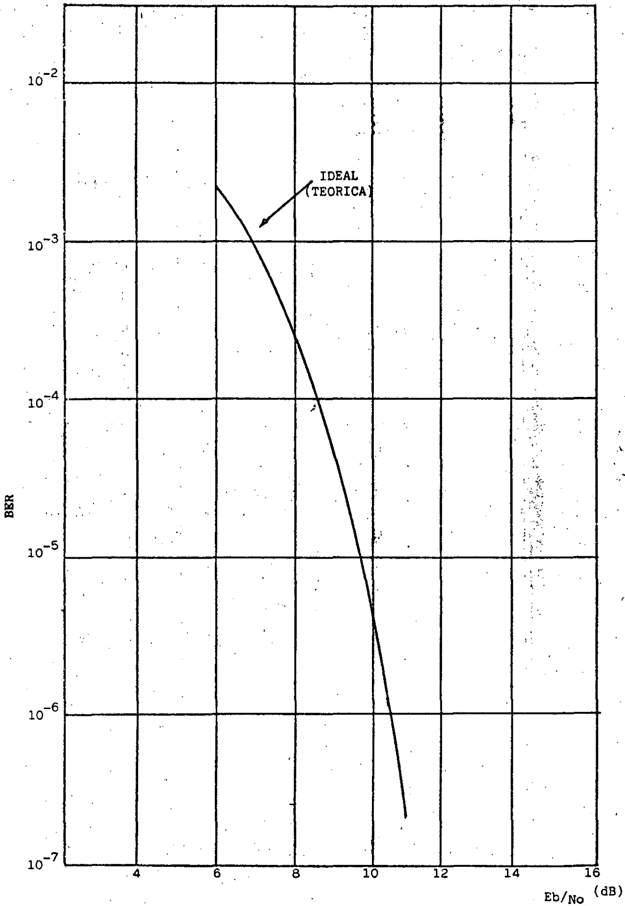
FIG.2 BIT ERROR RATE PARA UN MODEM SCPC-PSK
