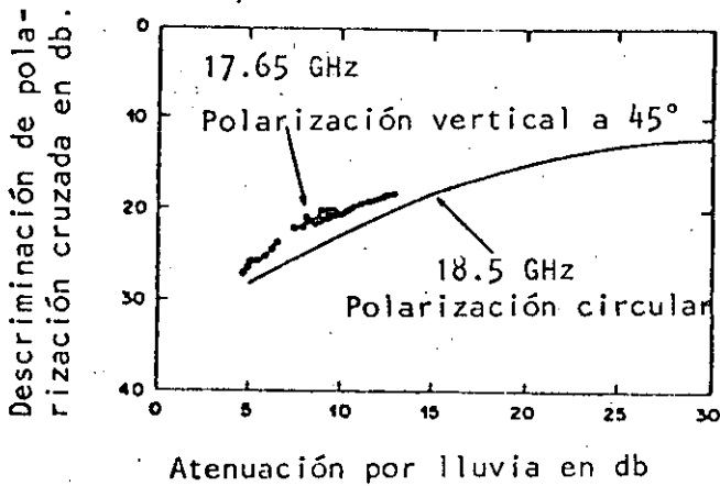
Fig. 36 Depolarización medida contra atenuación para polarización circular y polarización lineal a 45°.
