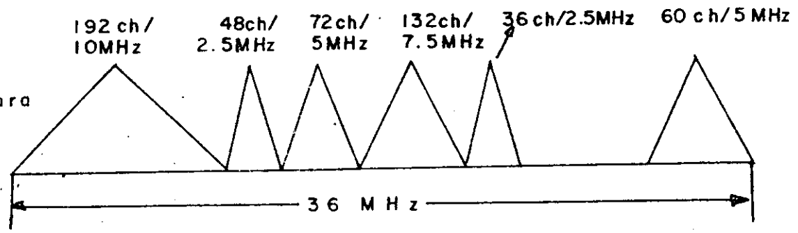
Fig.(7) Ejemplo de un arreglo en frecuencia aplicado al sistema del satélite INTELSAT IV-A con una interrelación combinada de frecuencia.
