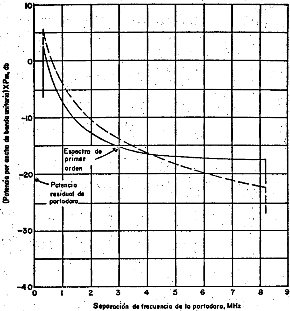
Fig. (4.8) Comparación del espectro de primer orden para una señal modulante de 1800 canales con preénfasis (línea continua) sin preénfasis (línea discontinua)
