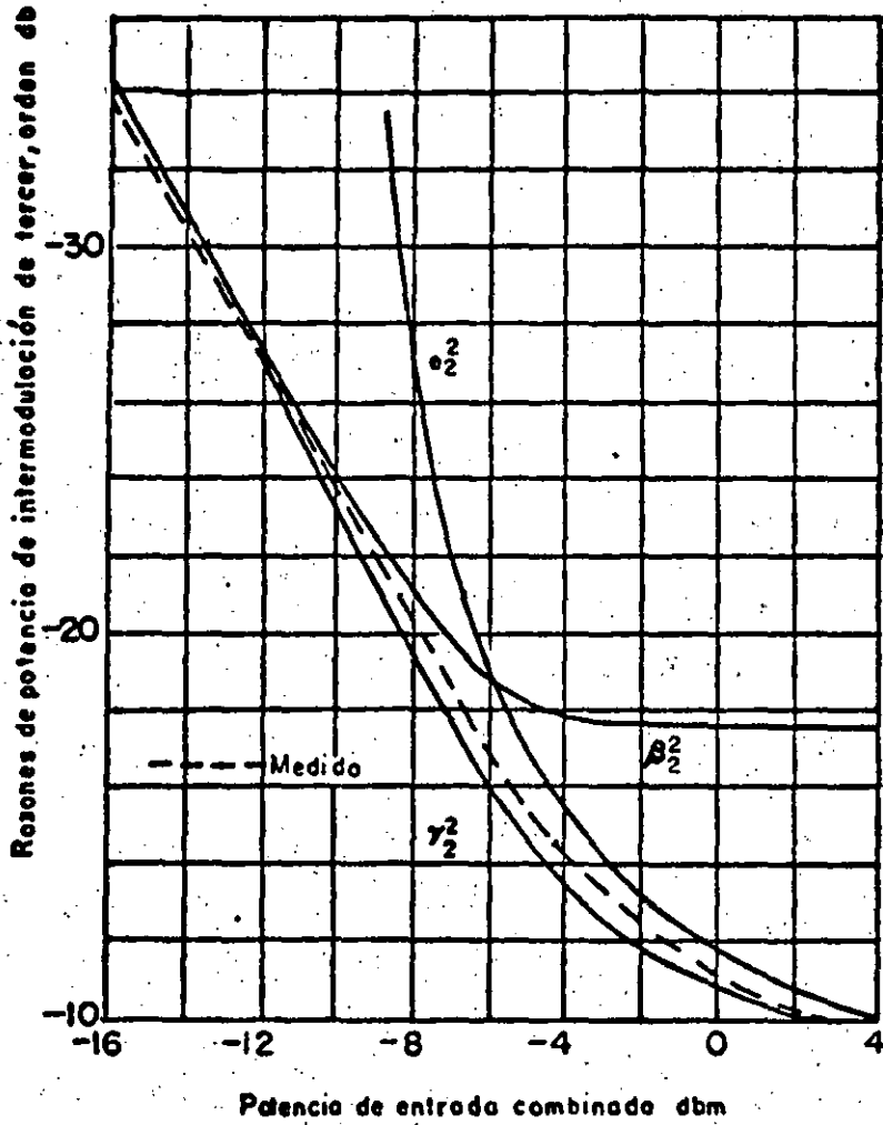
Fig. (4.15) Productos de intermodulación de tercer orden para una entrada de dos portadoras de igual amplitud
