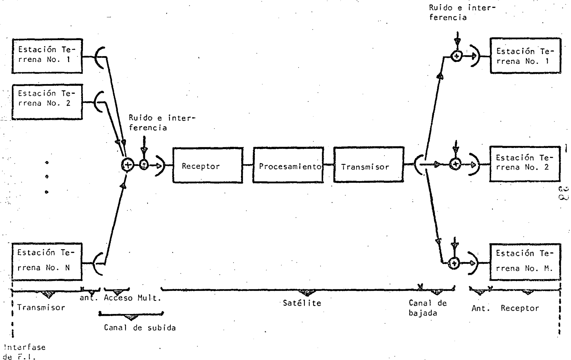
Fig. 25 Modelo de un sistema de comunicación (FI- a FI)
