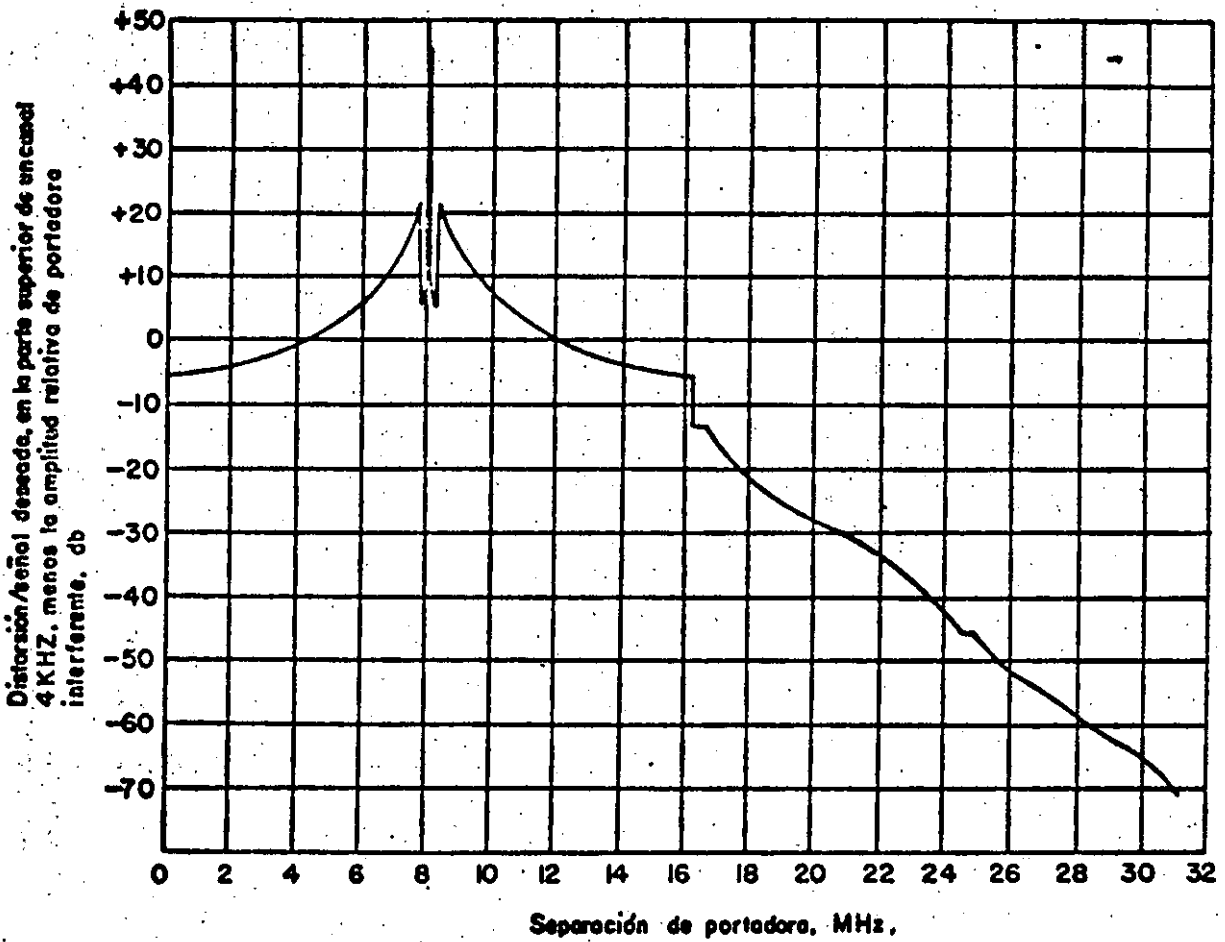
Fig. (4.6) Distorsión debida a una portadora interferente no modulada en un sistema de 1800 canales (se supone una característica de limitación ideal y no se emplea preénfasis).
