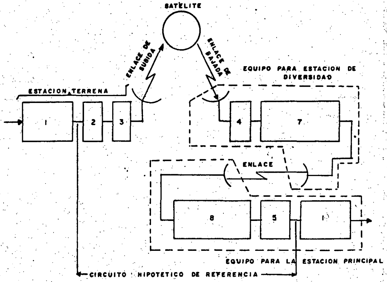
b) Caso donde se incluye una estación de diversidad. Fig.(1) Circuito Hipotético de referencia.
