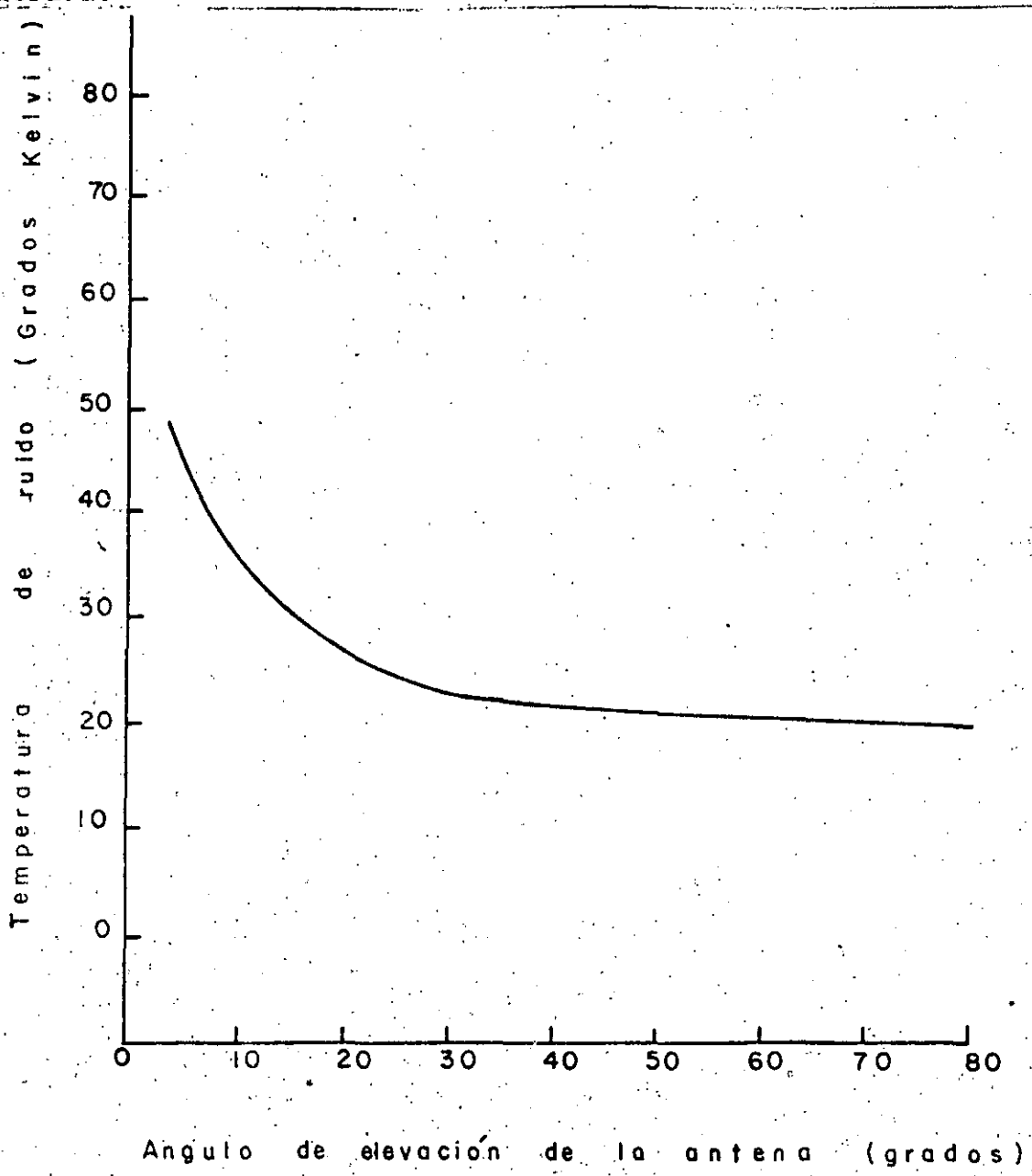
Fig. 25 Temperatura de ruido de una antena parabólica en función del ángulo de elevación.
