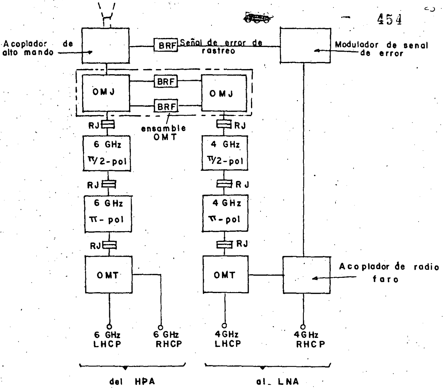
Fig. 4 Diagrama a bloques de un ensamble de alimentación para polarización ortogonal
