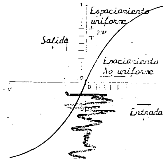
FIGURA Nº 6 Característica del Compresor no Lineal
