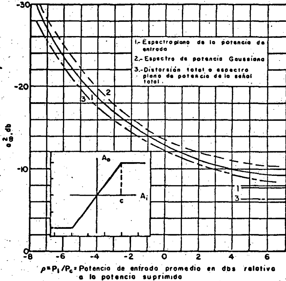
Fig. (4.13) Razón de la distorsión de intermodulación a la densidad de potencia de señal al centro de la banda de transmisión con una entrada de ruido plano.
