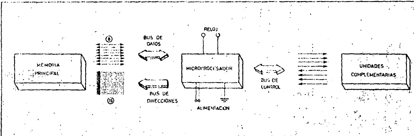
Organización externa de un microprocesador convencional de 8 bits actuando como unidad central de proceso de un sistema microordenador.
