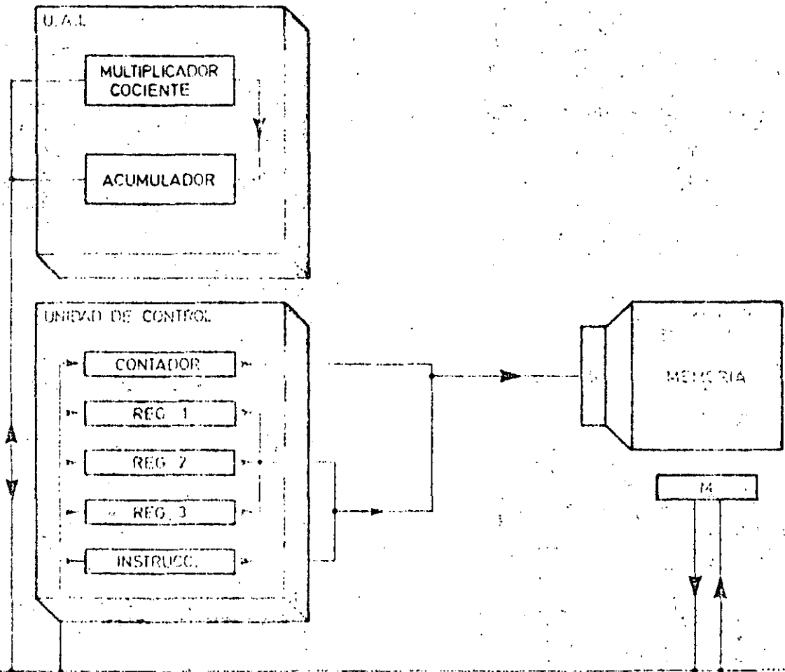
Una muestra de la CPU de un ordenador científico. Con el empleo de registros-índice y de un multiplicador-cociente se reduce el tiempo de ejecución de las operaciones, redondeando, a la vez, una gran precisión en los resultados.
