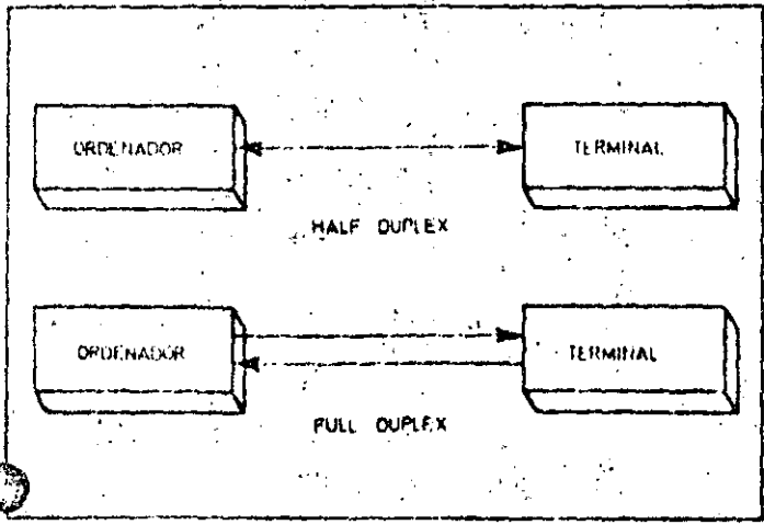
Existen dos formas mediante las cuales se comunican los terminales con el ordenador, una línea en los dos sentidos (half-duplex) y dos líneas, una en cada sentido (full-duplex).
