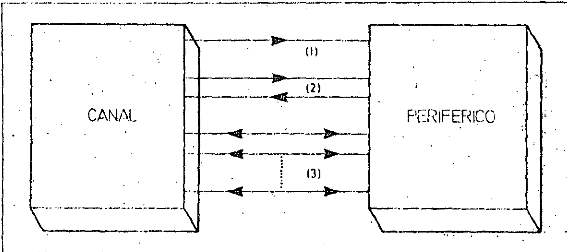
Esquema básico de la estructura de un br de adaptación (interface) genérico: (1) señal de lectura/escritura; (2) líneas para la sincronización de operaciones de transferencia; (3) líneas de transferencia de información.
