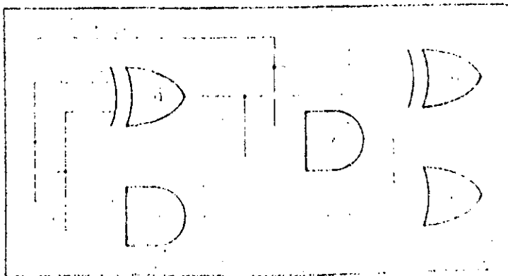
Realización práctica, mediante puertas lógicas, de un circuito sumador de tres bits con salida de suma (Y) y de acarreo (Z)
