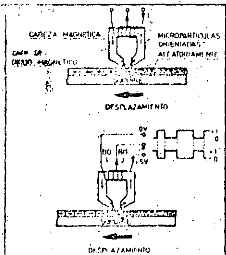
Escritura de informaciones en un disco magnético. La bobina emite un campo magnético que orienta las partículas que desfilan bajo el entrehierro. Este campo es creado en las bobinas por efecto de la circulación de la corriente.
