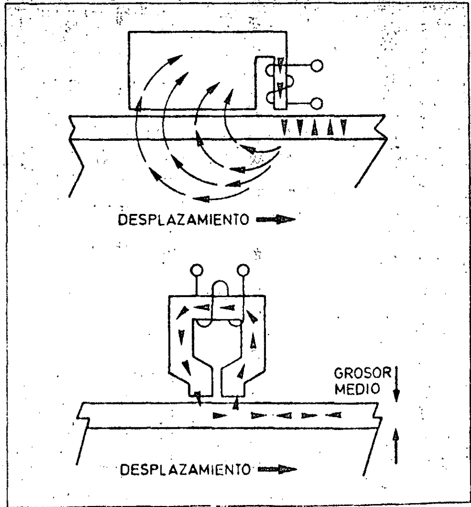
Otra de las características de los discos magnéticos es el sistema de grabación empleado: vertical (gráfico superior) o longitudinal (gráfico inferior), denominación que deriva de la orientación con la que se graba la información en el material magnético.
