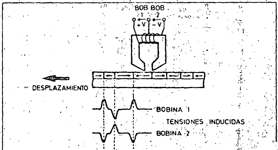
La lectura del disco se realiza la cabeza captando en el entrehierro el campo magnético variable originado por la distinta orientación de las partículas sobre el medio magnético.
