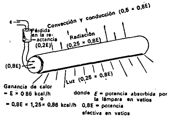
FIG. 31. Conversión de la energía eléctrica en calor y luz en las lámparas fluorescentes
