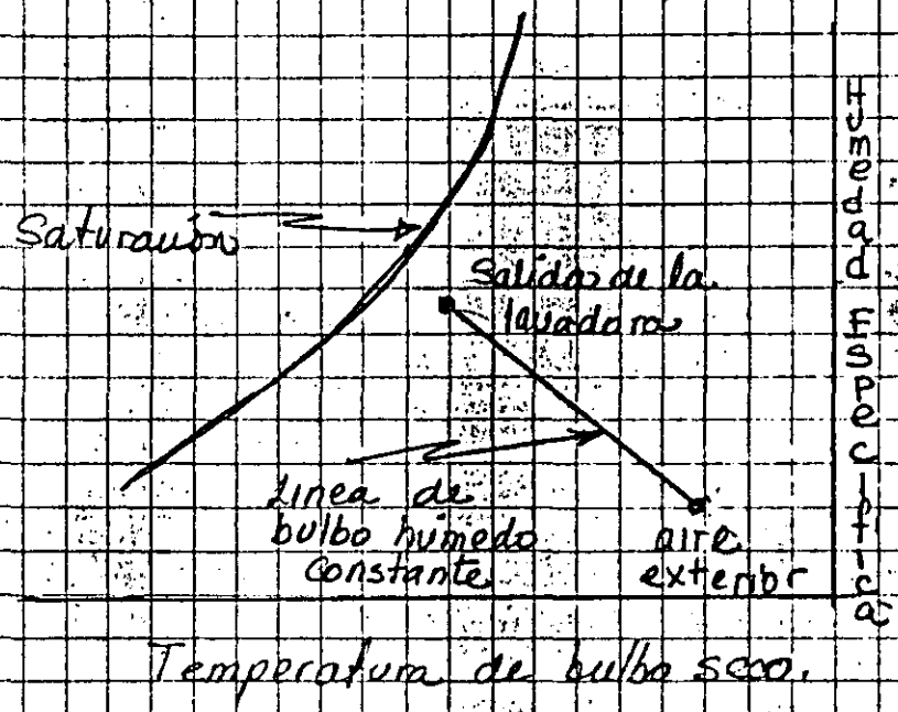
Proceso de enfriamiento evaporativo Figura. 12
