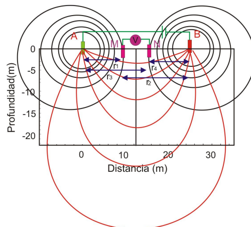
Figura 2.1. Líneas de corriente (rojo) y de potenciales.
