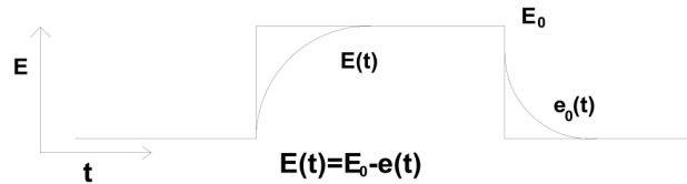
Figura 2.19. Voltaje de entrada y decaimiento en un medio polarizable debido a una onda cuadrada de corriente. (SEG, Mining Geophysics, V2).
