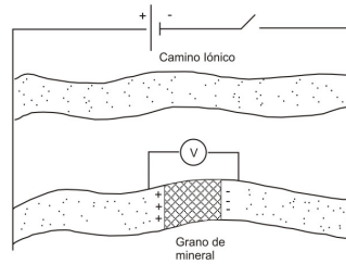
Figura 2.6. Fenómeno de polarización de electrodos en los contactos mineral-electrolitos (Orellana, 1974).
