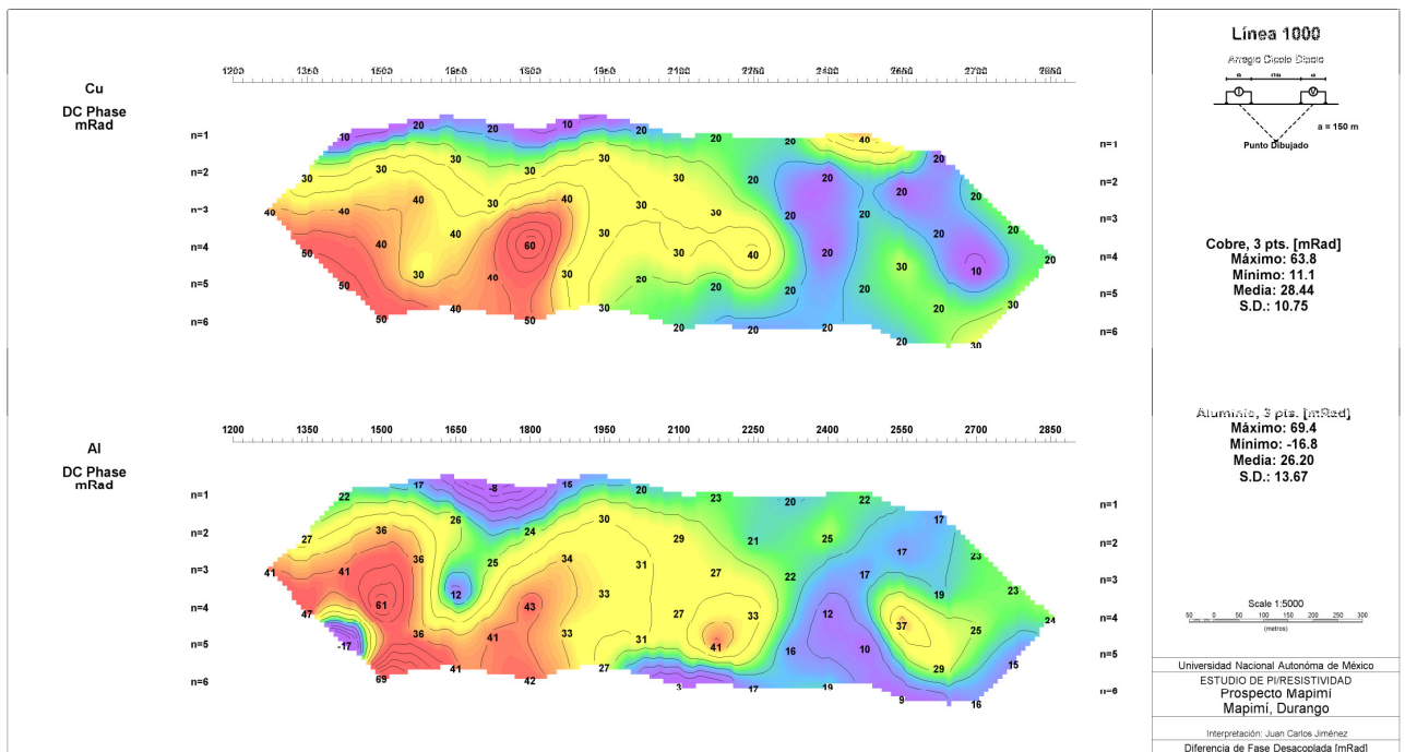
Figura 5.3. Pseudosecciones geofísicas de la fase desacoplada (3 puntos). En la parte superior se muestra el levantamiento con cobre y en la parte inferior el levantamiento con aluminio.
