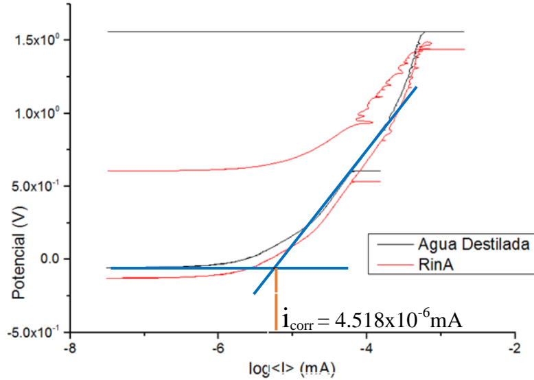
Figura 27. Curva de polarización anódica del el Acero inoxidable 316L inmerso en solución Ringer A, a temperatura de 22°C en condiciones estáticas
