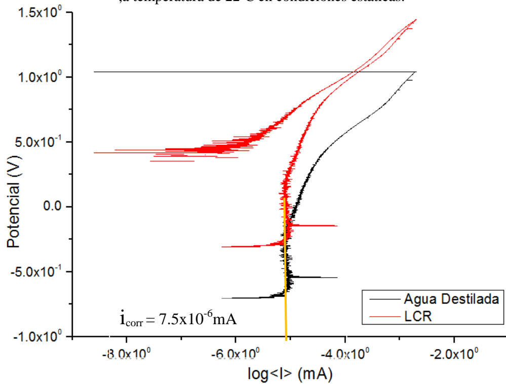
Figura 37. Curva de polarización anódica para la aleación de Ti-Al, inmerso en Liquido Cefalorraquídeo, a temperatura de 22°C en condiciones estáticas.
