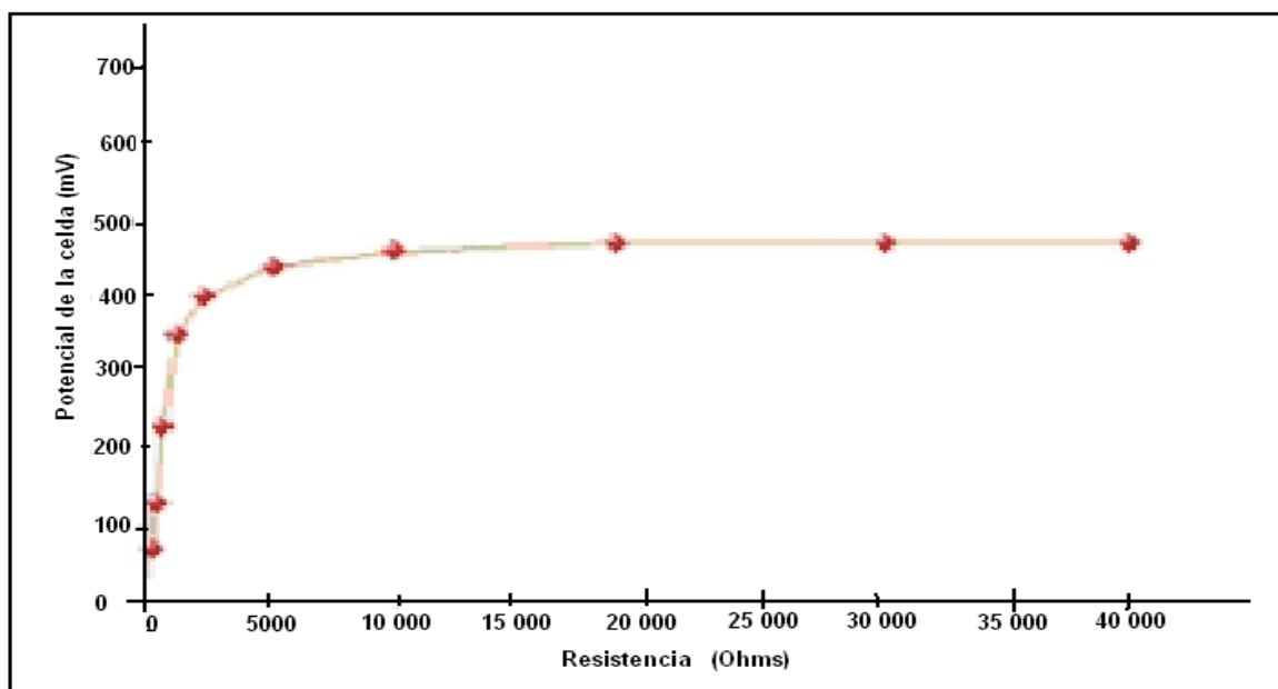
Gráfica 4.3 Voltaje obtenido variando las resistencias Fuente: Cosechando electricidad de las bacterias.
