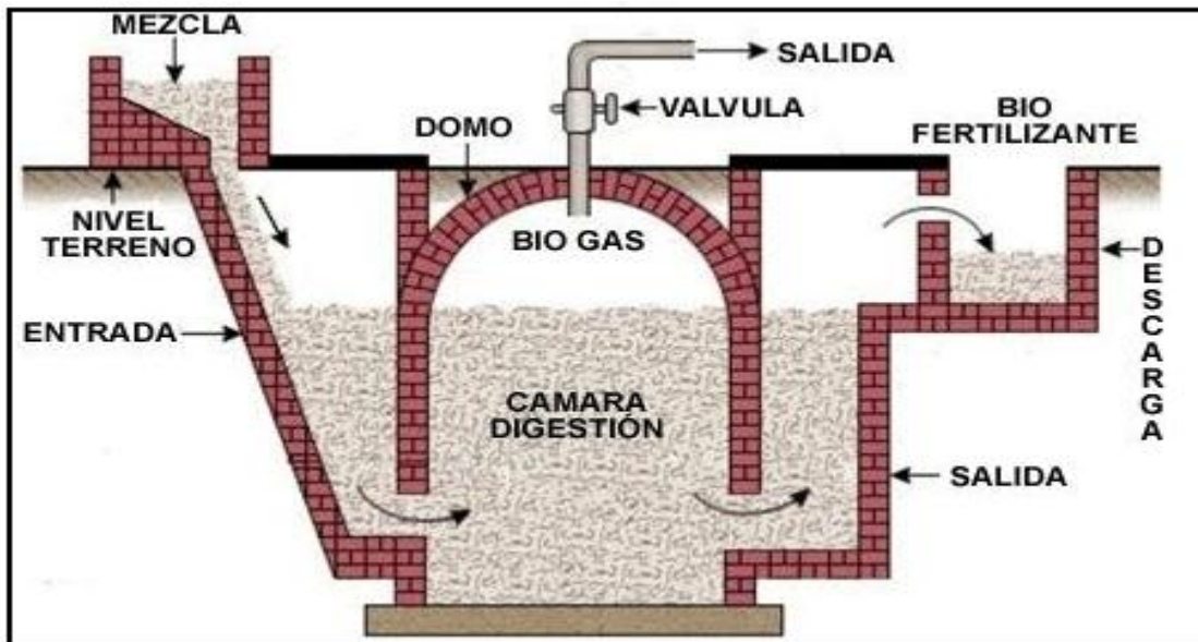
Fig. 3.1 Diagrama de funcionamiento de un biodigestor
