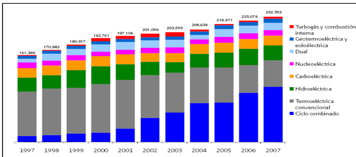
Gráfica 1.2 Generación bruta en el servicio público por tipo de central en GWh.
