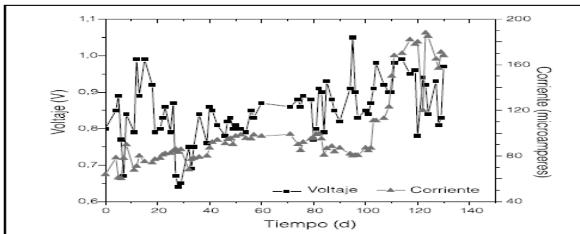
Gráfica 4.5 Esta gráfica nos muestra los valores obtenidos de voltaje y corriente obtenidos empleando Geobacter Sulfurreducens .
