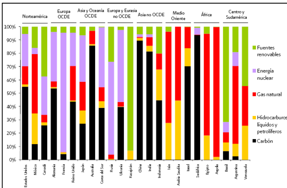
Gráfica 1.1 Participación porcentual de fuentes primarias para la generación de energía, las fuentes renovables se componen por hidráulica, eólica, geotermia y biomasa.
