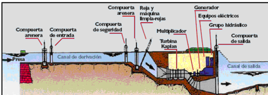
Fig. 2.2 Diagrama de una central mini hidráulica Fuente: Energías renovables para todos. Tomo Hidráulica
