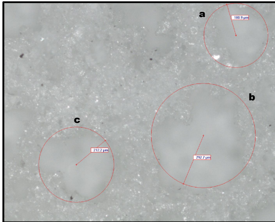
FIGURA 4.9 Poros medianos y poros grandes, la imagen fue obtenida con un microscopio óptico con un aumento de 50X. a) 180.9 \mu\text{m} , b) 292.7 \mu\text{m} , c) 212.2 \mu\text{m}
