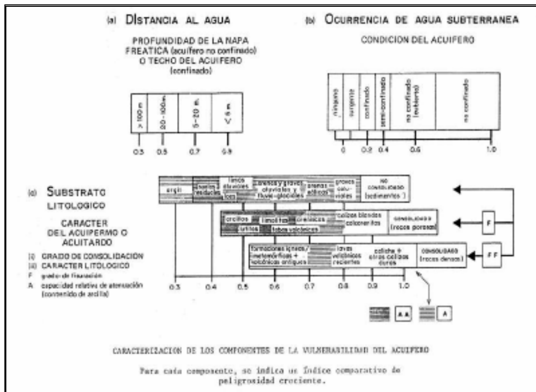
Figura 12. Diagrama para el método GOD
