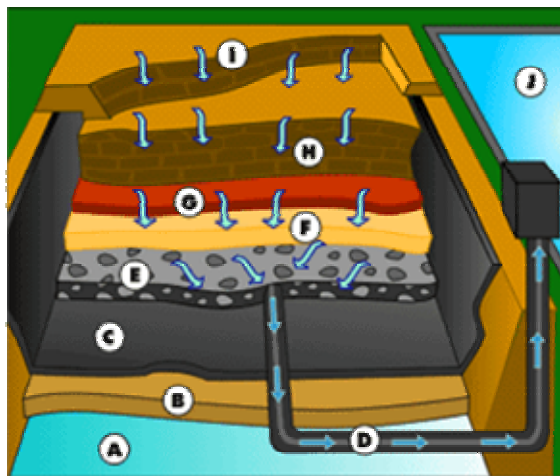
Figura 6. Estructura de un relleno sanitario Fuente: www.dropofoil.com
