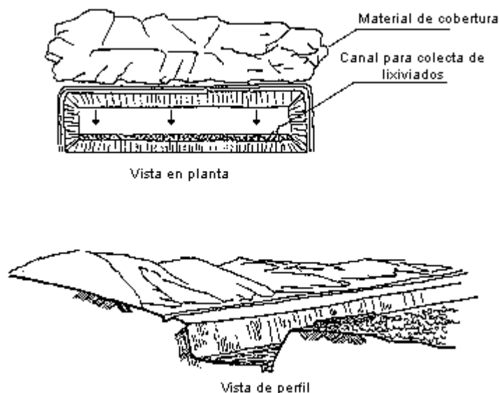
Figura 7. Relleno Sanitario tipo Zanja.
