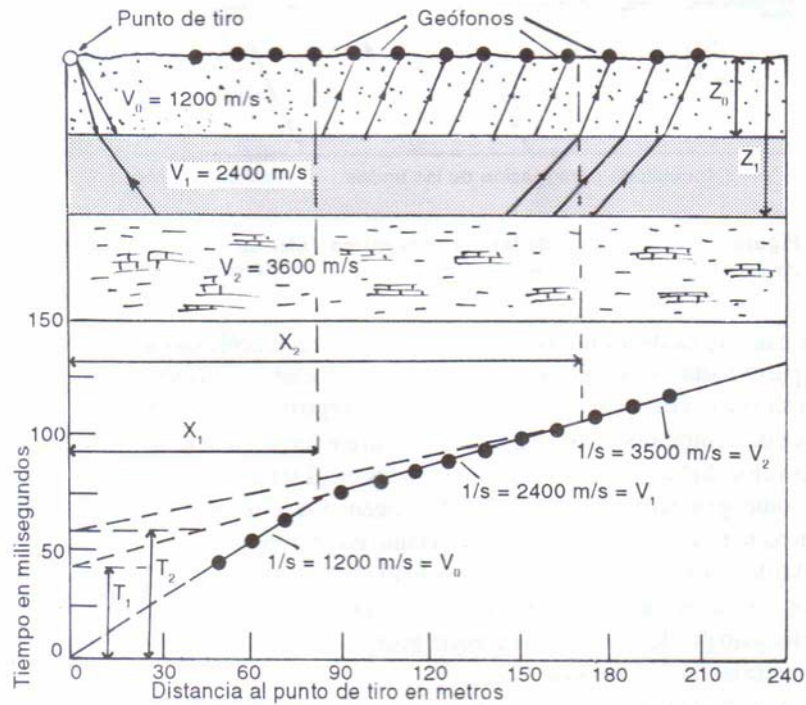
Figura 14. Dromocrónica de una Prueba Sísmica. Fuente: Ruiz, 2000.
