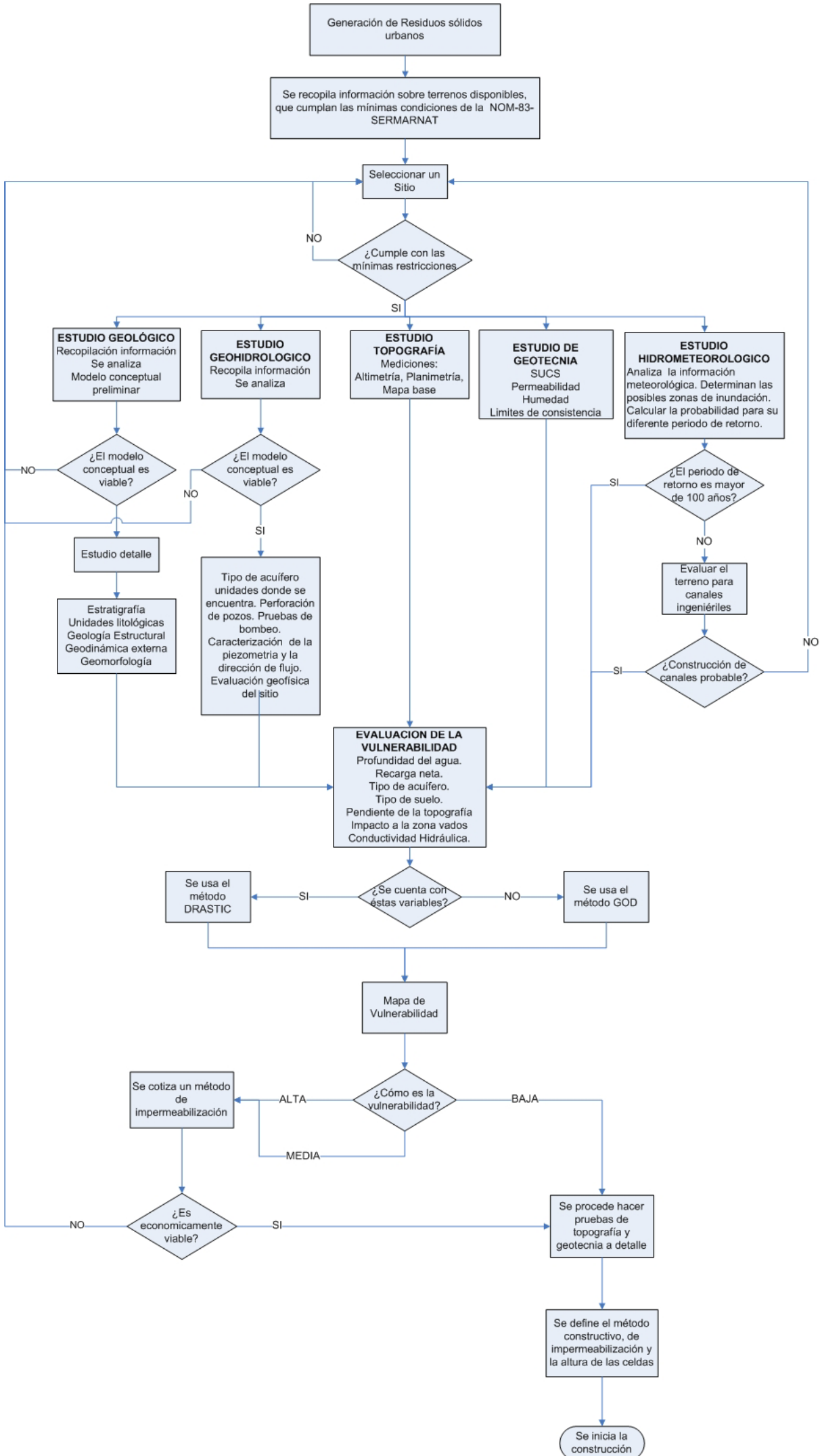
Figura 14a. Diagrama de flujo para la selección de un sitio de relleno sanitario
