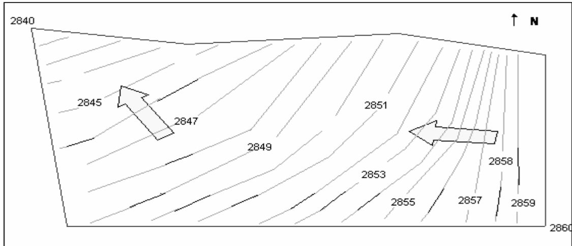
Figura 11. Configuración del flujo subterráneo en el terreno del Relleno Sanitario.
