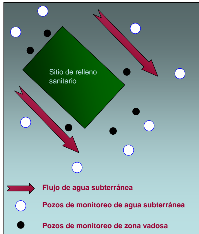
Figura 17. Ejemplo de un programa de monitoreo, vista de planta.
