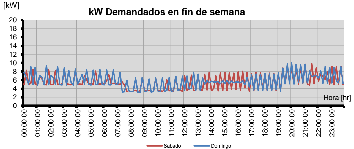
Gráfica 6. Gráfica de demanda en fin de semana del 9 al 16 de octubre de 2014 LEMA.
