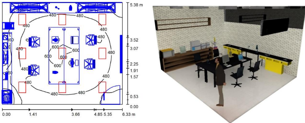
Figura 9 Vista general de laboratorios, Edificio LEMA, Instituto de Física
