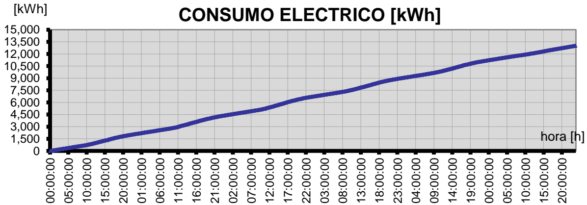
Grafica 4. Grafica de consumo eléctrico acumulado del 17 al 24 de septiembre de 2014 Colisur.
