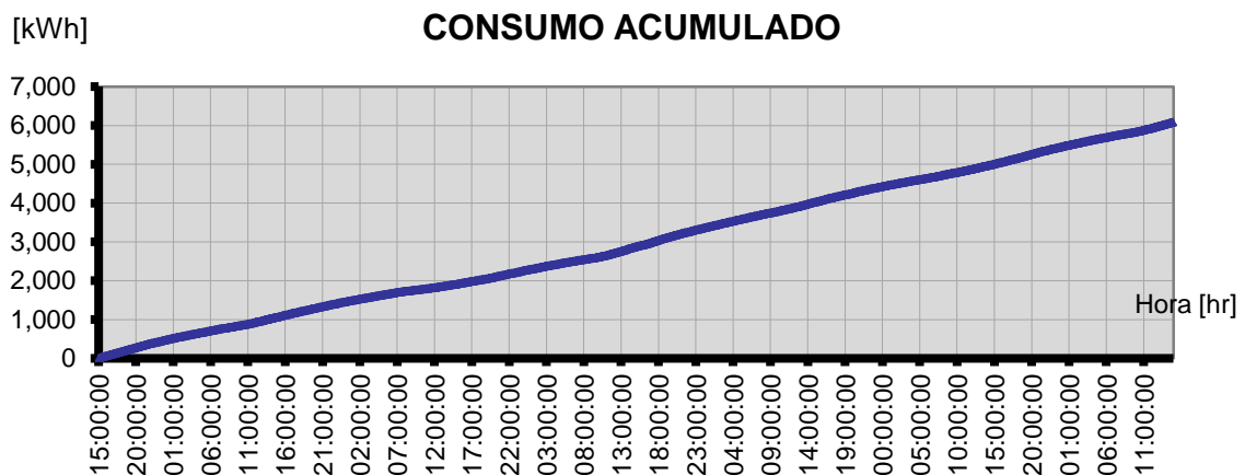
Gráfica 7. Gráfica de consumo eléctrico acumulado del 9 al 16 de octubre de 2014 LEMA
