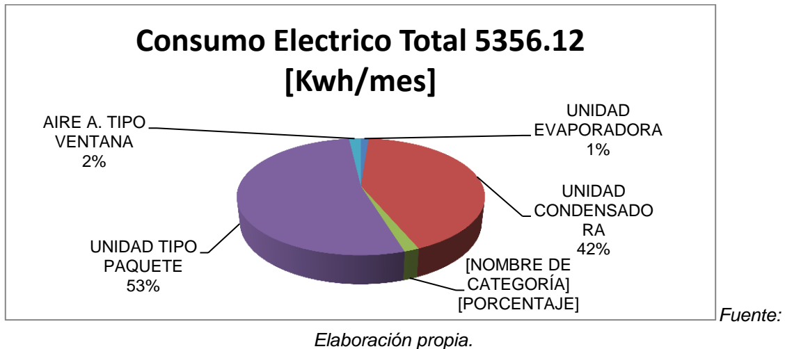
Grafica 14. Consumo Eléctrico Mensual de Equipos de Aire Acondicionado.
