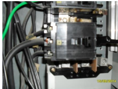
Imagen 2.16 Interruptor principal
