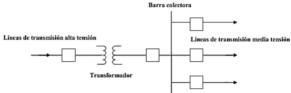
Imagen 1.10 Subestación reductora.
