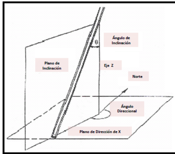
Fig. 4.5 Planos de inclinación en un pozo direccional (Cárdenas, 2008)
