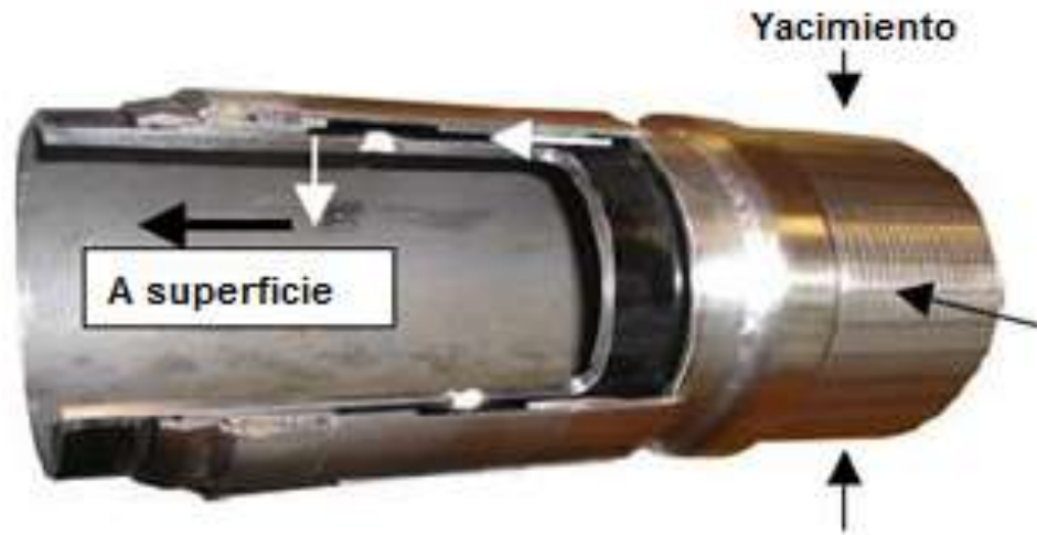
Figura 6.4 ICD tipo boquilla
