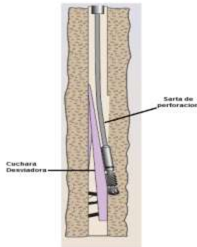
Figura 2.6 Cuchara desviadora en agujero descubierto
