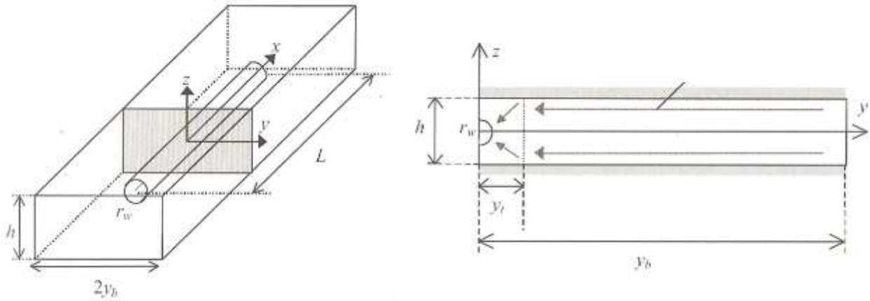
Figura 4.3 Geometría del flujo del modelo de Furui
