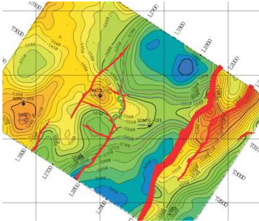
Figura 5.8 Modelo Estructural
