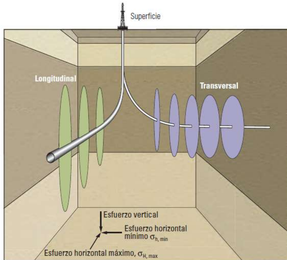
Figura 4.12 Fracturas longitudinales y transversales
