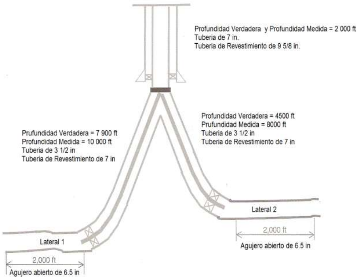
Figura 7.1 Pozo multilateral
