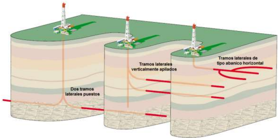
Figura 2.15 Configuraciones básicas de un pozo multilateral
