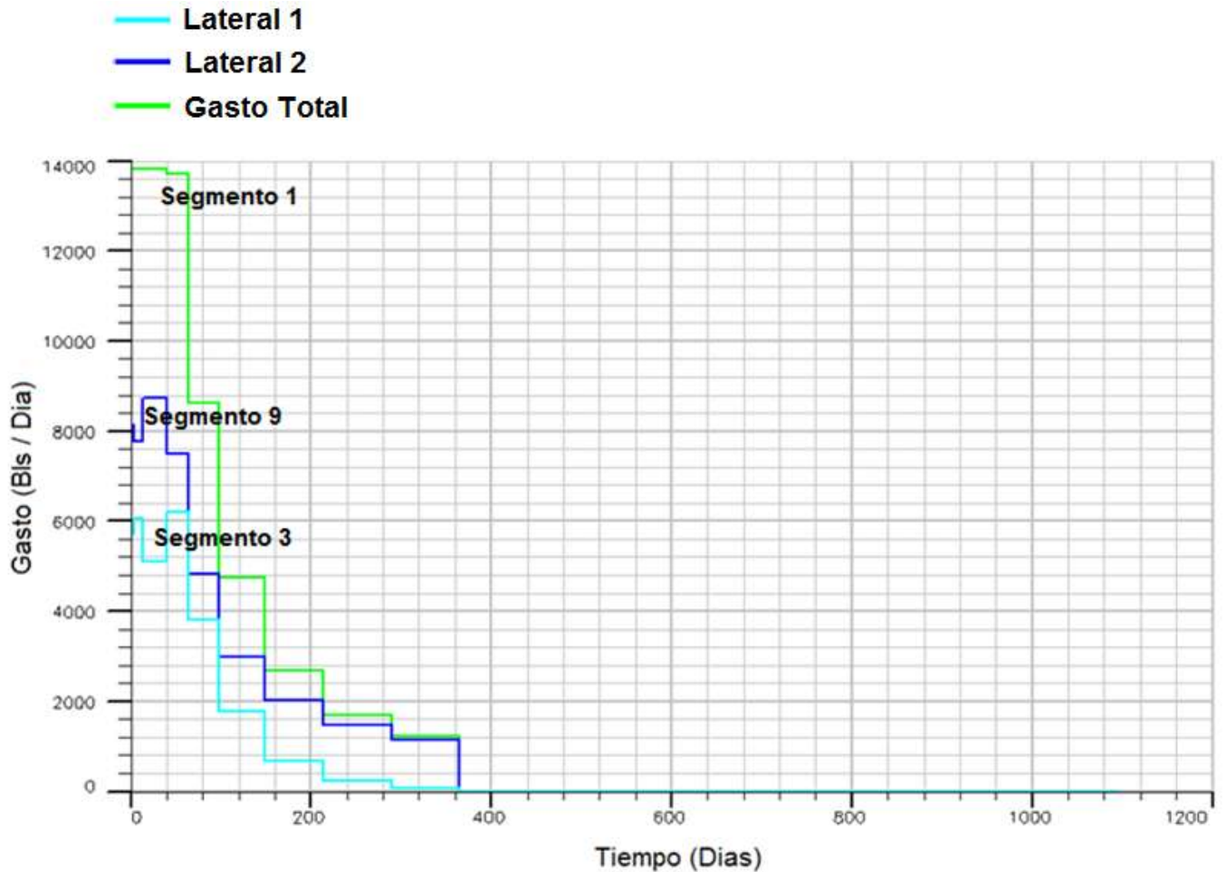
Figura 7.23 Gastos del pozo multilateral caso 1
