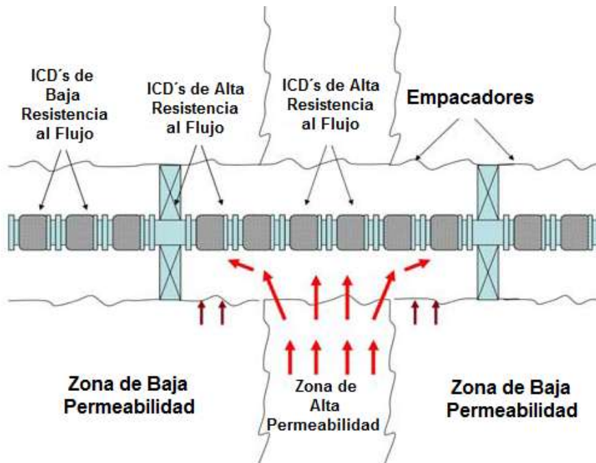
Figura 6.12 La zona de alta permeabilidad limita la contribución de flujo de las zonas de baja permeabilidad
