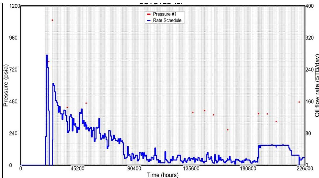
Figura 5.11 Historia de Presión Producción del Pozo C-3 (CNH/UNAM, 2012).
