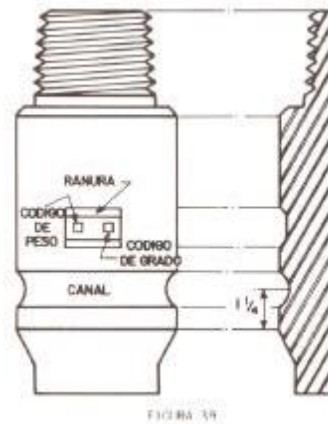
Fig. 3. 11 Si el piñón tiene la acanaladura en la base y la ranura en el centro, se tratará de una tubería de alto peso y alta resistencia.
