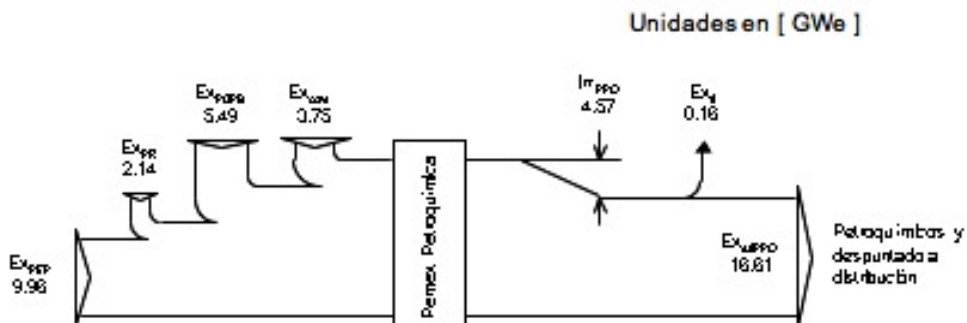
Figura 6.4 Balance de exergía para Pemex Petroquímica (PPQ).
