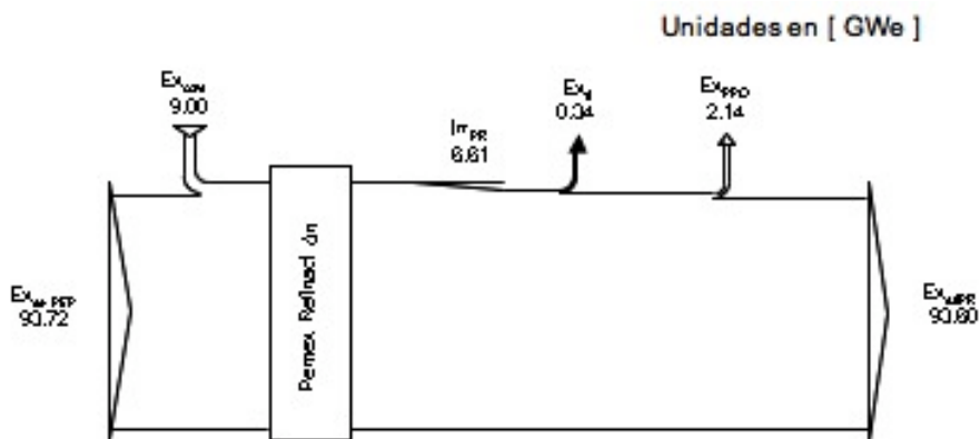
Figura 6.2 Balance de exergia para Pemex Refinación (PR).
