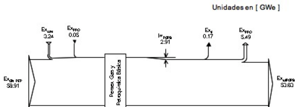
Figura 6.3 Balance de exergia para Pemex Gas y Petroquímica Básica (PGPB).
