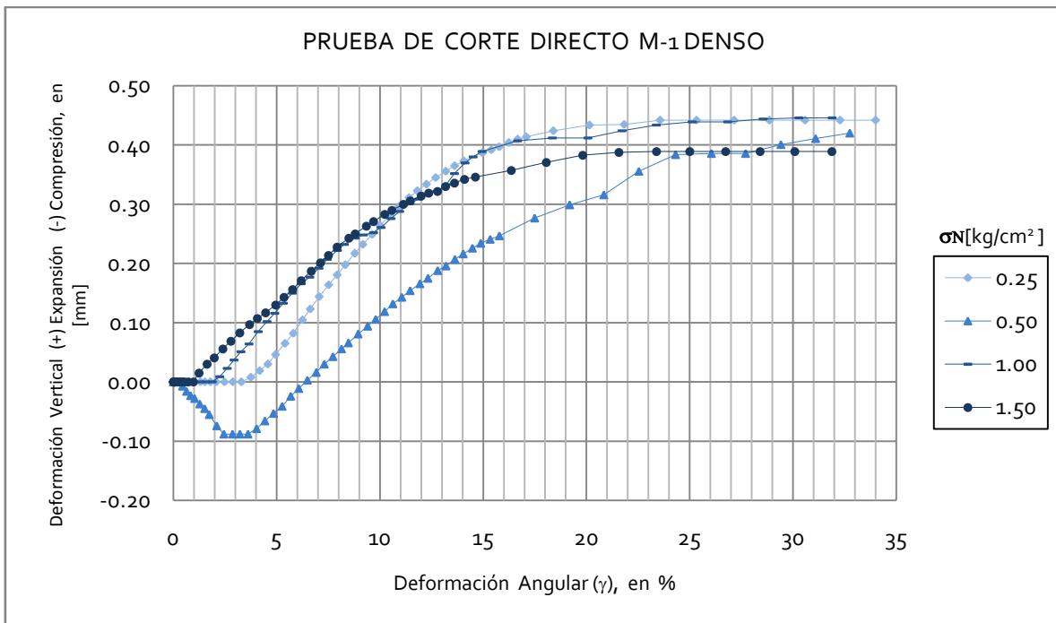
Figura 6.4 Curva Deformación Angular, Deformación Vertical (Expansión y Compresión) de la muestra M-1 Estado Denso
