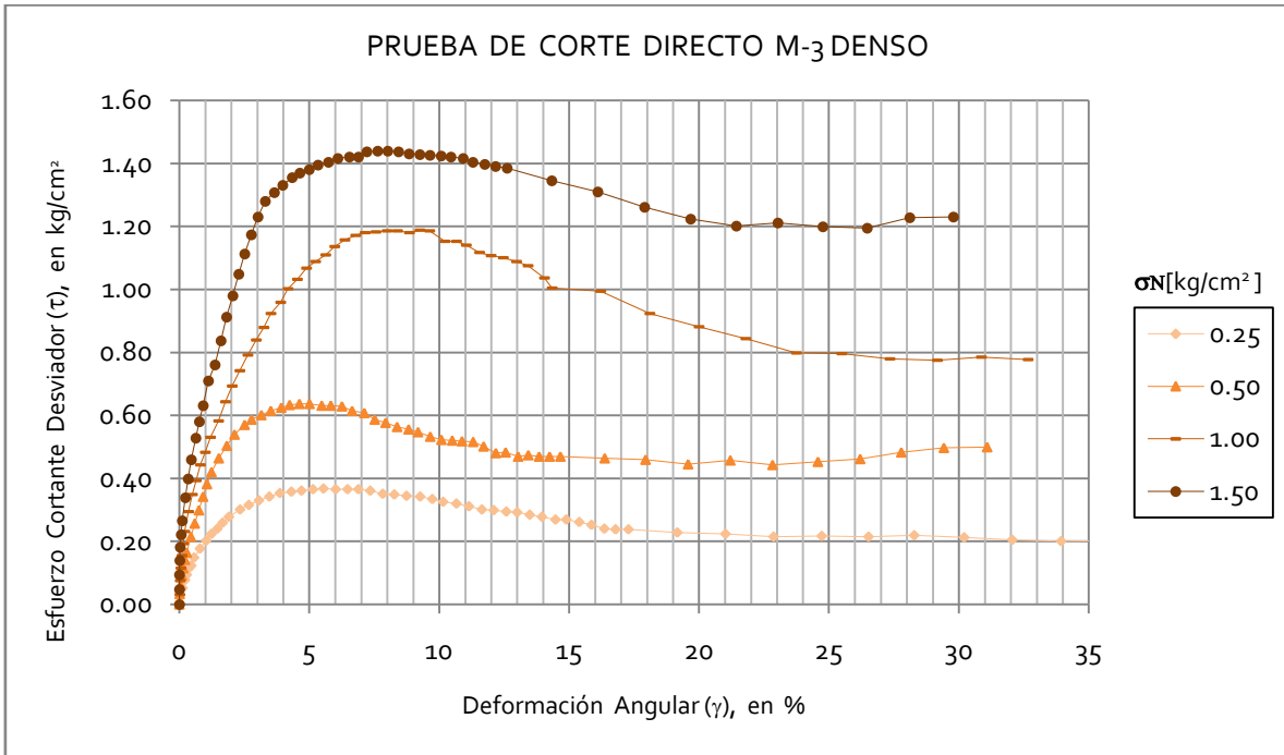
Figura 6.11 Curva de la Muestra M-3 Deformación Angular ( \gamma ) en porcentaje, contra Esfuerzo Cortante Desviador ( \tau ), en [ \text{kg/cm}^2 ].
