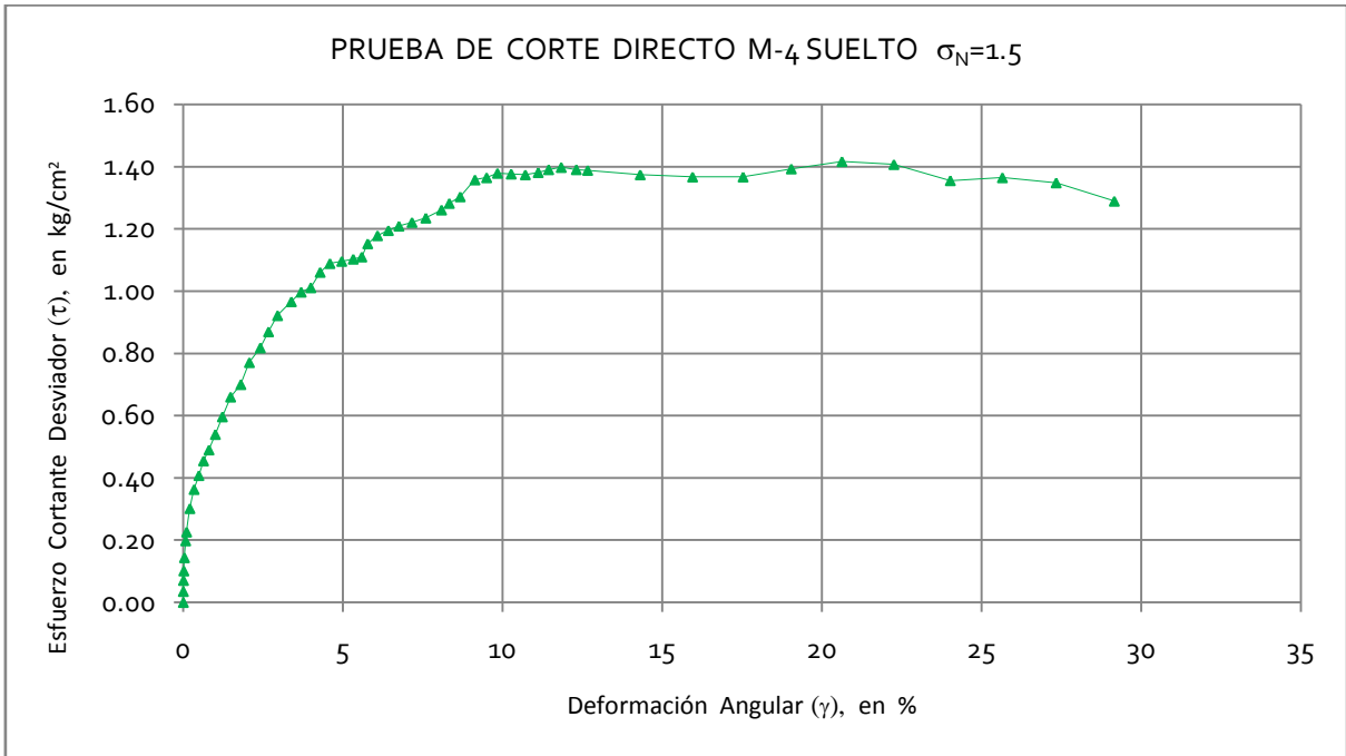
Figura 5.55 Curva Deformación Angular, Esfuerzo Cortante Desviador de la M-4 Estado Suelto \sigma_N=1.5
