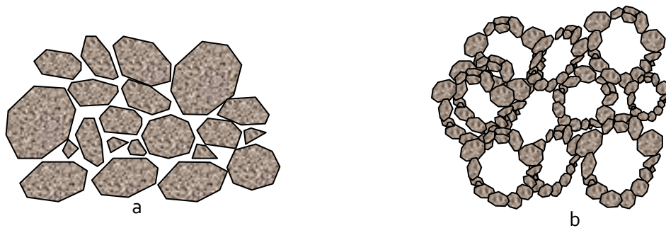
Figura 1.5 Forma de reacomodo de las partículas del suelo (Das, 1998). (a) Densa. (b) Suelta.
