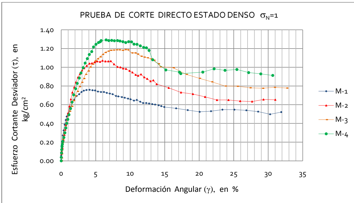
Figura 6.25 Curvas de todas las muestras, Deformación Angular ( \gamma ) en porcentaje, contra Esfuerzo Cortante Desviador ( \tau ), en [ \text{kg/cm}^2 ]. Con \sigma_N=1 Estado Denso
