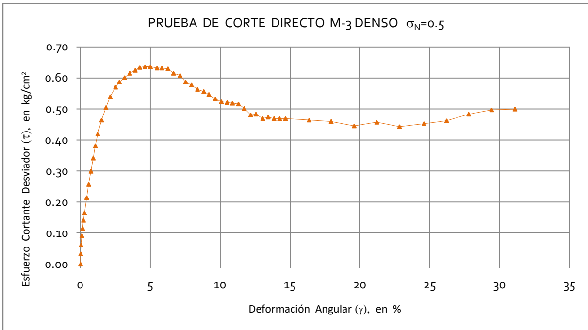
Figura 5.43 Curva Deformación Angular, Esfuerzo Cortante Desviador de la M-3 Estado Denso \sigma_N=0.5
