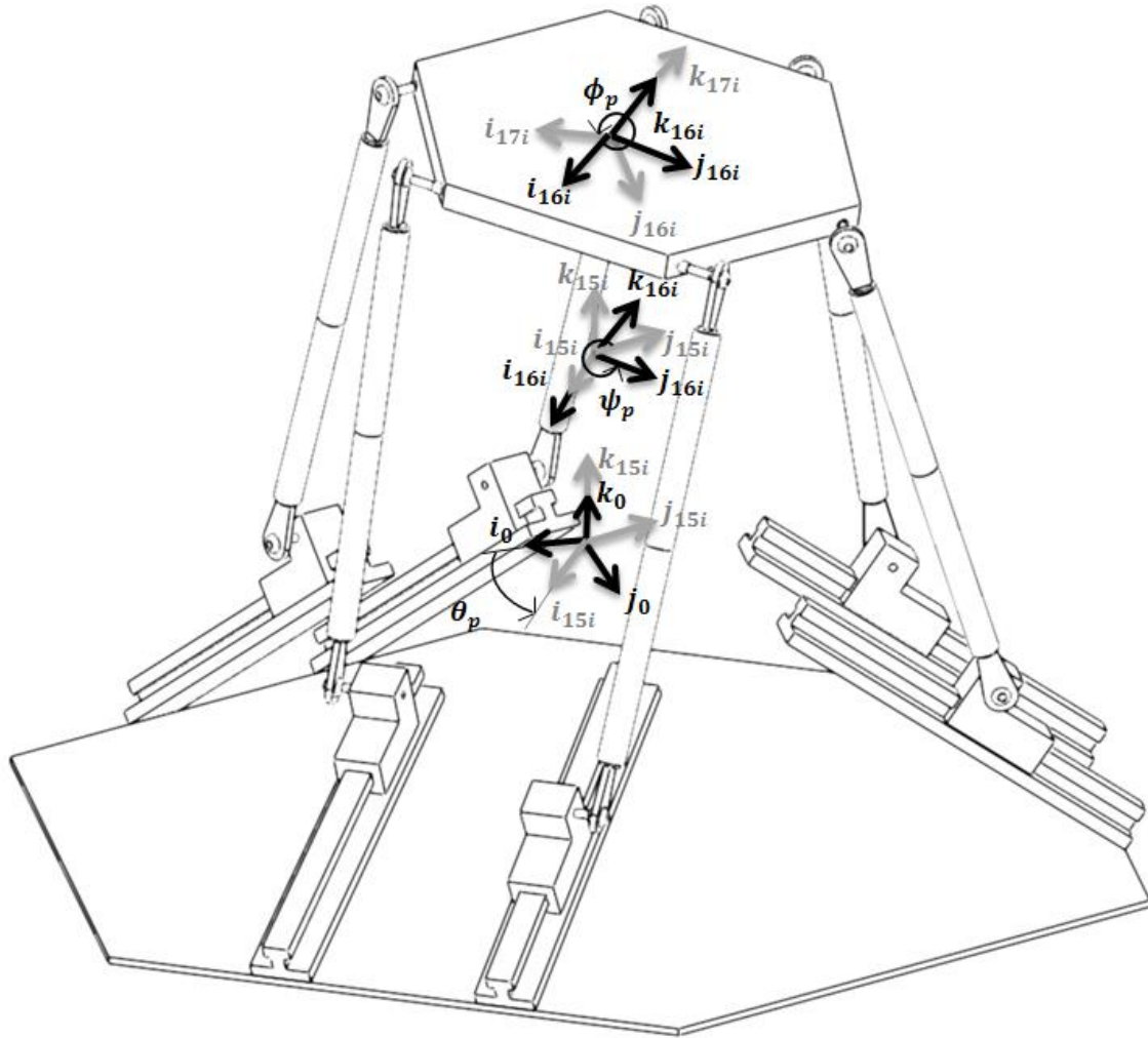
Fig. 2.7 Ángulos de Euler
