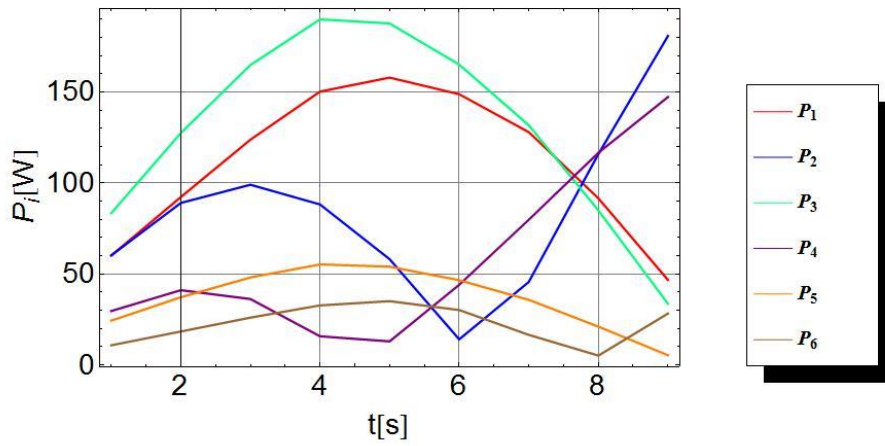
Fig. 4.21 Gráfica de potencia necesaria en los actuadores
