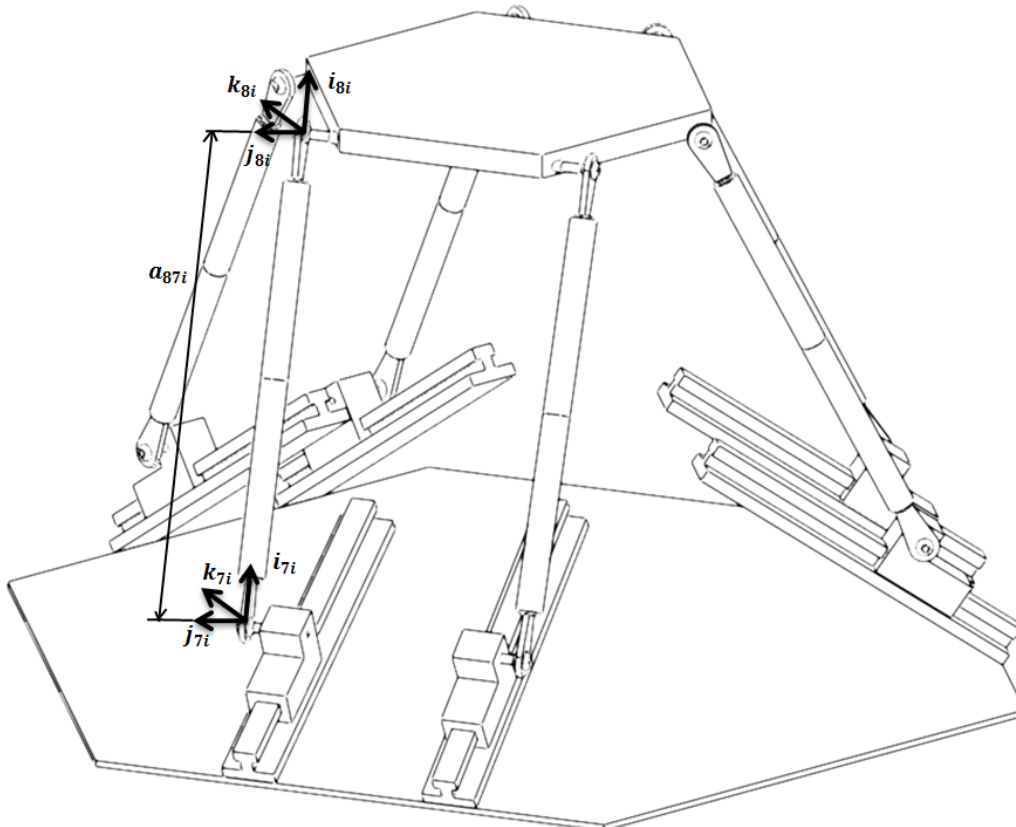
Fig. 2.4 Sistemas de referencia del 7i al 8i
