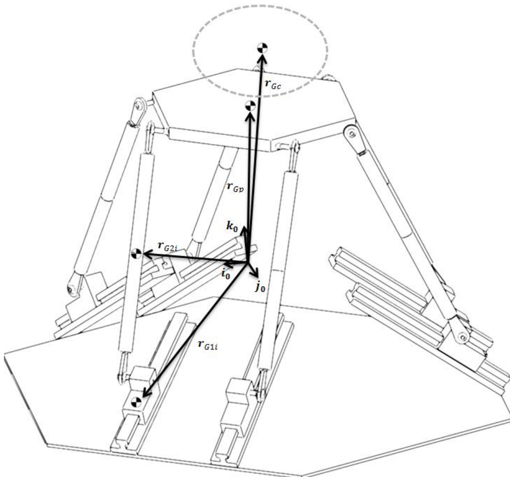
Fig. 3.2 Vectores de centro de gravedad
