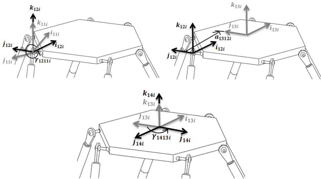
Fig. 2.6 Sistemas de referencia del 11i al 14i
