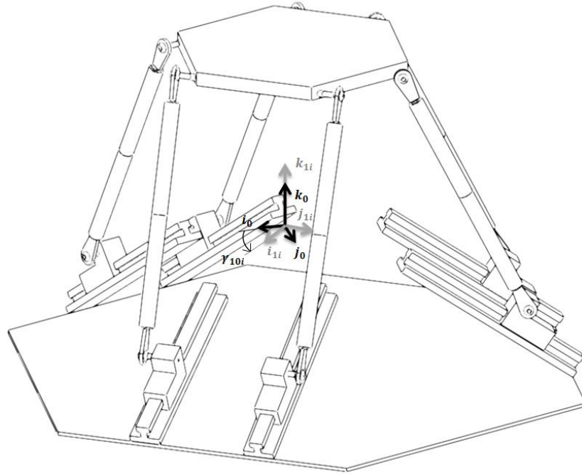
Fig. 2.1 Sistemas de referencia del inercial al 1i
