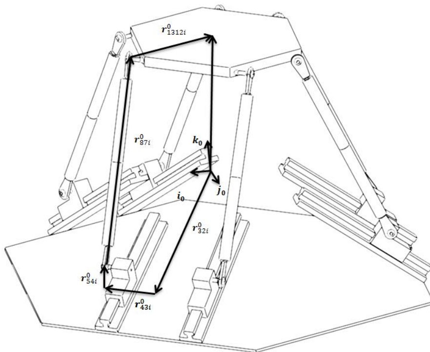
Fig. D.1 Ecuación de Lazo
