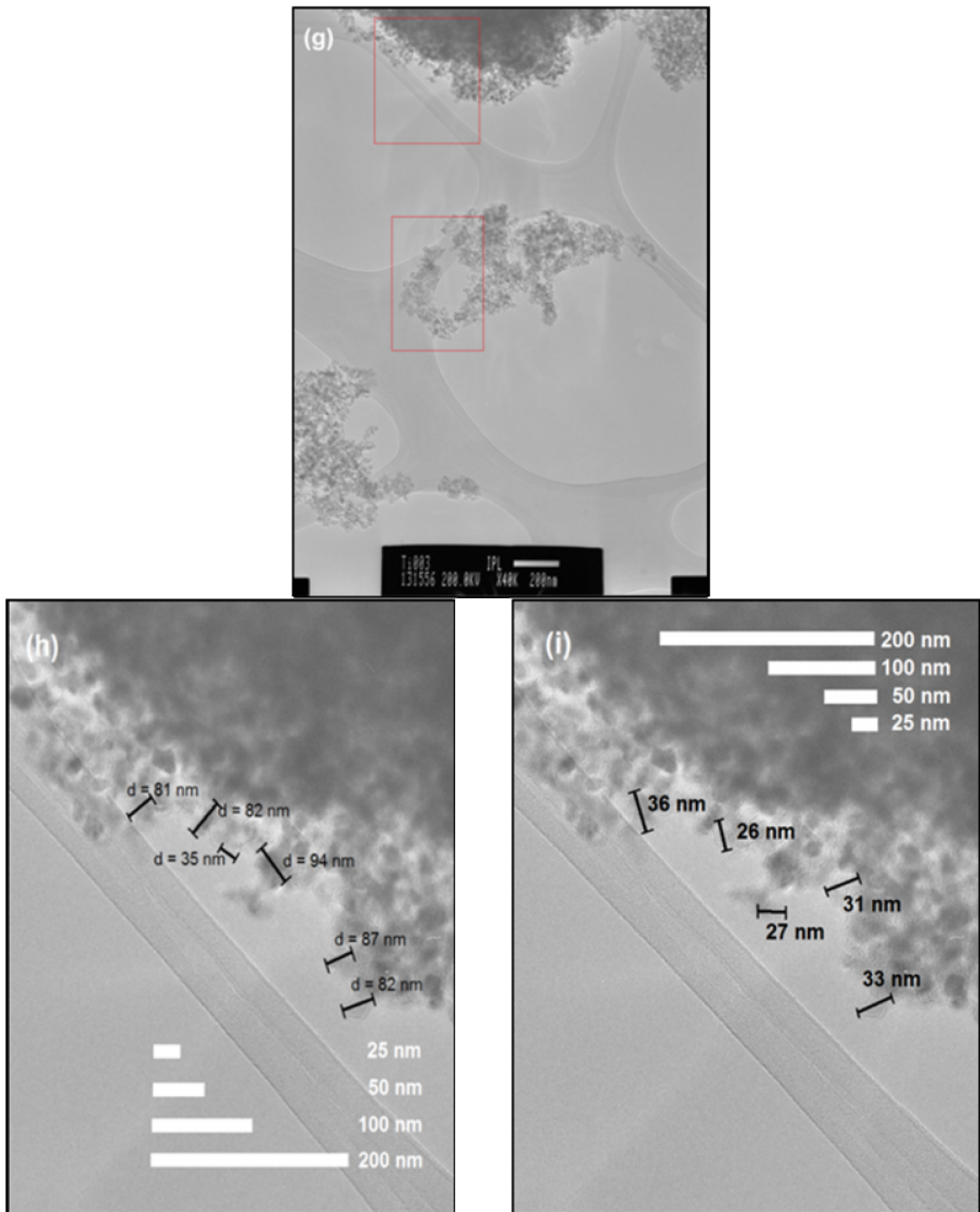
Figura 4.1. g) imagen arriba, micrografía TiO 2 con una resolución de 200 nm, h) imagen izquierda abajo, ampliación de la primera imagen, con tamaños de cristal entre los 31 a 81 nm, i) imagen derecha abajo, ampliación de la primera imagen, entre los 27 a 36 nm
