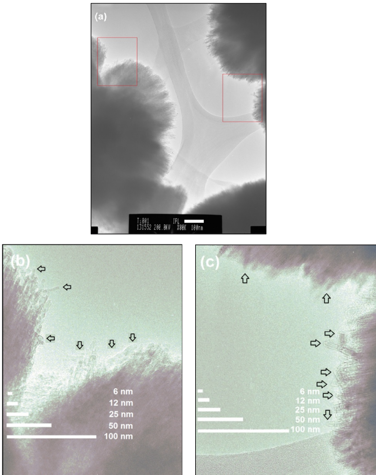
Figura 4.1. a) imagen arriba, micrografía Ti001 con una resolución de 100 nm, b) imagen izquierda abajo, ampliación de la primera imagen donde se observan estructuras filamentosas señaladas con flechas, c) imagen derecha abajo ampliación de la primera imagen se observan otras estructuras filamentosas aglomeradas de entre 5-6 nm de diámetro
