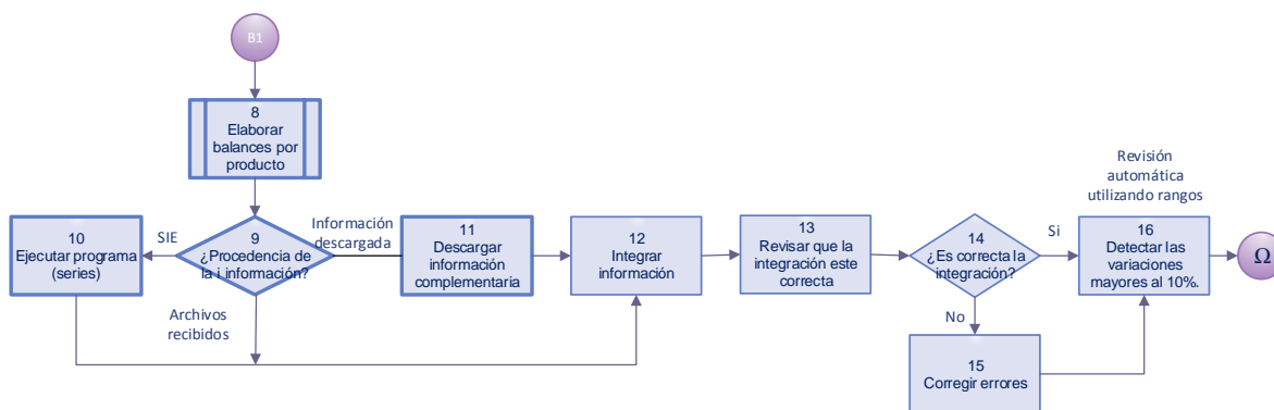
Figura 3. 26 Diagrama de flujo de balances por producto (parte 1). Fuente: Elaboración propia.
