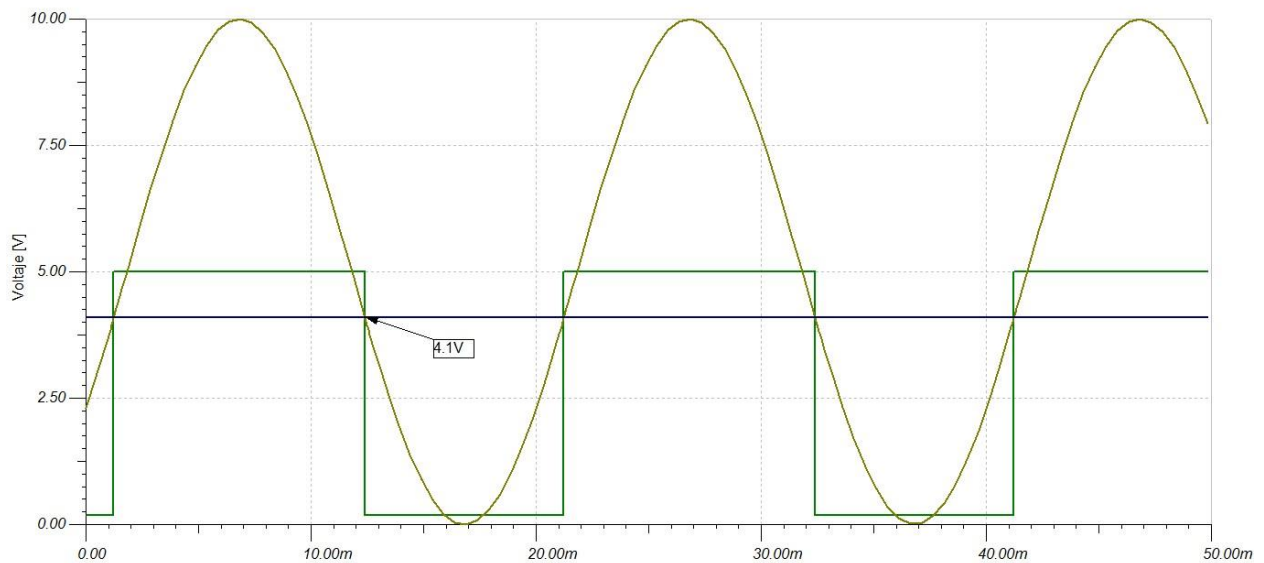
Figura 4.17. Simulación del comparador de voltaje.
