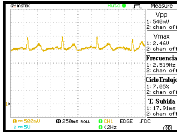
Figura 5.1. Señal ECG: salida de la tarjeta de adquisición luego de filtro pasa bajas y filtro Notch.
