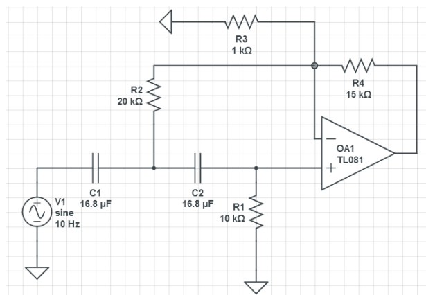
Figura 4.12. Circuito esquemático del filtro pasa altas con respuesta Butterworth y topología Sallen Key.
