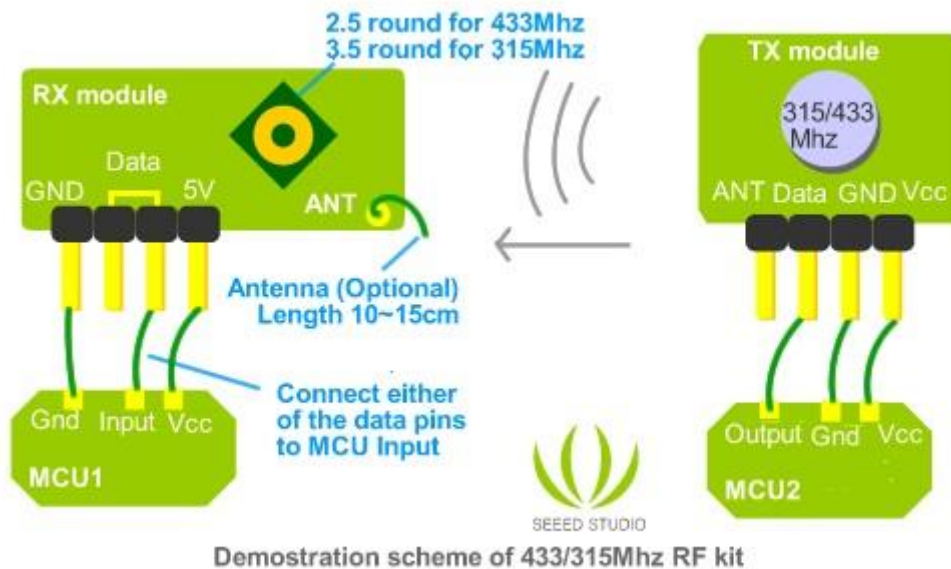
Figura 4.29. Demostración para la conexión de los módulos RF de 433MHz con dos micro-controladores [65].
