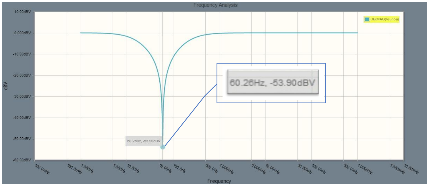
Figura 4.11. Respuesta en frecuencia del filtro supresor de banda con frecuencia de corte de 60Hz.
