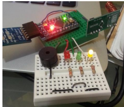
Figura 5.16. Demostración de la alarma para la arritmia bradicardia, led color amarillo.
