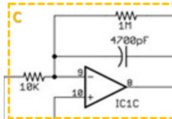
Figura 4.6. Sub-circuito para el filtro pasa bajas.
