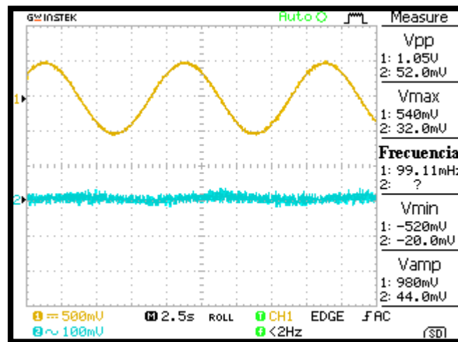
Figura 5.2. Comprobación del filtro pasa altas y señal de entrada de 0.1Hz y 1V (canal 1, señal amarilla).
