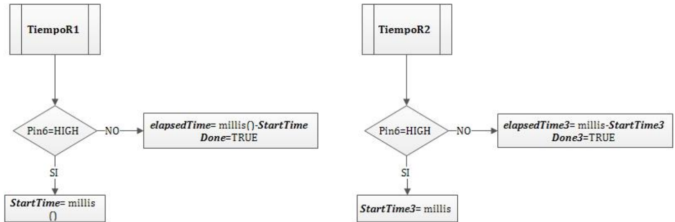
Figura 4.21. Diagrama de flujo para las subrutinas TiempoR1 y TiempoR2 .
