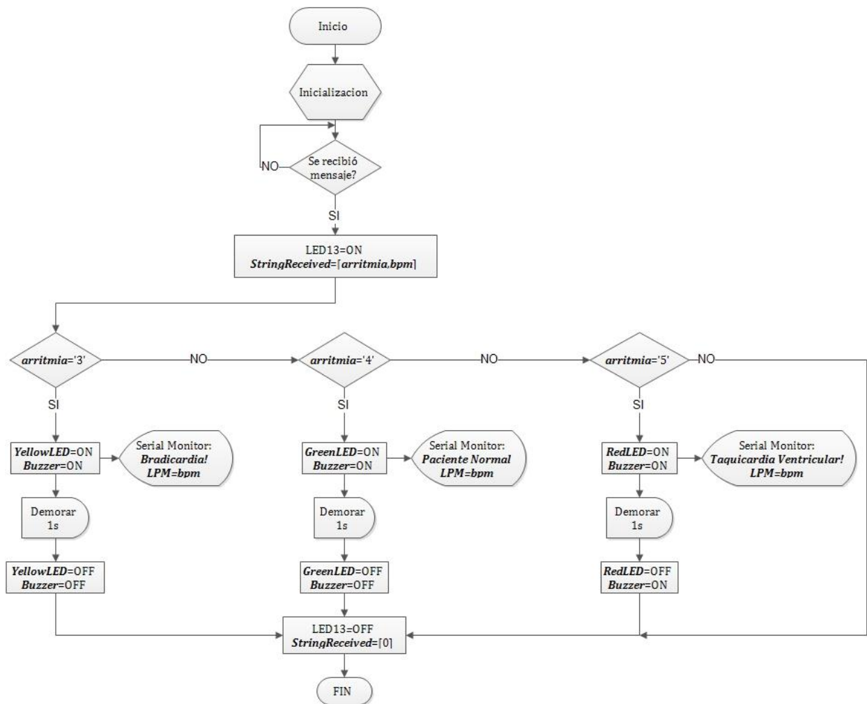
Figura 4.35. Diagrama de flujo del algoritmo para la decodificación de alarma.
