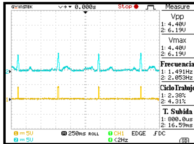
Figura 5.7. Detección de los picos R en la señal de ECG: la señal amarilla (canal 1) es la entrada al detector de picos y la señal azul es la salida de la etapa de adquisición y filtrado (canal 2).
