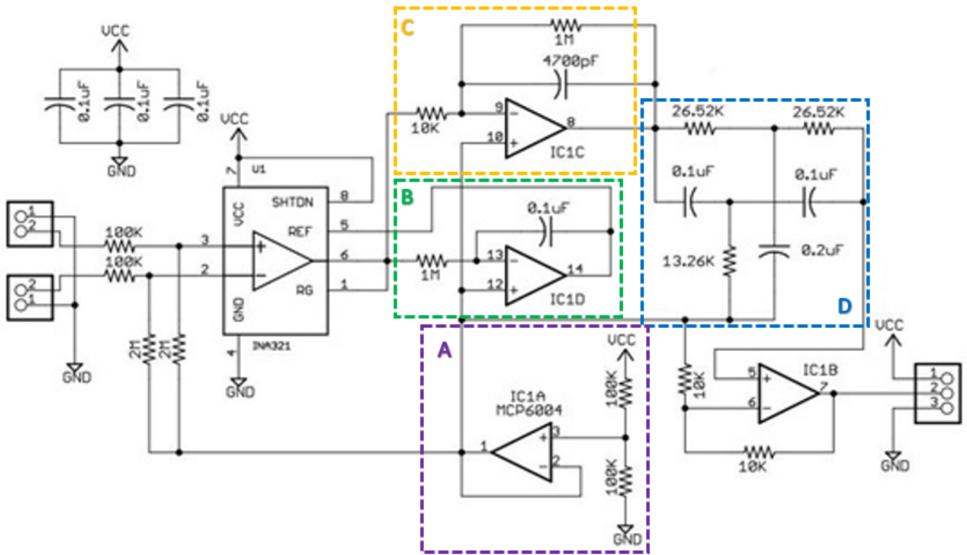
Figura 4.3. Circuito esquemático de la tarjeta de adquisición [60].
