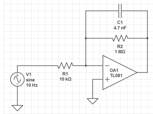
Figura 4.7. Circuito esquemático de filtro pasa bajas simulado.
