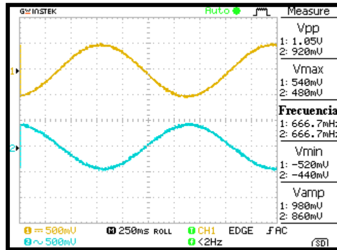
Figura 5.3. Comprobación del filtro pasa altas y señal de entrada de 0.6Hz y 1V (canal 1, señal amarilla).
