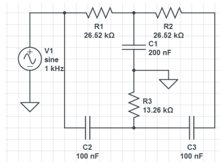
Figura 4.10. Circuito esquemático de filtro supresor de banda con simulado.
