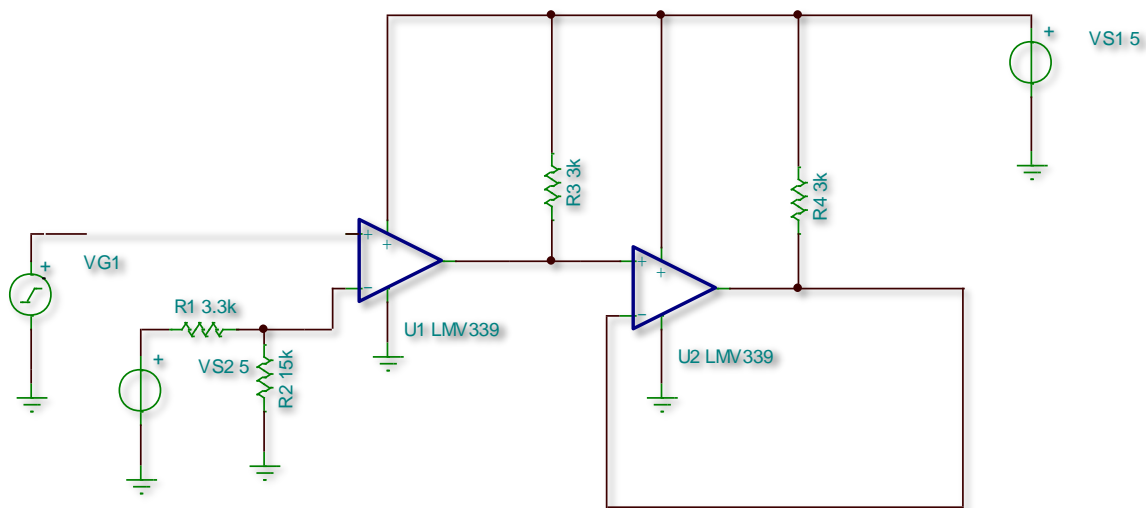
Figura 4.16. Circuito esquemático para detectar máximos.
