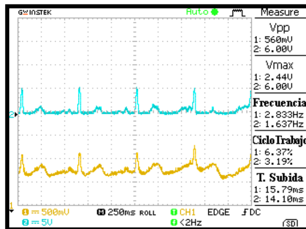
Figura 5.6. Señal ECG: comparación de la salida de la tarjeta de adquisición (canal 1, señal amarilla) y salida del filtro 0.67hz (canal 2, señal azul).
