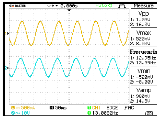
Figura 5.4. Comprobación del filtro pasa altas y señal de entrada de 13 Hz y 1V (canal 1, señal amarilla).
