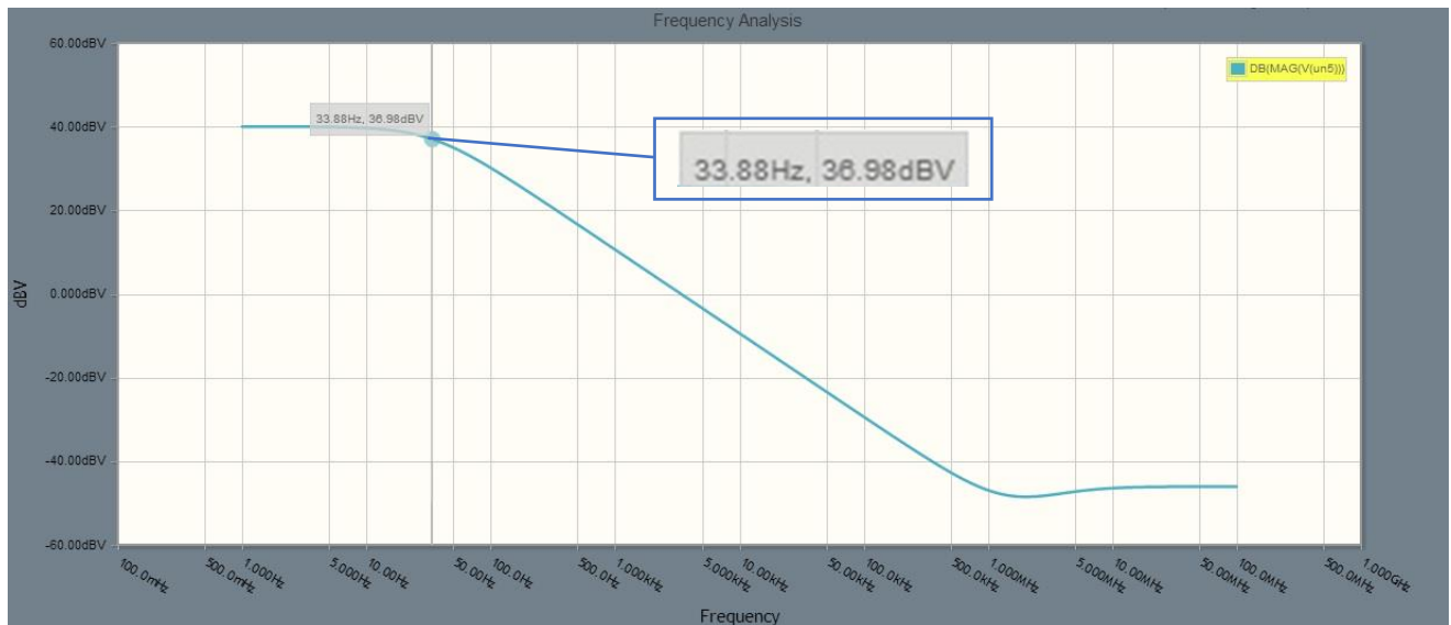
Figura 4.8. Respuesta en frecuencia del filtro pasa bajas con frecuencia de corte de 33.86Hz.
