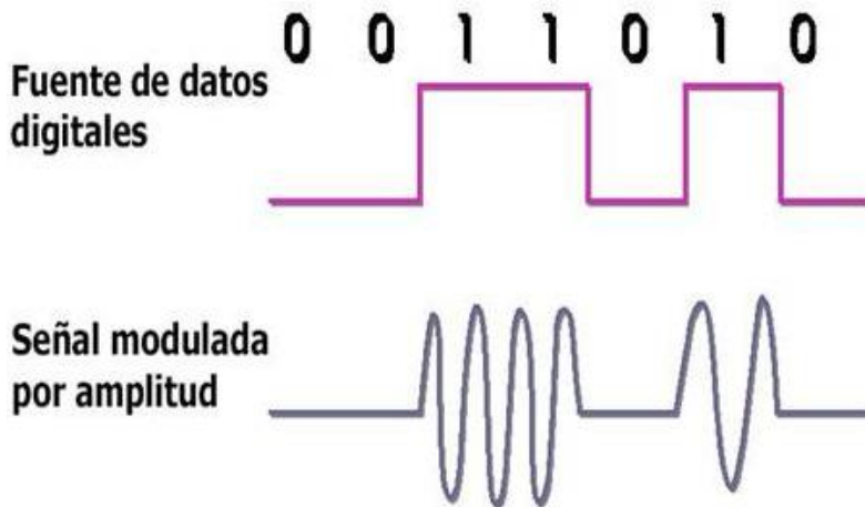
Figura 4.31. Ejemplo de una modulación por desplazamiento de amplitud (ASK) [69].
