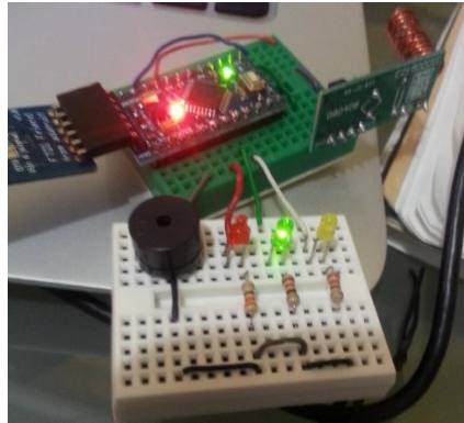
Figura 5.18. Demostración de la alarma para la arritmia bradicardia, led color verde.
