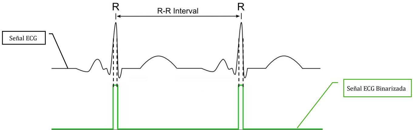
Figura 4.15. Representación de la señal de ECG, intervalo R-R y su respectiva señal binarizada.
