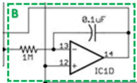
Figura 4.5. Sub-circuito para el ajuste del voltaje de desplazamiento.
