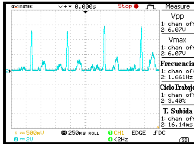
Figura 5.5. Señal ECG: luego del filtro pasa altas de 0.67Hz y amplificación.
