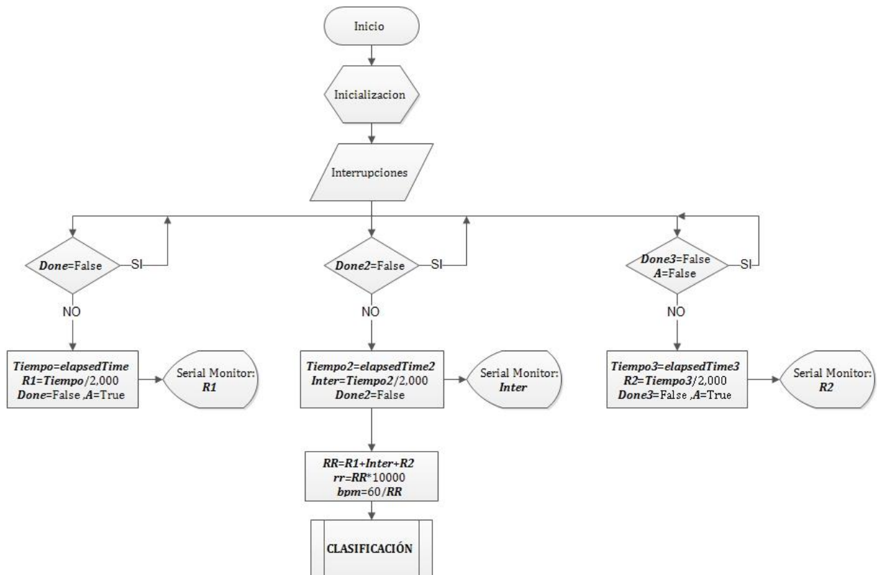
Figura 4.24. Diagrama de flujo para el lazo en el cual se calcula la duración del intervalo RR.
