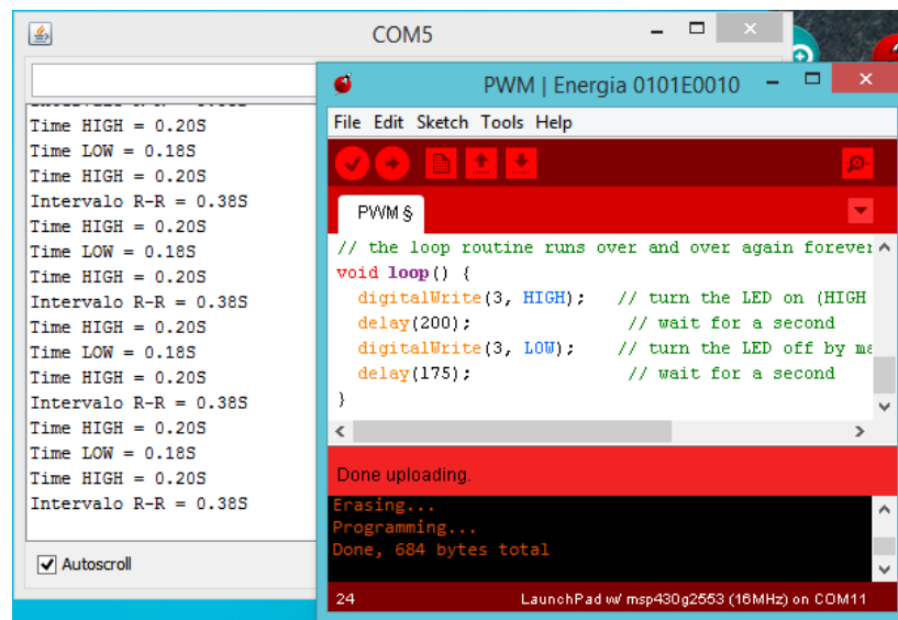
Figura 5.10. Detección de la señal PWM para un intervalo de 0.375 s.
