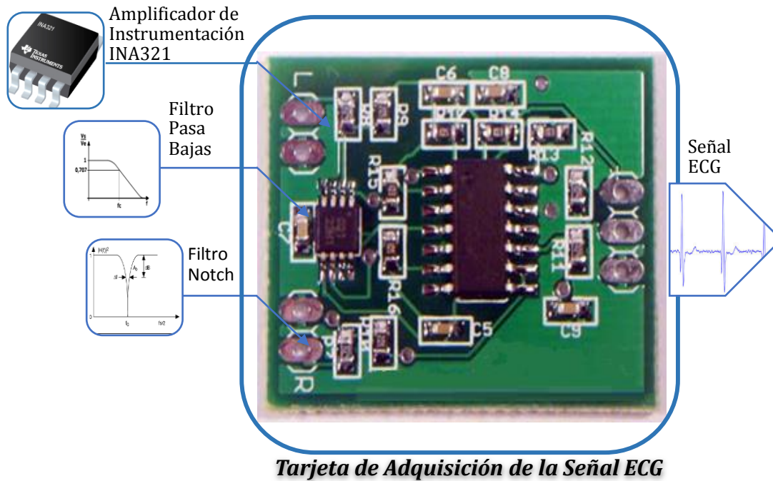
Figura 4.2. Tarjeta de adquisición basada en el amplificador de instrumentación INA321 con filtro pasa bajas a 34Hz y filtro Notch de 60 HZ.
