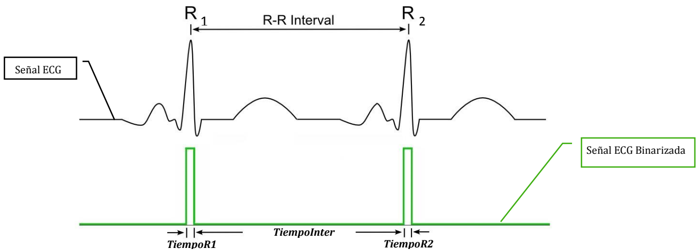
Figura 4.23. Representación de la medición de los intervalos para las subrutinas TiempoR1 , TiempoInter y TiempoR2 .
