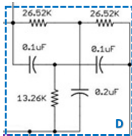
Figura 4.9. Sub-circuito del filtro supresor de banda (Notch).
