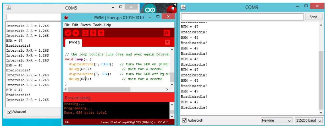
Figura 5.15. Detección de la arritmia bradicardia, con un intervalo de 1.26 s y BPM igual a 47.
