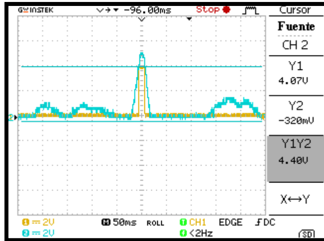
Figura 5.8. Voltaje de referencia para el comparador de voltaje.
