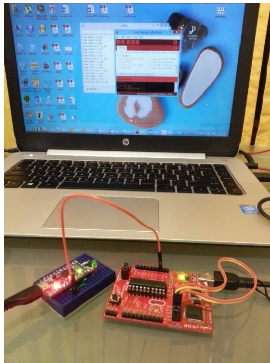
Figura 5.9. Tarjeta de desarrollo Arduino Pro-Micro, detector del intervalo RR y tarjeta de desarrollo para el micro-controlador MSP432553, simulador de la señal PWM.
