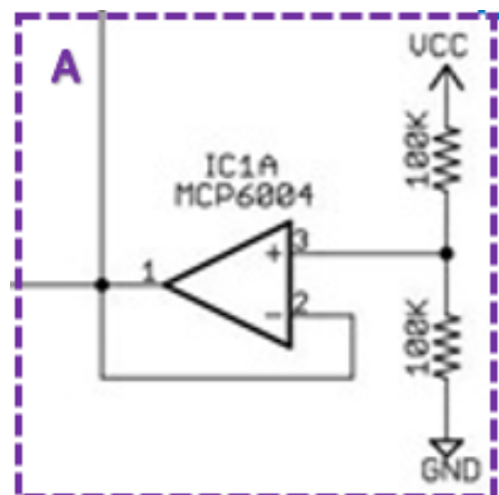
Figura 4.4. Sub-circuito para voltaje de referencia.
