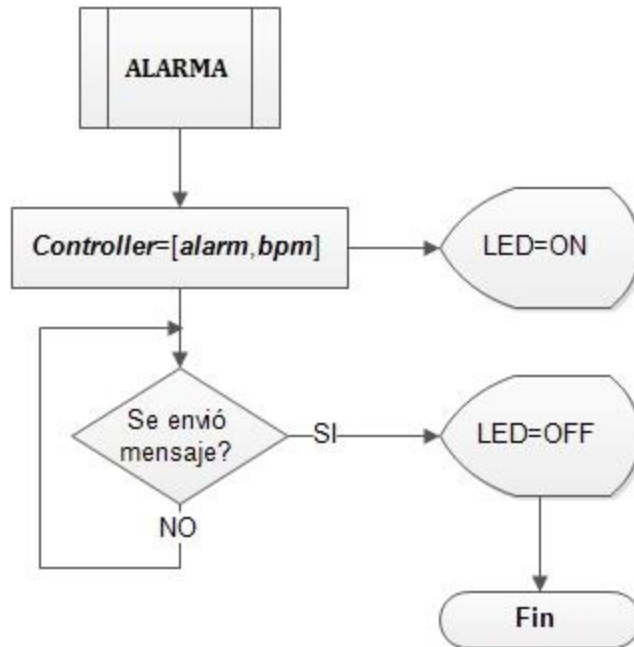
Figura 4.27. Diagrama de flujo de la subrutina Alarma .
