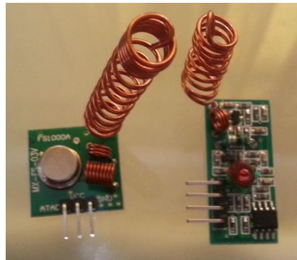
Figura 4.30. Módulos de RF con sus respectivas antenas.
