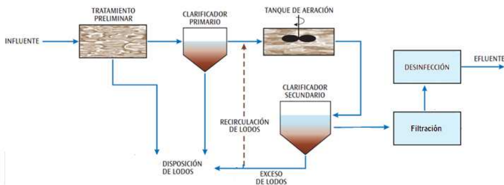
Figura 8- Componentes de un sistema de lodos activados con tratamiento de lodos 36
