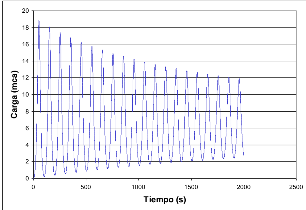
Figura 5.7. Sobrepresión alcanzada en el emisor a la altura de la falla con X = 1900 m, L_{Bolsa\ de\ aire} = 50 m.
