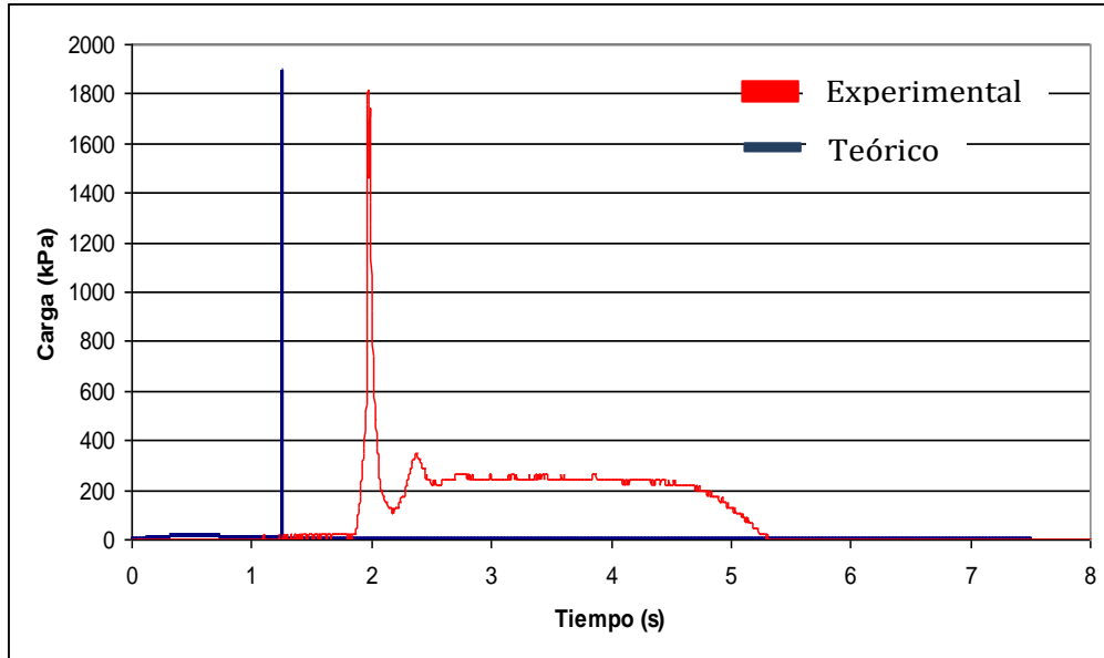
Figura 4.18. Patrón tipo 3, d_o = 16 mm, H_0 = 275 kPa, x = 2.2 m.
