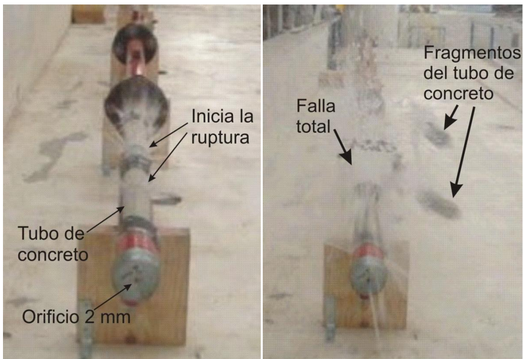
Figura 4.28. Izquierda: inicia la ruptura y fuga de agua para H_0 = 68.95 \text{ kPa} ó 7 \text{ mca} , d_0 = 2 \text{ mm} y x = 2.2 \text{ m} . Derecha: falla total del tubo de concreto.
