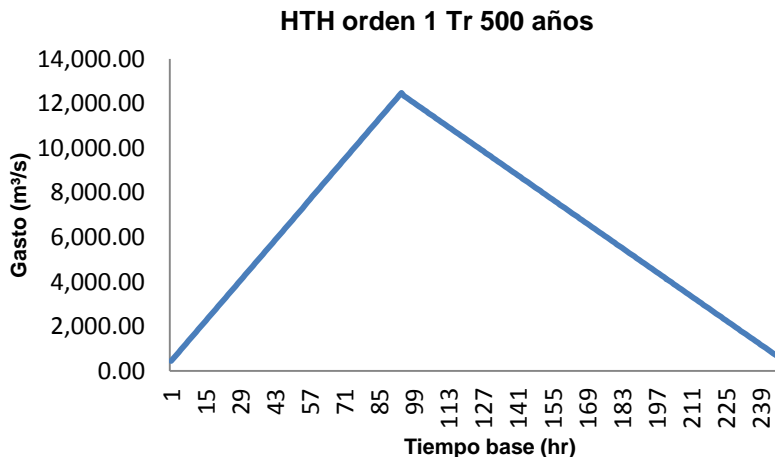
Ilustración 5.21. Hidrograma Triparamétrico Hermitiano de orden 1° para un Tr de 500 años
