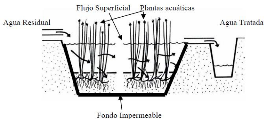
Figura 2. Sistema de flujo superficial. Fuente: (Mena-Sanz, 2008)
