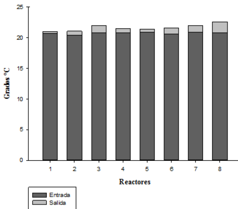
Figura 17. Temperatura en los 8 reactores experimentales
