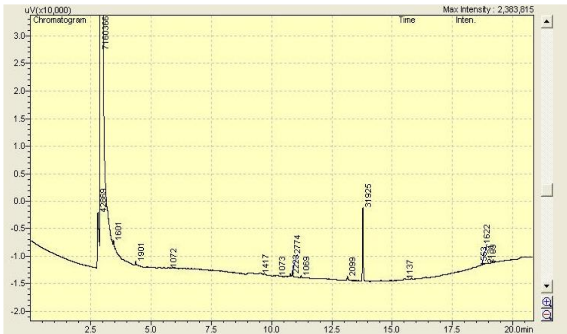
Figura 40. Cromatograma de reactor 6 (suelo), remoción de lindano.
