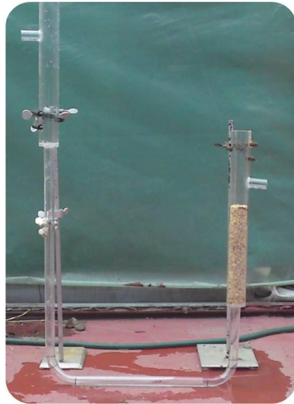
Figura 5. Permeámetro
