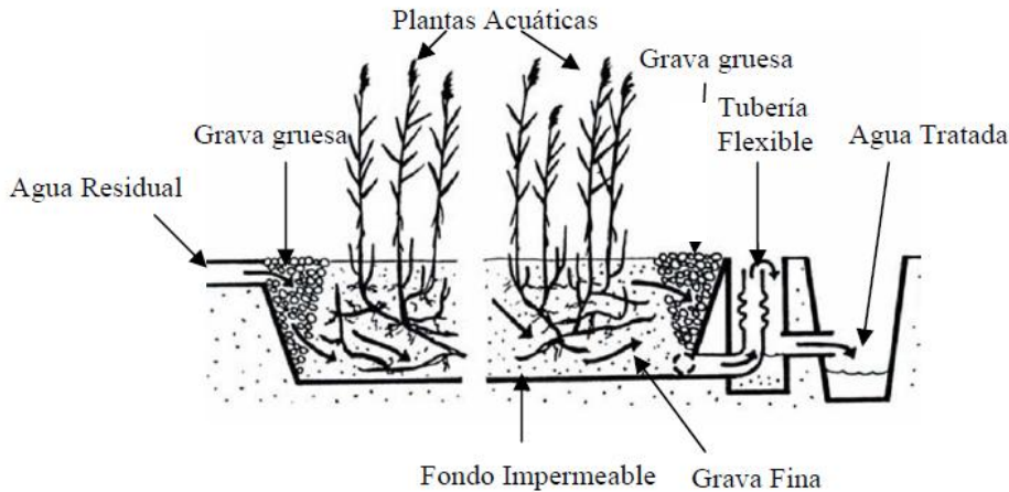
Figura 3. Sistemas de flujo subsuperficial horizontal. Fuente: (Mena-Sanz, 2008)
