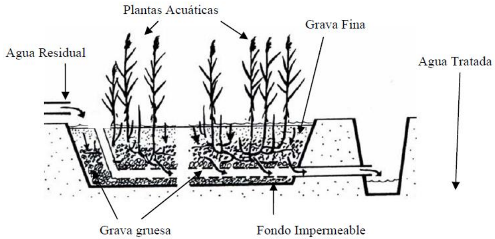
Figura 4. Sistemas de flujo subsuperficial vertical. Fuente: (Mena-Sanz, 2008)
