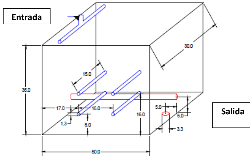
Figura 7. Dimensiones de los sistemas experimentales “HAFSSR” medida en (cm)
