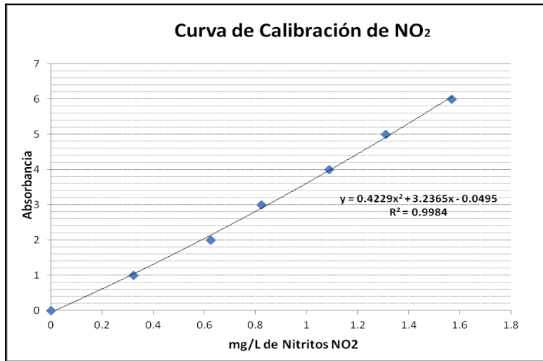
Figura 27. Curva de calibración Nitritos
