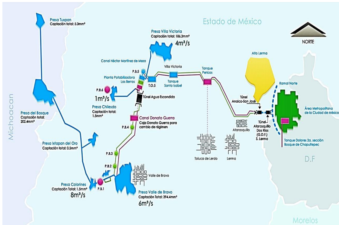
Figura 1 Croquis del Sistema Cutzamala (Fuente CONAGUA 2005 agua.org.mx)
