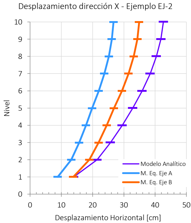
Figura IV-16 Gráficas de desplazamientos - Ejemplo EJ-2
