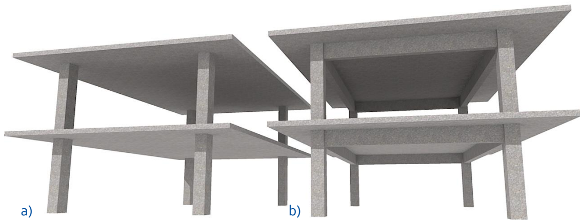
Figura I-6 Tipos de losas: a) Losa sin vigas, o plana b) Losa maciza soportada por vigas
