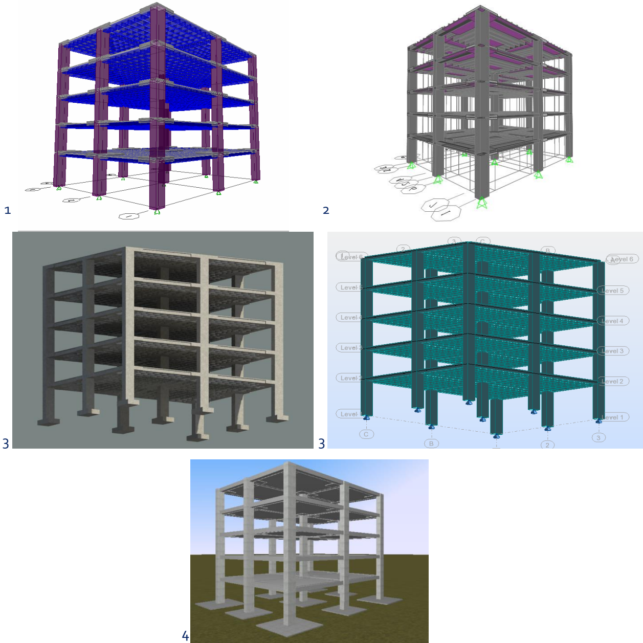
Figura III-3 Isométrico del modelo en los diferentes programas analizados.
