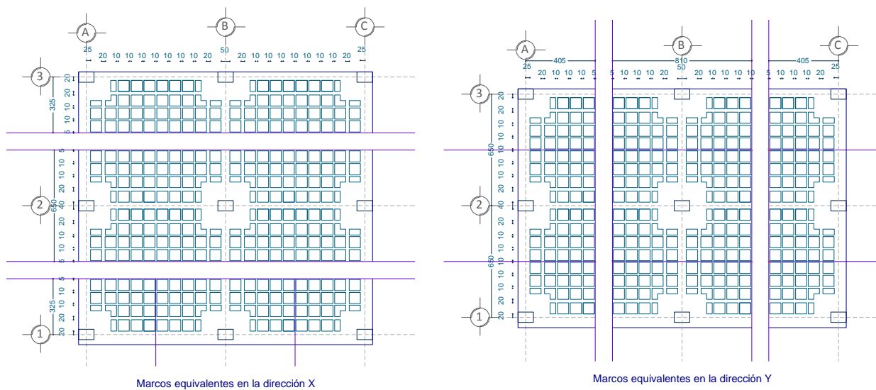
Figura III-8 Marcos equivalentes en las dos direcciones para el ejemplo E-1
