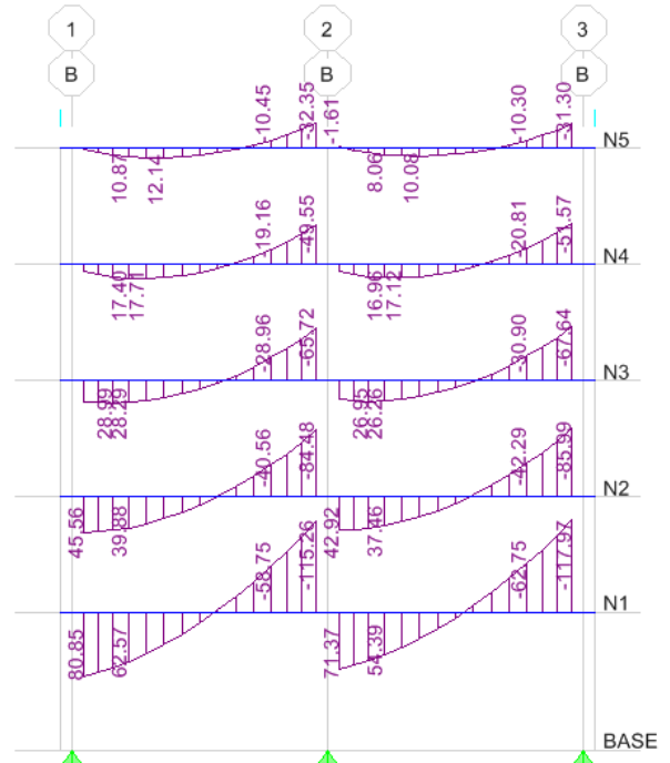
MARCO EJE B
