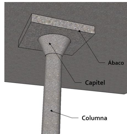
Figura I-8 Detalle de capitel y ábaco en columna circular.
