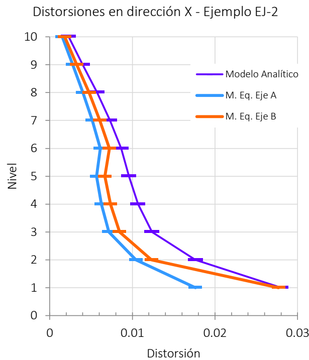
Figura IV-17 Gráficas de distorsiones - Ejemplo EJ-2
