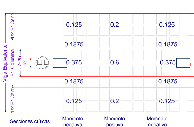
Figura II-7 Distribución del momento para el dimensionamiento por flexión ante cargas verticales de acuerdo con la sección 8.5 de las NTC-C
