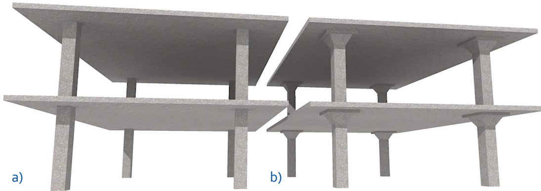
Figura I-9 Losas planas: a) Placa plana; b) Losa plana con columnas con ábaco y capitel.
