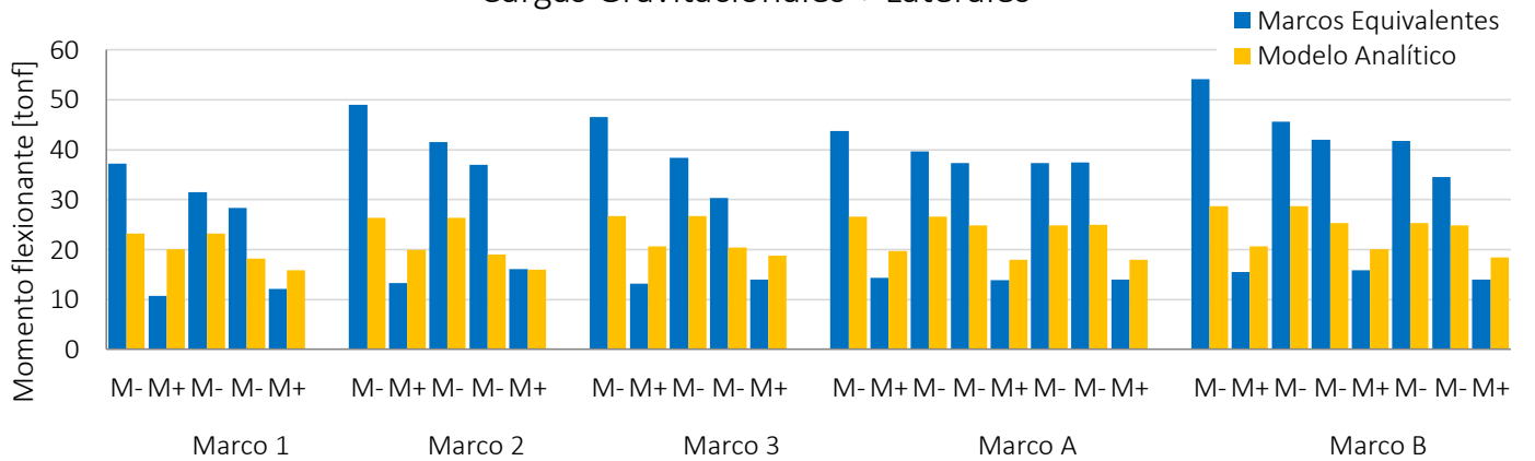
Figura IV-5 Gráfica de momentos Marco Equivalente vs. Modelo Analítico. Ejemplo Ej-2
