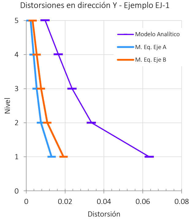
Figura IV-15 Gráficas de distorsiones - Ejemplo Ej-1
