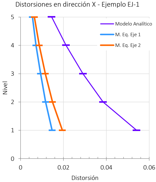
Figura IV-15 Gráficas de distorsiones - Ejemplo Ej-1
