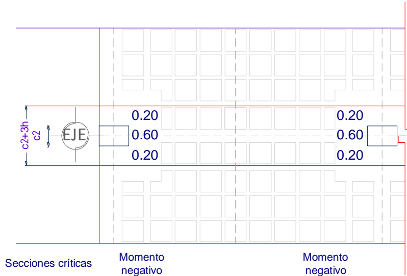
Figura II-8 Distribución del momento para el dimensionamiento por flexión ante cargas laterales de acuerdo con la sección 8.5 de las NTC-C
