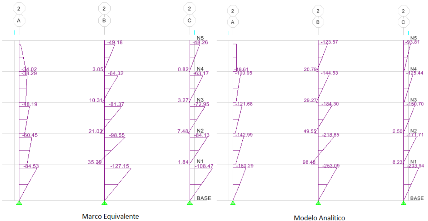
Figura IV-8 Momentos flexionantes en columnas Ejemplo EJ-1
