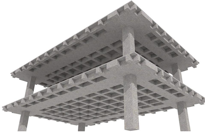
Figura I-10 Losa reticular. Se aprecia la zona maciza alrededor de columnas y entre ejes de columnas.
