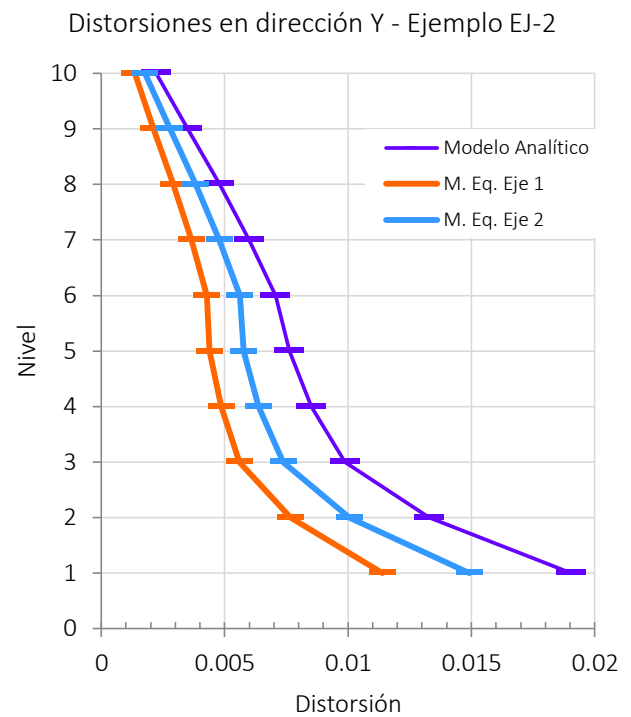
Figura IV-17 Gráficas de distorsiones - Ejemplo EJ-2
