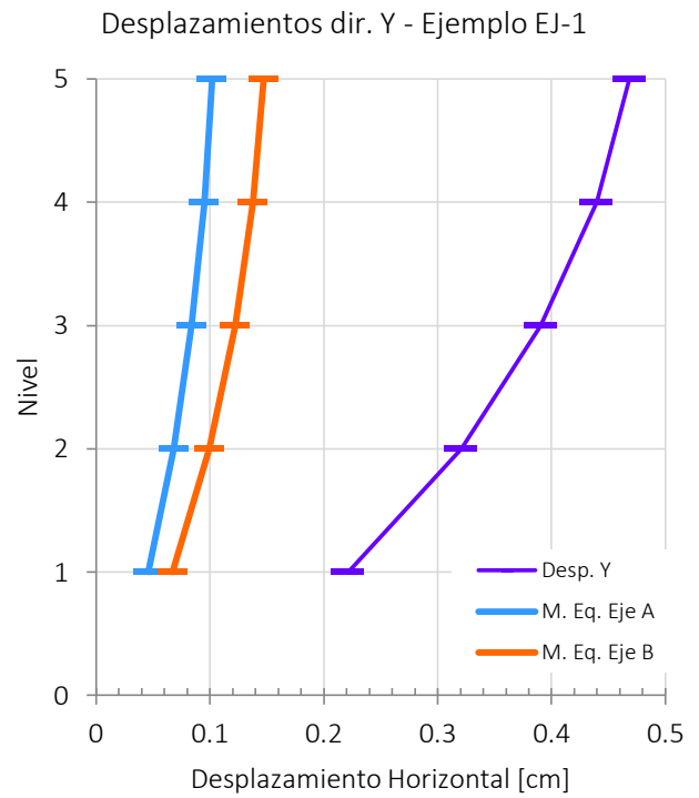
Figura IV-14 Gráficas de desplazamientos - Ejemplo EJ-1
