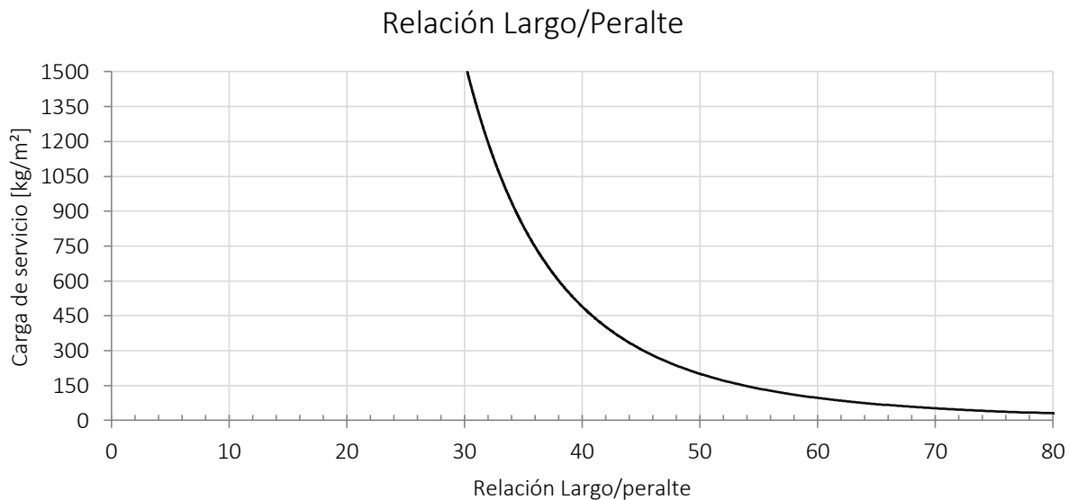
Figura II-4 Gráfica claro/peralte.
