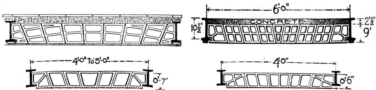
Figura I-3 Sistemas de piso de arcos planos hechos con bloques de cemento, típicos a finales del siglo XIX y principios del XX
