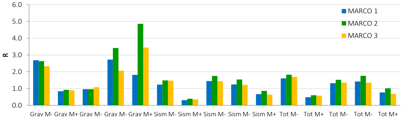
Figura IV-6 Relación MNTC/MMAN por condición de análisis. Ejemplo EJ-2
