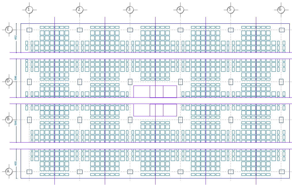
Marcos equivalente en la dirección X
