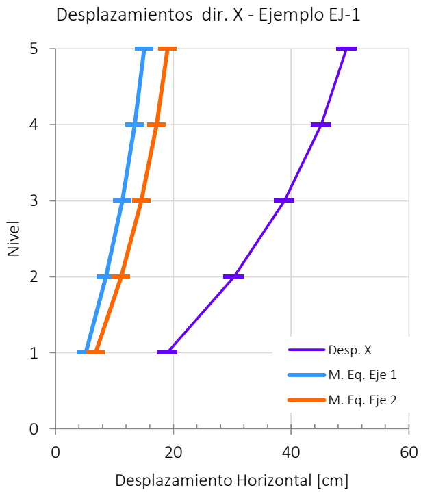
Figura IV-14 Gráficas de desplazamientos - Ejemplo EJ-1
