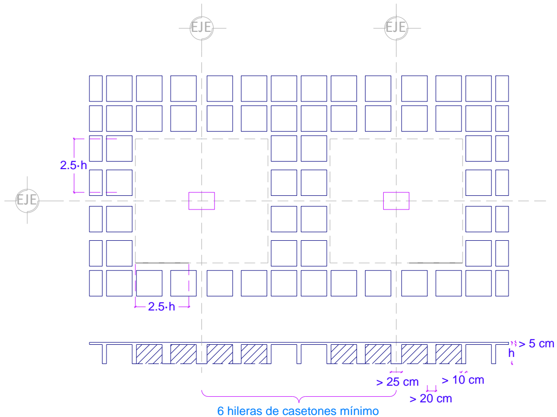
Figura II-1 Requisitos geométricos generales para losas planas aligeradas de acuerdo con NTC-C, RCDF-04.
