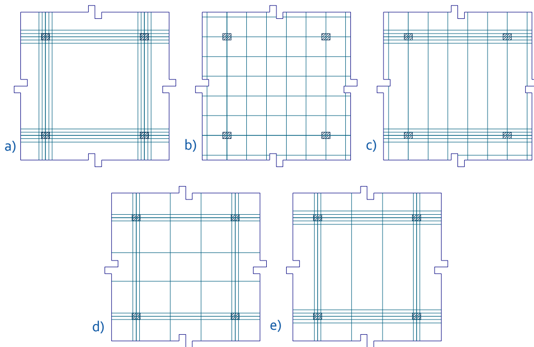
Figura I-11 Diversos arreglos de tendones en losas presforzadas.
