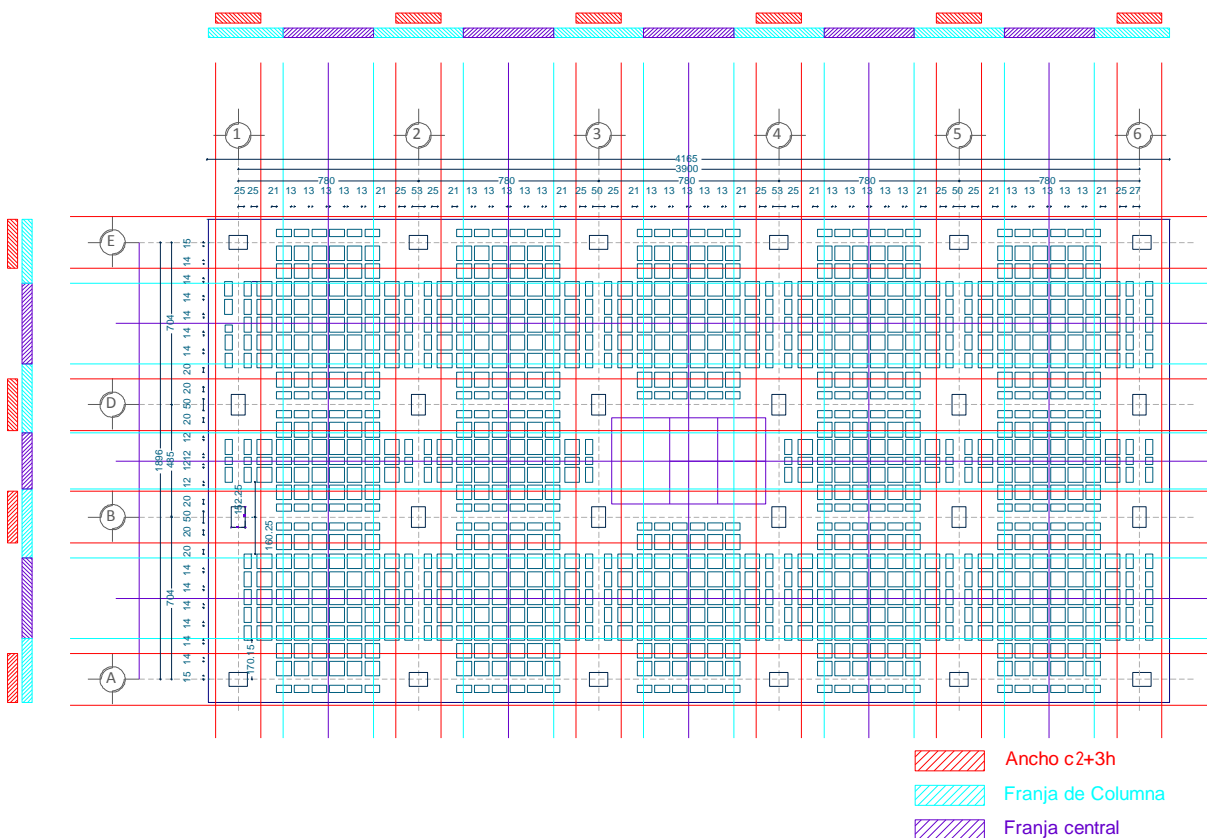
Figura III-16 División para el análisis por marcos equivalentes. Ejemplo EJ-2
