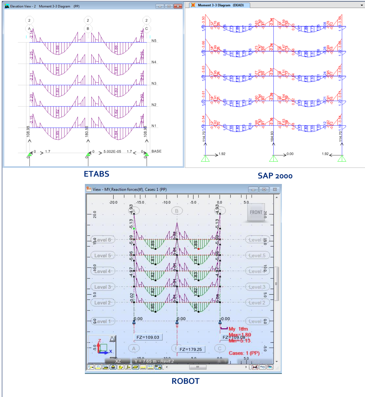
Figura III-4 Reacciones y Momentos para la condición de carga de Peso Propio en la elevación 2 en los diferentes programas analizados.
