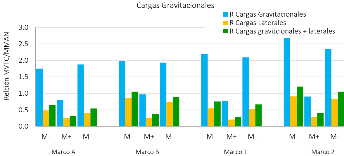
Figura IV-2 Relación MNTC/MMAN por marco. Ejemplo EJ-1
