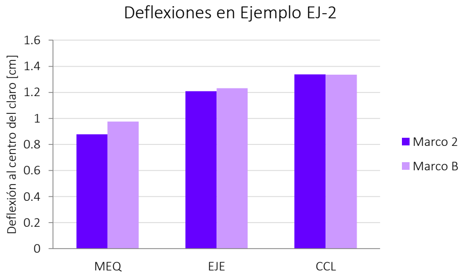
Figura IV-13 Deflexiones en ejemplo EJ-2
