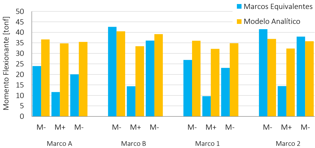
Figura IV-1 Gráfica de momentos marco equivalente vs. Modelo analítico. Ejemplo Ej-1
