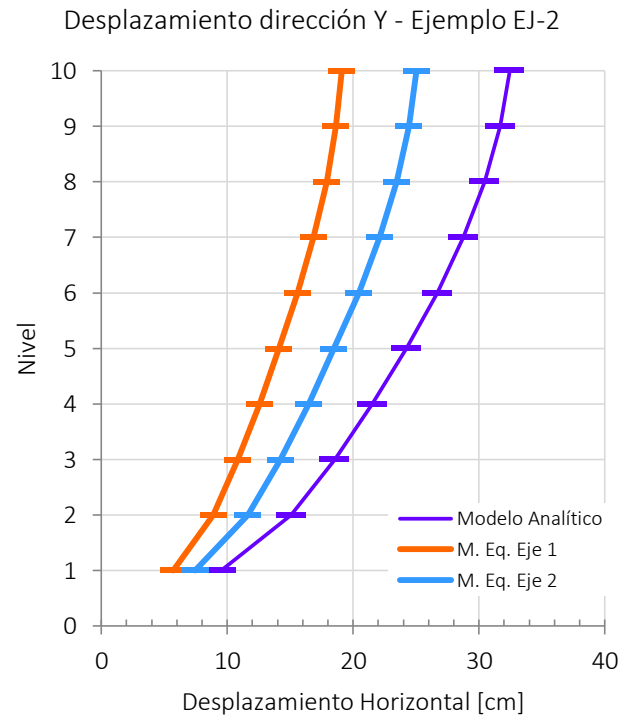
Figura IV-16 Gráficas de desplazamientos - Ejemplo EJ-2
