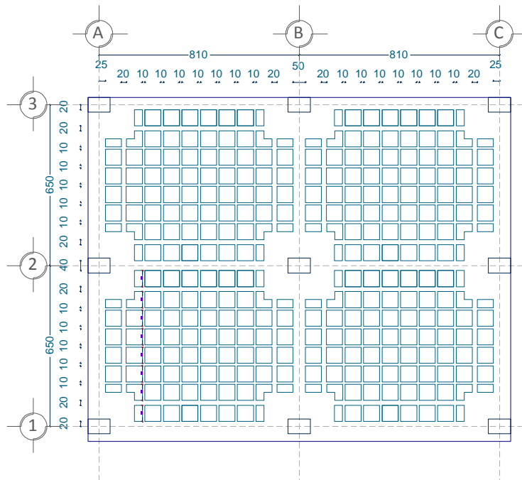
Figura III-2 Distribución de casetones para el ejemplo EJ-1
