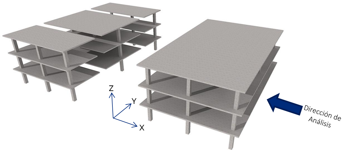
Figura II-6 Marcos equivalentes de la estructura en dirección X
