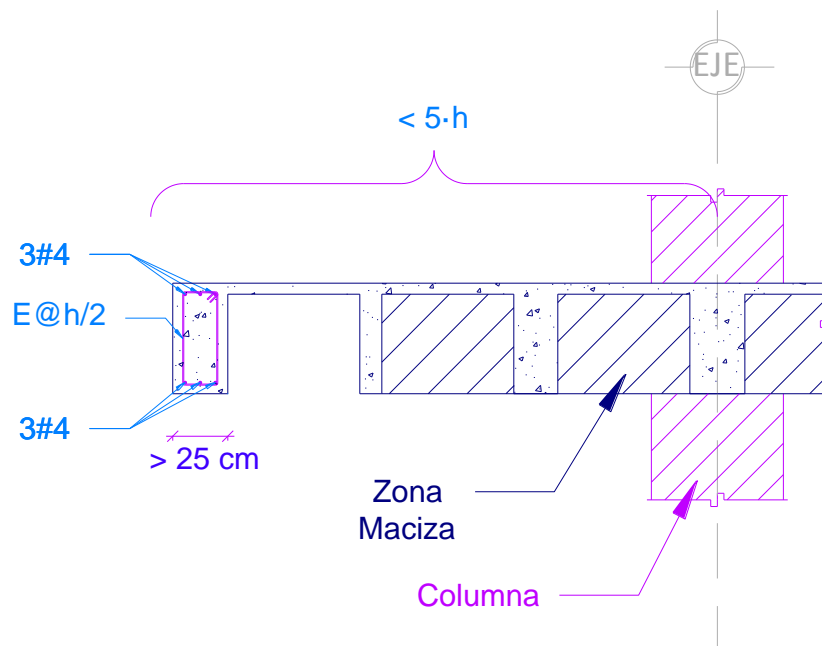
Figura II-2 Recomendaciones para borde de losa plana aligerada.
