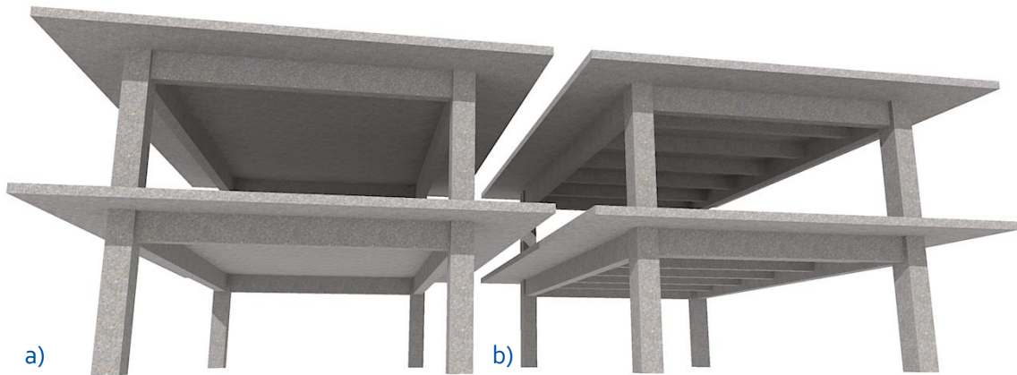
Figura I-7 Losas soportadas por vigas: a) Losa en dos direcciones; b) Sistema de travesaños y vigas con losa en una dirección
