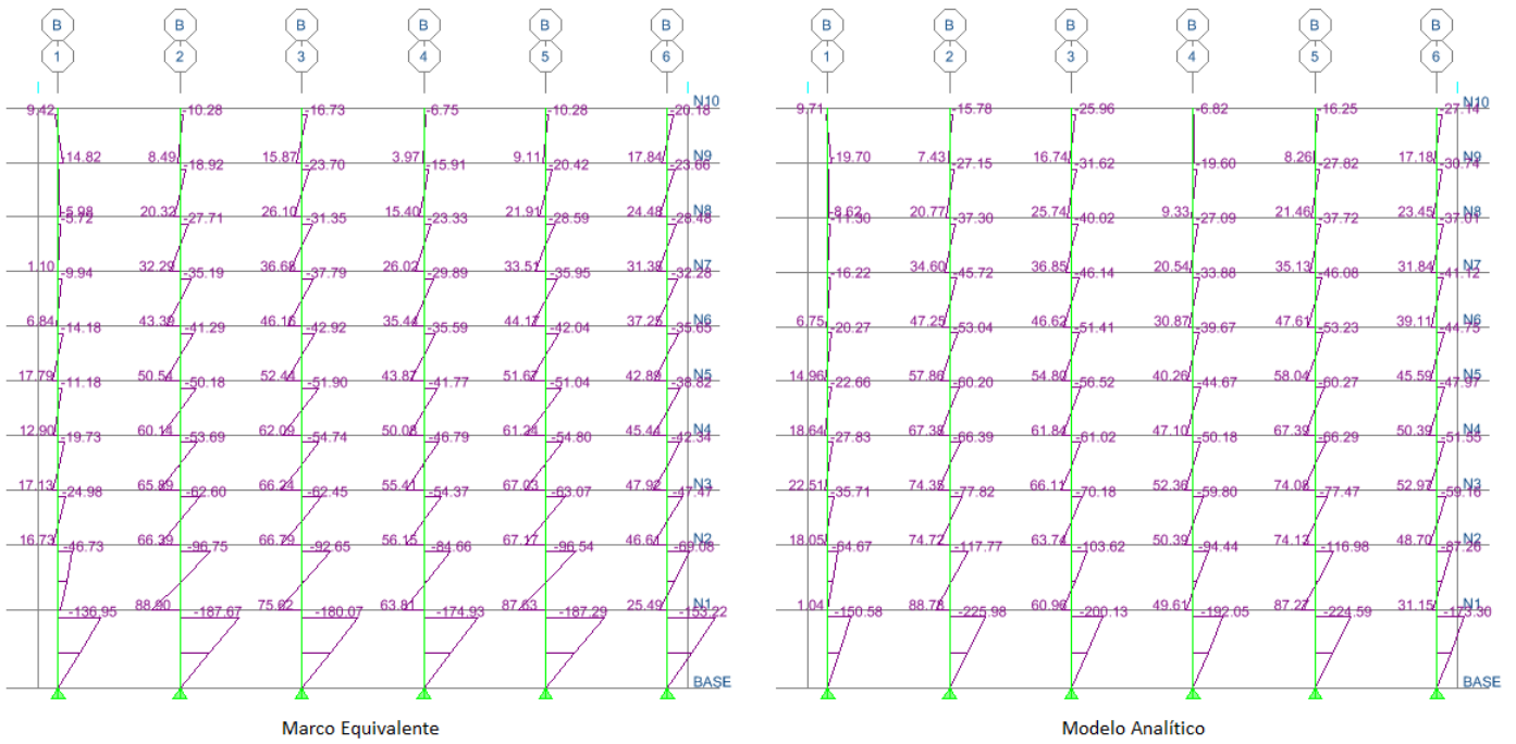
Figura IV-9 Momentos flexionantes en columnas. Ejemplo Ej-2
