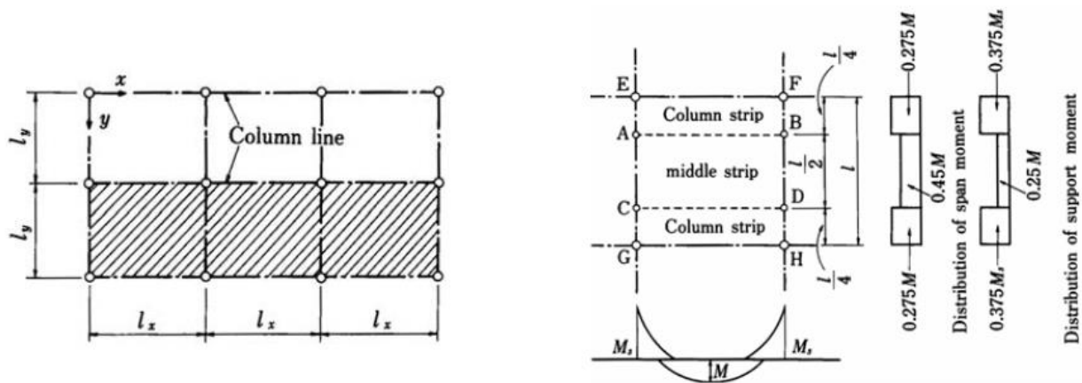
Figura II-9 Distribución del momento en franjas centrales y de columna conforme al reglamento AIJ.
