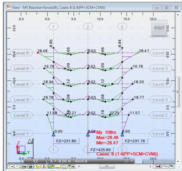
Figura III-5 Diagramas de momento para la condición de carga de Grav=1.4(PP+SCM+CVM) en los ejes 2 y B en los tres programas de cálculo.
