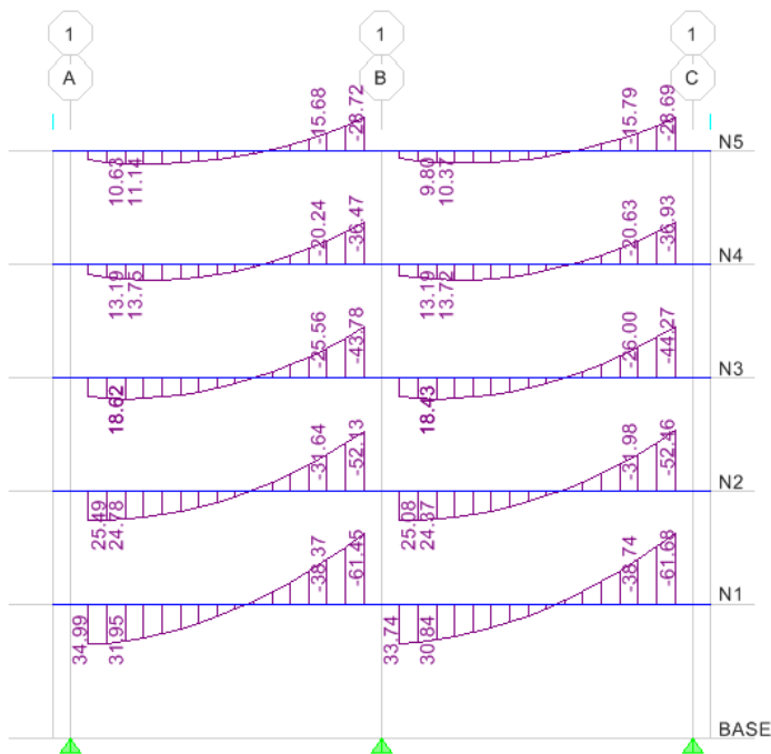
MARCO EJE 1
