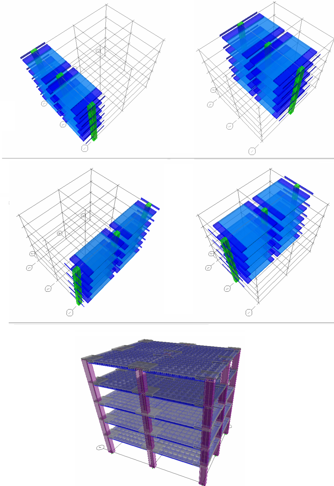
Figura III-14 Marcos equivalentes y modelo completo. Ejemplo EJ-1
