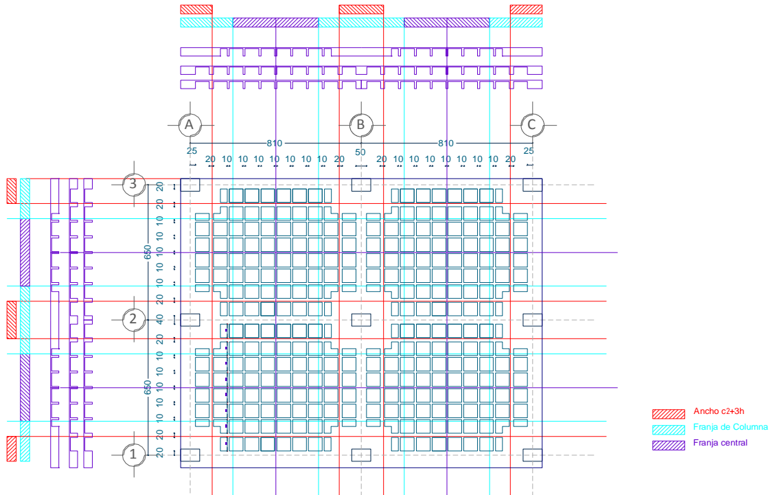
Figura III-7 Tablero a analizar y su división para el análisis por marcos equivalentes. Ejemplo EJ-1
