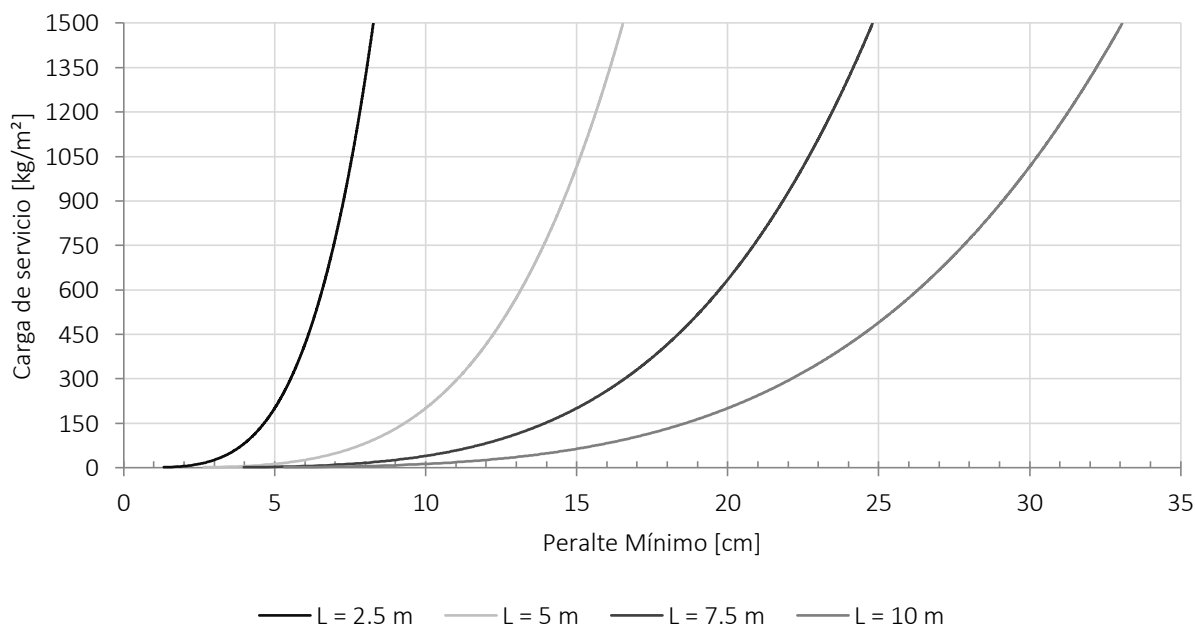
Figura II-3 Gráfica de peraltes mínimos calculados con la sección 8.10 de las NTC-C
