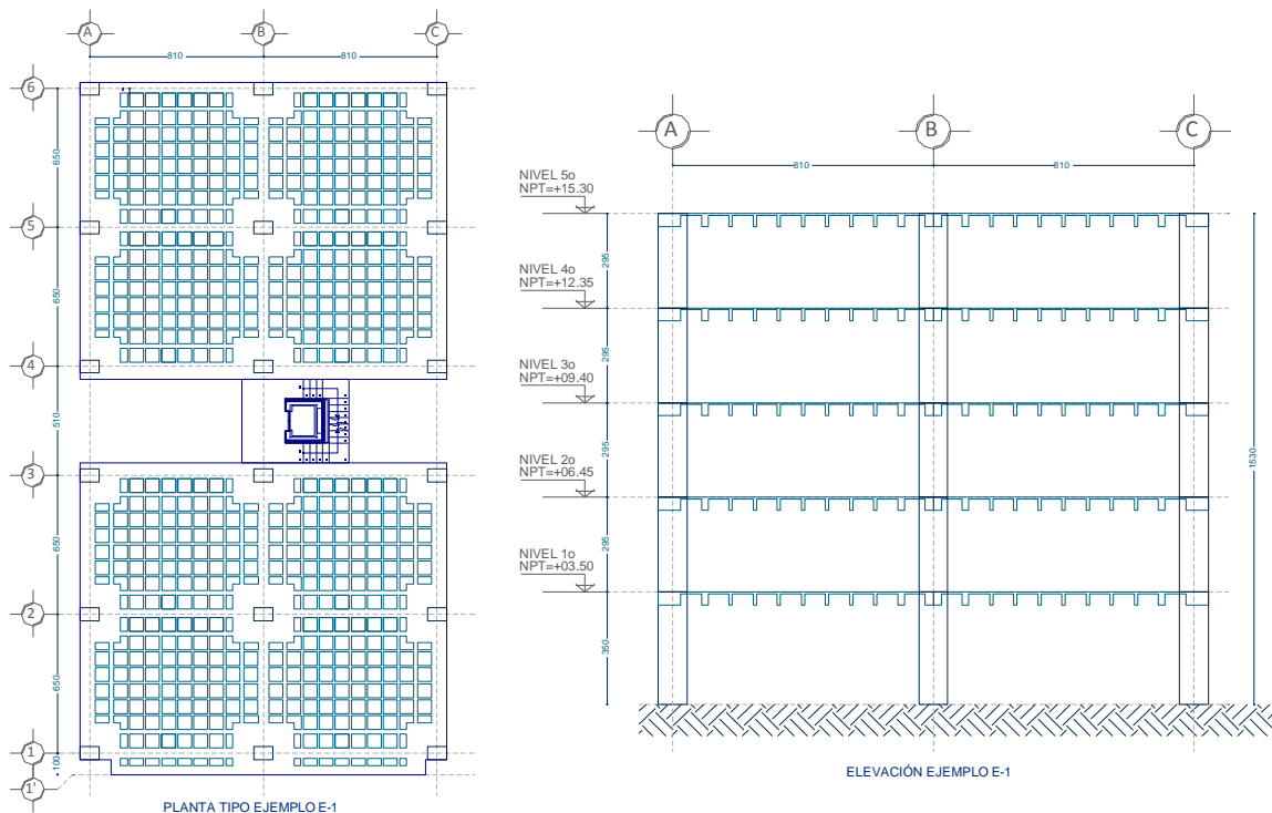
Figura III-1 Planta tipo y elevación. Ejemplo EJ-1
