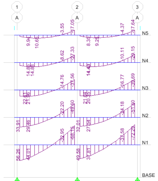
MARCO EJE A
