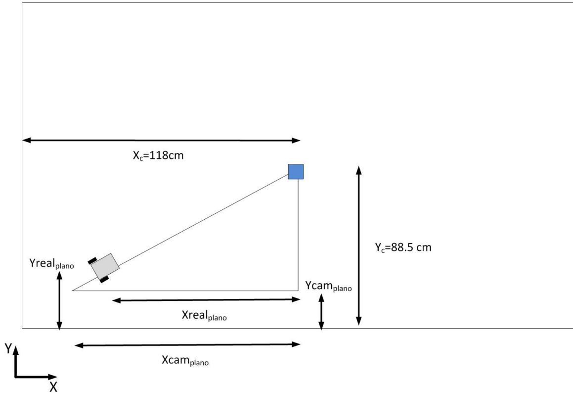
Figura 6.18: Corrección de coordenadas de cámara plano XY
