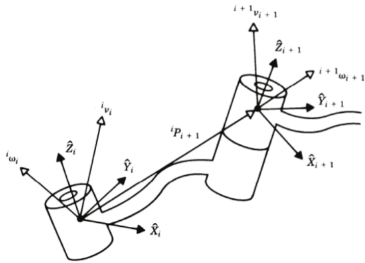
Figura 4.4: Metodo de propagación de velocidades del eslabón i al i+1
