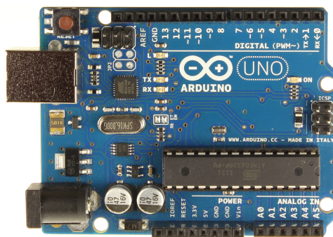
Figura 5.10: Tarjeta de desarrollo Arduino Uno
