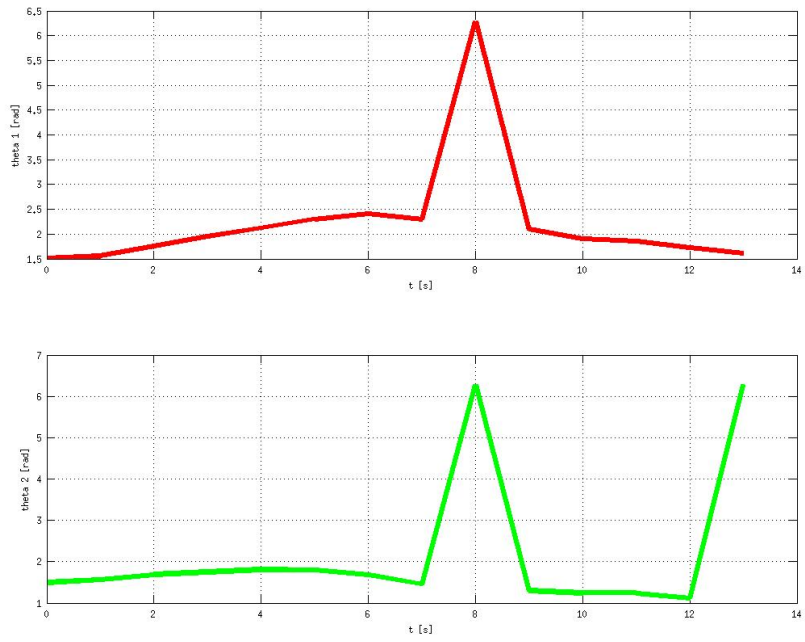
Figura 6.32: Orientación de los robots durante el transporte
