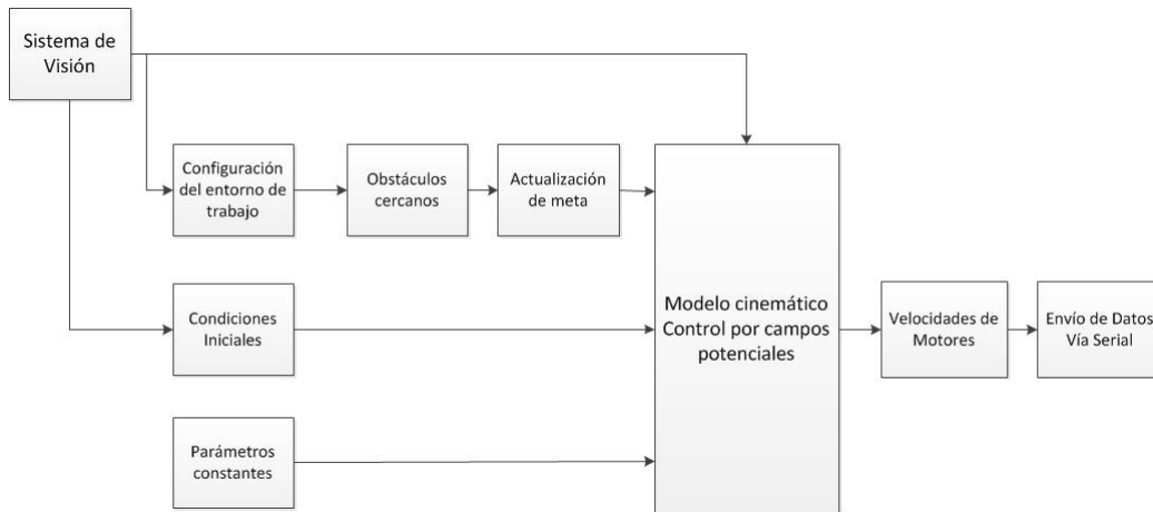
Figura 6.19: Funcionamiento Control en Tiempo Real
