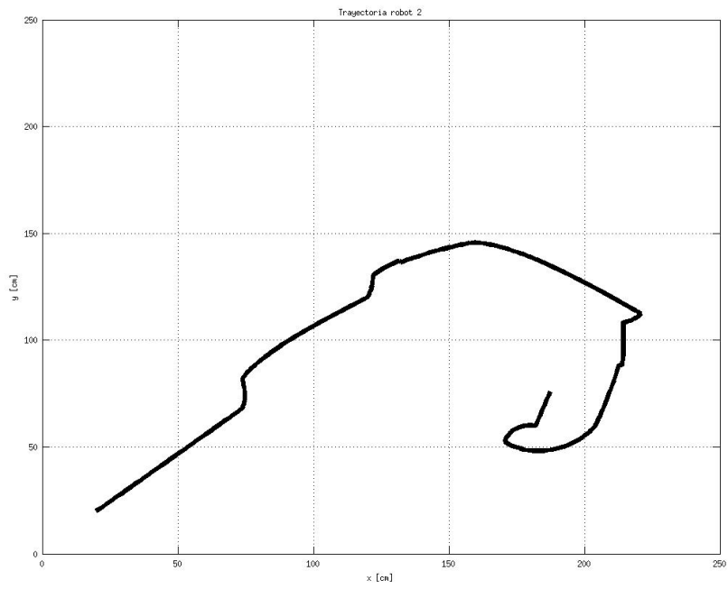
Figura 6.6: Trayectoria del robot 2
