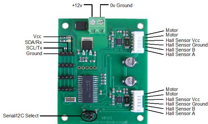
Figura 5.12: Tarjeta MD25
