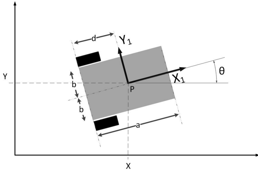
Figura 4.2: Robot tipo 2.0
