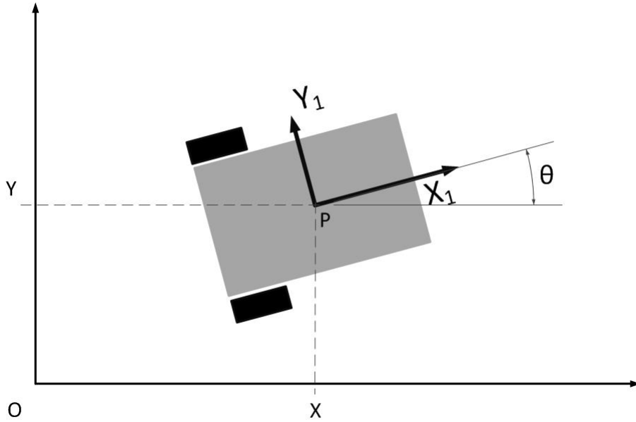
Figura 4.1: Postura de un robot móvil
