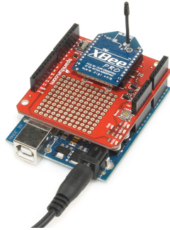
Figura 5.11: Xbee shield
