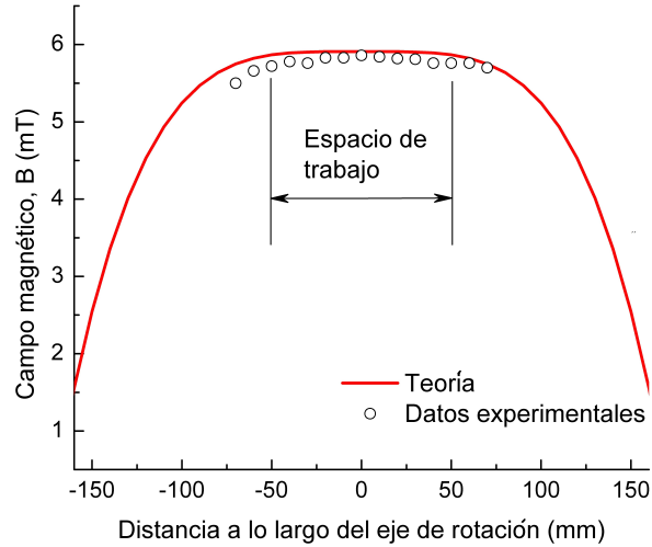
Figura 3.4: Campo magnético a lo largo del eje de rotación de las bobinas [7].
