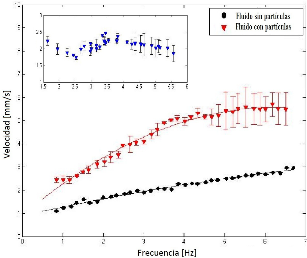
Figura 4.7: Nadador con cola de flexibilidad media en los fluidos con y sin partículas. Las líneas continuas representan ajustes polinomiales de segundo orden. El recuadro superior izquierdo de la figura muestra la relación de velocidades, R = \frac{V_{cp}}{V_{sp}} , contra la frecuencia adimensional, f^* = \frac{f \cdot D}{V_{cp}} , donde D es el diámetro de la cabeza, V_{cp} y V_{sp} las velocidades en el fluido con y sin partículas respectivamente.
