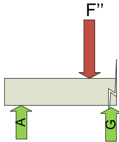
Figura C.7 Diagrama de cuerpo libre con el apoyo G
