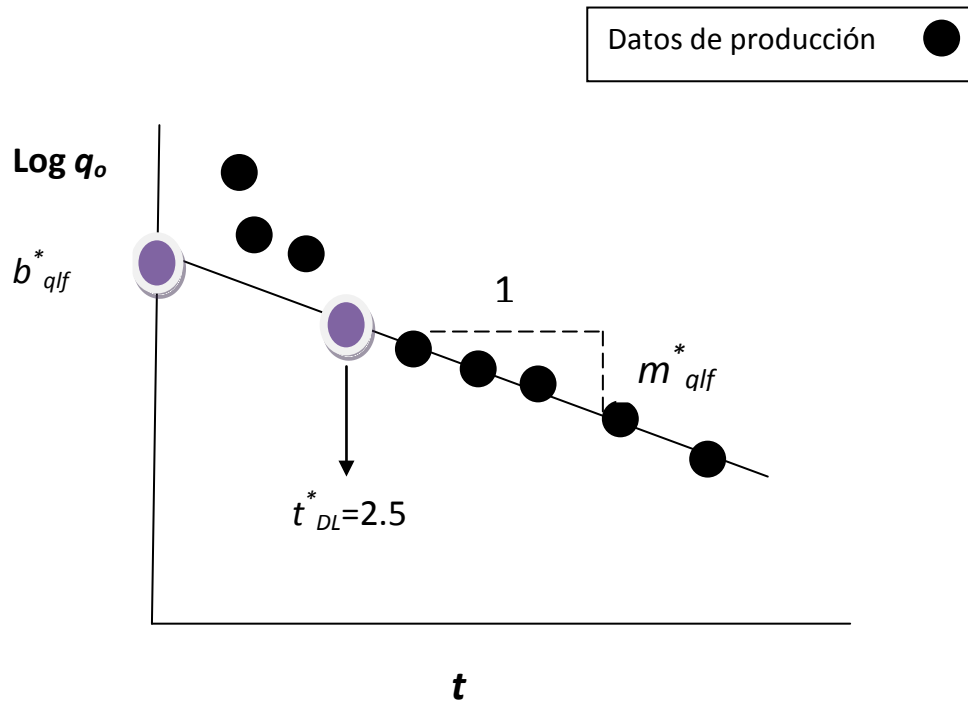
Figura 12 Gráfica de declinación exponencial para el análisis de datos de producción.
