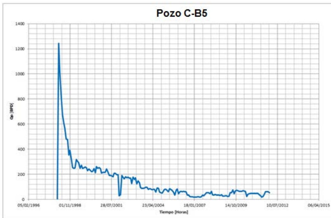
Fig. 3.11 Historia de producción del pozo C-B5
