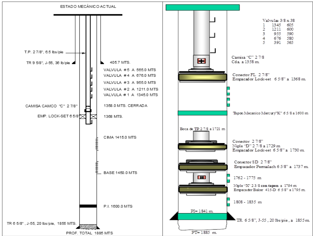
(A) (B) Figura 5.1a. Estado Mecánico del Pozo FI-123 antes de la instalación del Sistema Gravitacional
