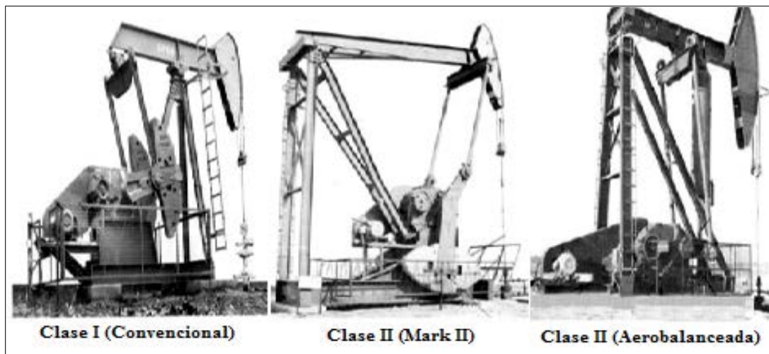
Fig.2.2b - Geometrías de Unidades de Bombeo Tipo Balancín
