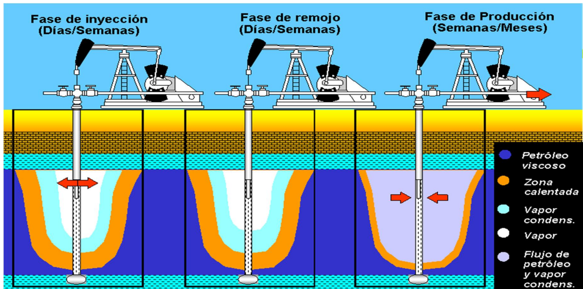
Figura 1.1 Fases de la Inyección Cíclica de Vapor
