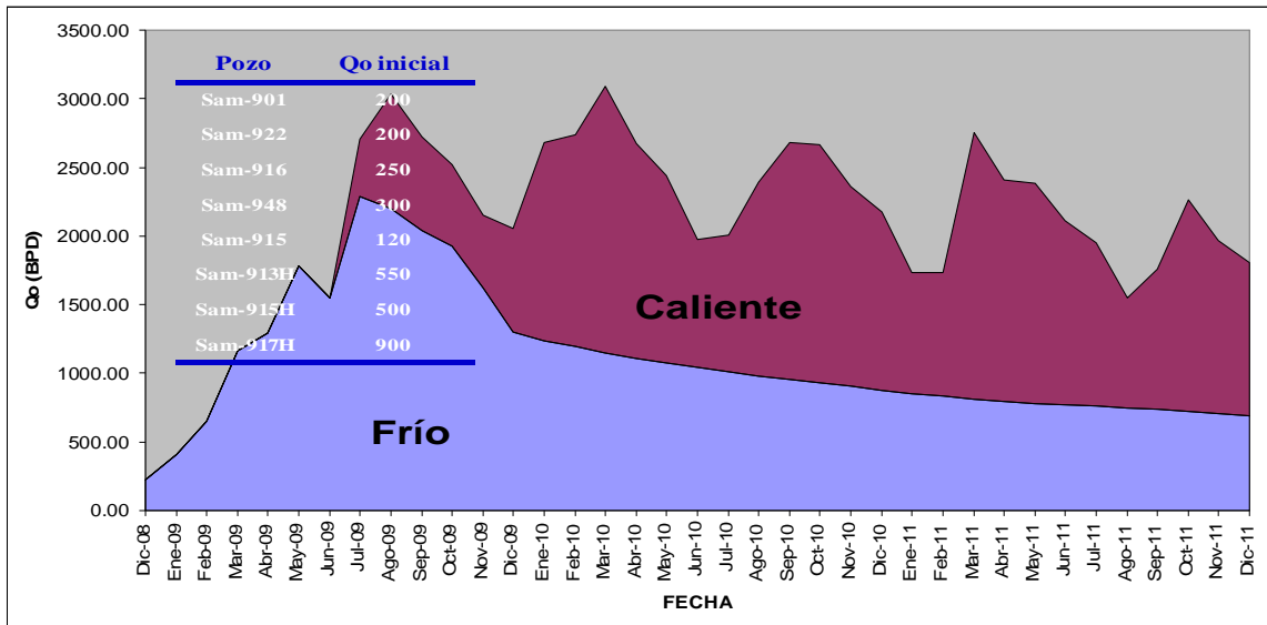
Figura. 4.12 Comportamiento del gasto de aceite extra pesado, en frío y en caliente fuente: Pemex
