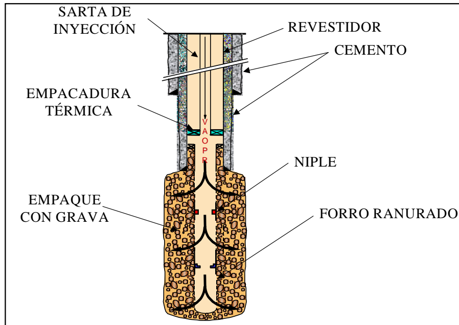
Figura 4.10 Empacador Térmico
