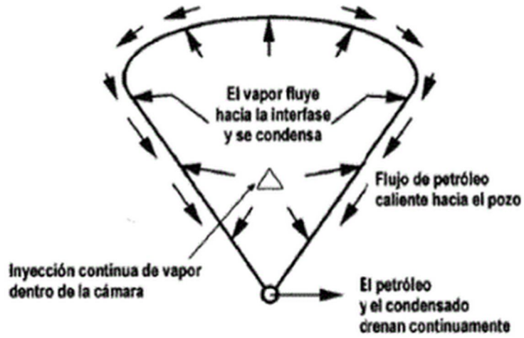
Figura.3.2. 2- Proceso de drenaje por gravedad asistido con Vapor (Butler)
