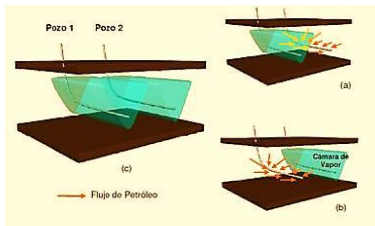
Figura 3.2 a, 3.2 b, 3.2 c proceso HASD
