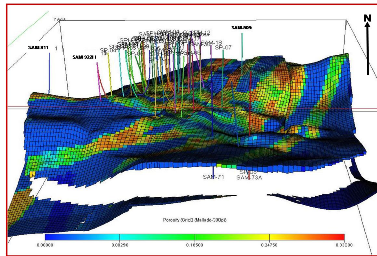
Figura 4.8 -Modelo de Simulación del campo Samaria Neógeno fuente: Pemex
