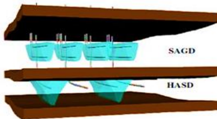
Figura 3.3 Comparación del Proceso HASD vs SAGD
