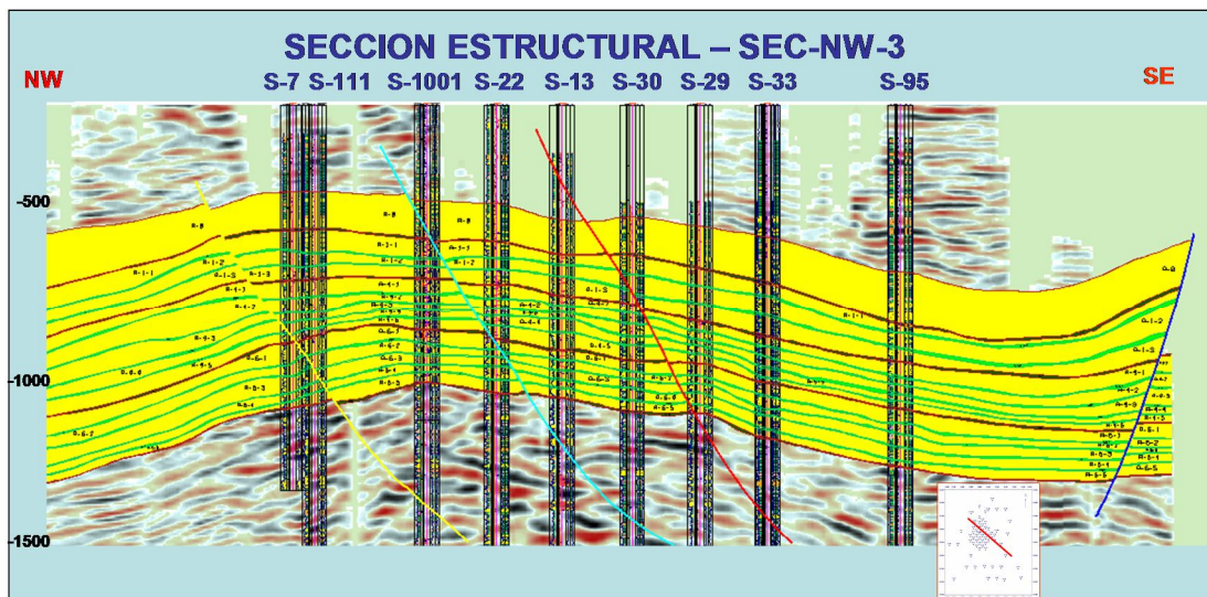
Figura 4.5: Sección estructural de un Campo de la Región Sur. fuente: Pemex
