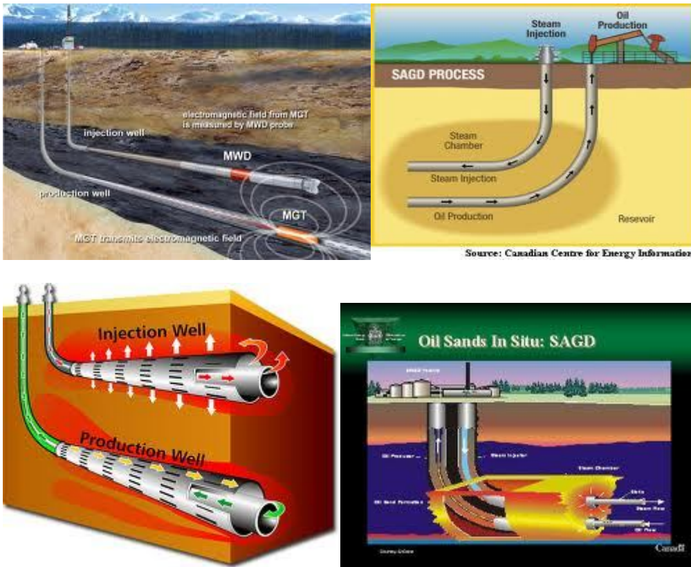
Figura 3.2.3 Imágenes Para Ilustrar el Método SAGD
