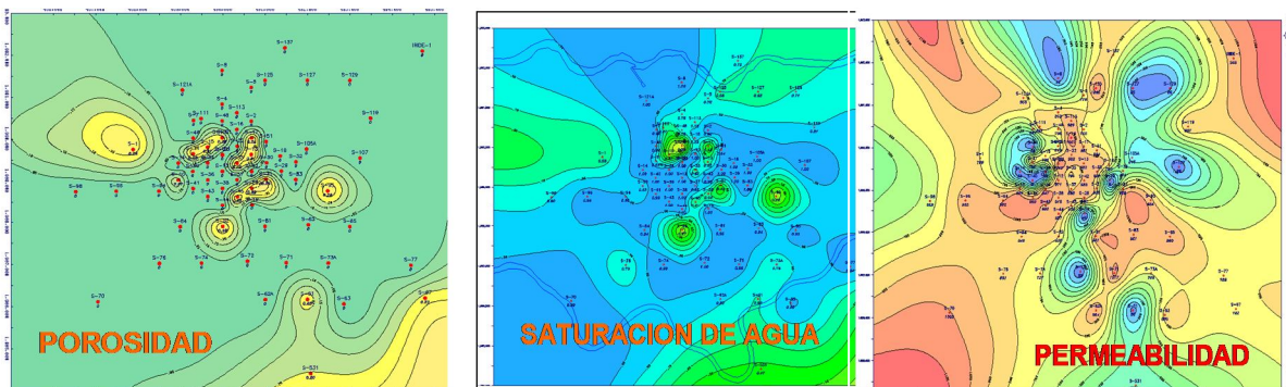
Figura 4.7.- Plano de Isopropiedades de un campo en la región sur. fuente: Pemex
