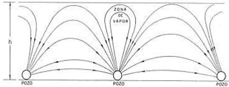
Figura 3.1 Inyección Cíclica de Vapor en Pozos Horizontales
