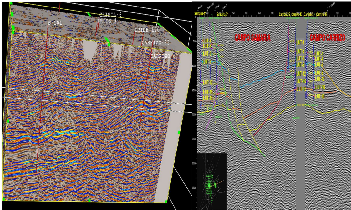
Figura 4.4. Sección sísmica del bloque. fuente: Pemex
