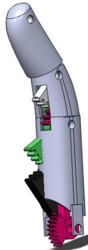
Figura 3.7: Mecanismo con la carcasa.
