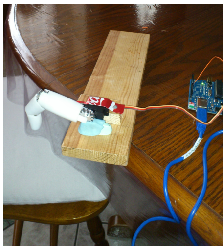
Figura 7.14: Flexión máxima del dedo.
