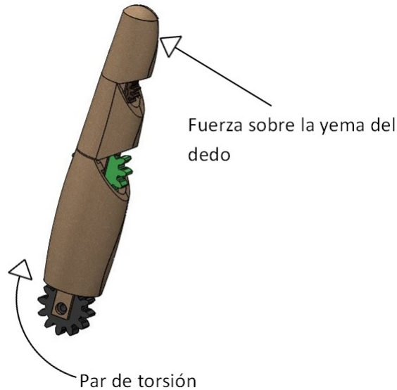
Figura 4.4: Esquema de la fuerza del dedo y el par de torsión.
