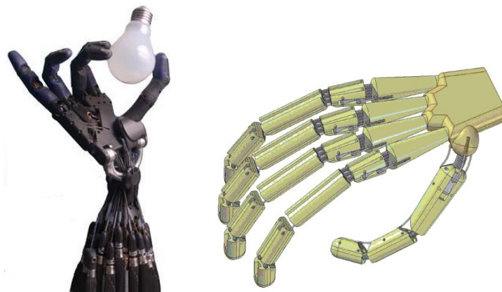
a) Shadow Hand[11].
