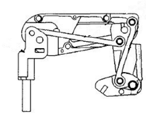
Figura 1.5: Mecanismo de 4 barras en la mano Robonaut [12].
