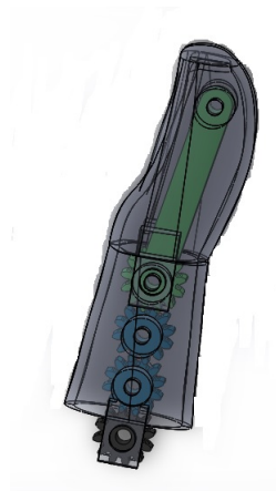
Figura 3.19: Mecanismo pulgar.
