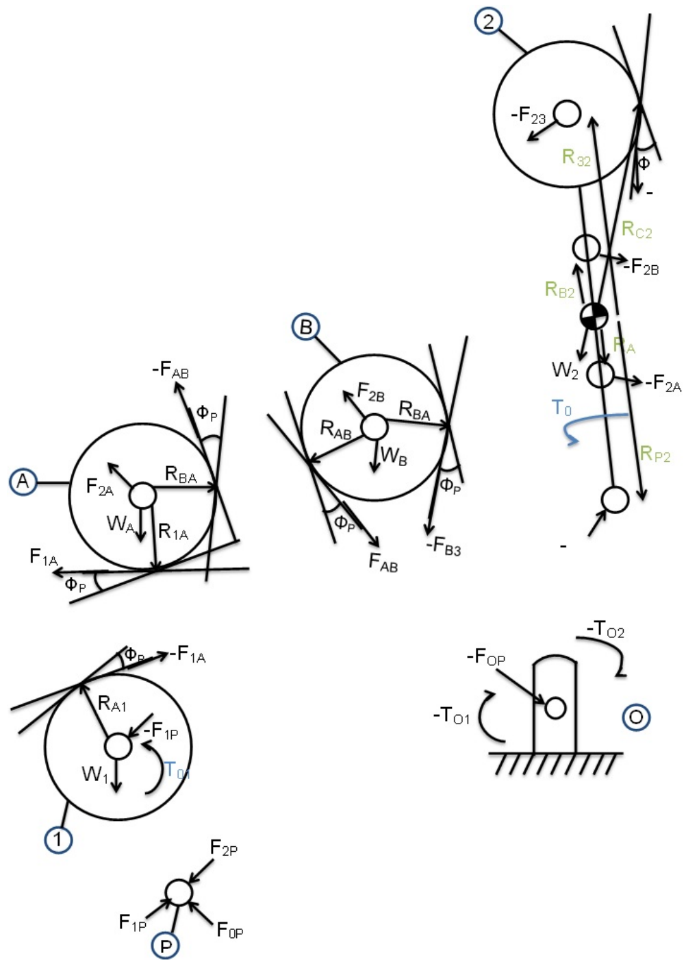
Figura 4.2: Diagramas de cuerpo libre 1 del dedo medio.
