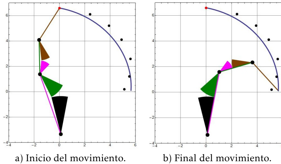
Figura 3.5: Movimiento flexión-extensión del mecanismo.
