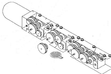
Figura 1.11: Configuración del dedo de la mano NTU [23].
