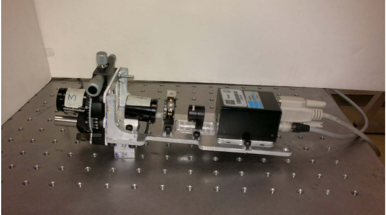
Figura 6.9 Ensamblaje del mecanismo de alineación M6 y los componentes ópticos del sensor.
