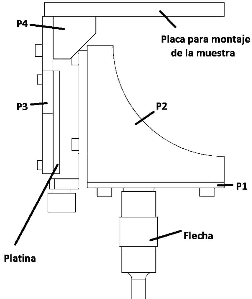
Figura 4.22 Vista lateral del mecanismo de ajuste M7.
