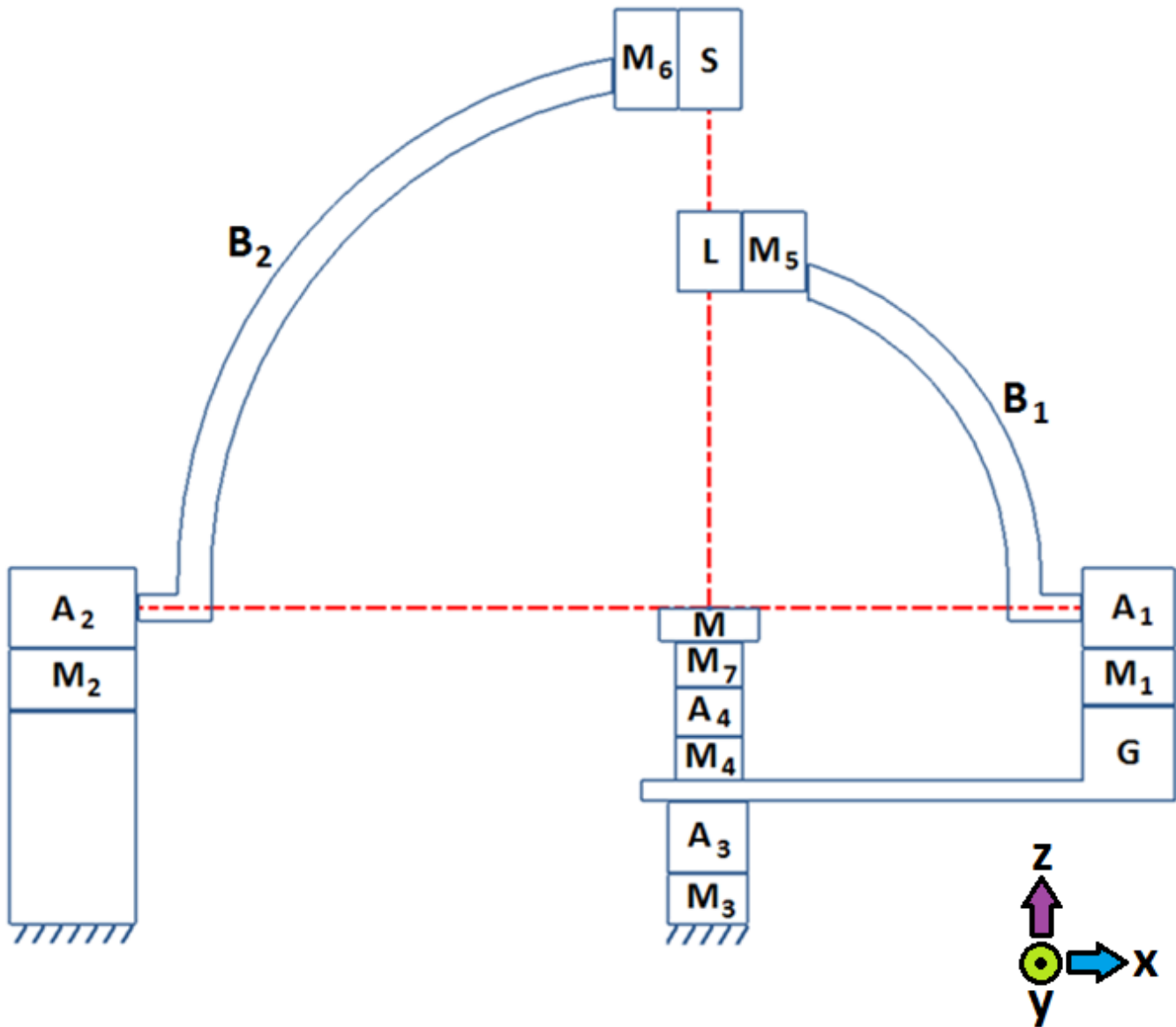
Figura 3.7 Mecanismos de alineación del equipo M_1 , M_2 ,..., M_7 .
