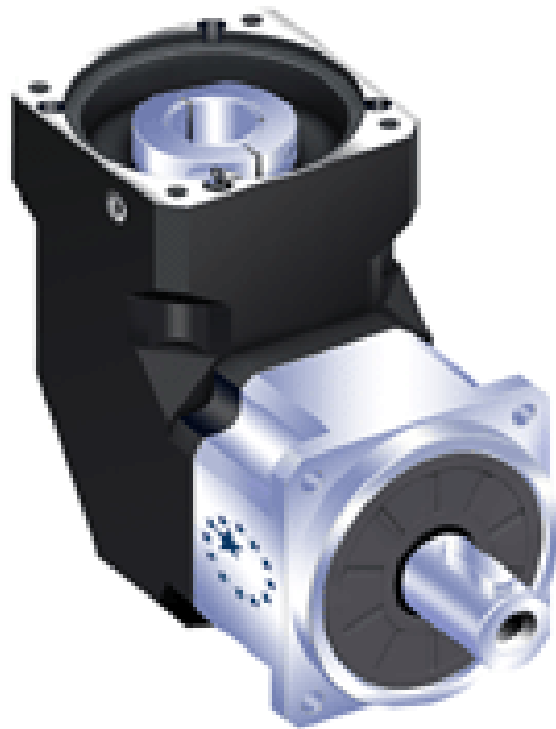
Figura 4.3 Reductor de velocidad ABR-060-070-S2-P1. Cortesía de Apex Dynamics, Inc.
