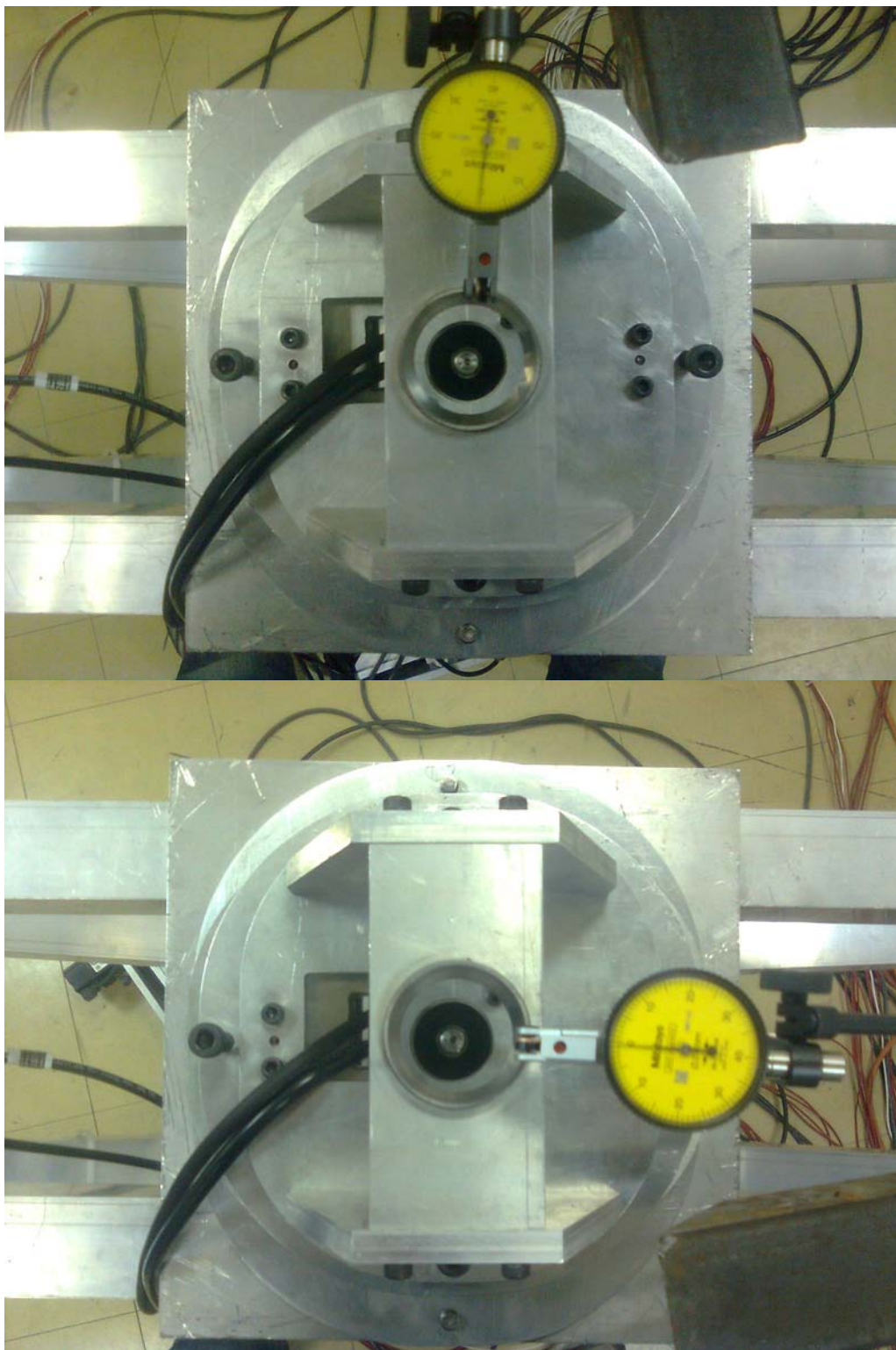
Figura 6.14 Alineación del mecanismo de giro de la muestra con el eje de giro del brazo G.
