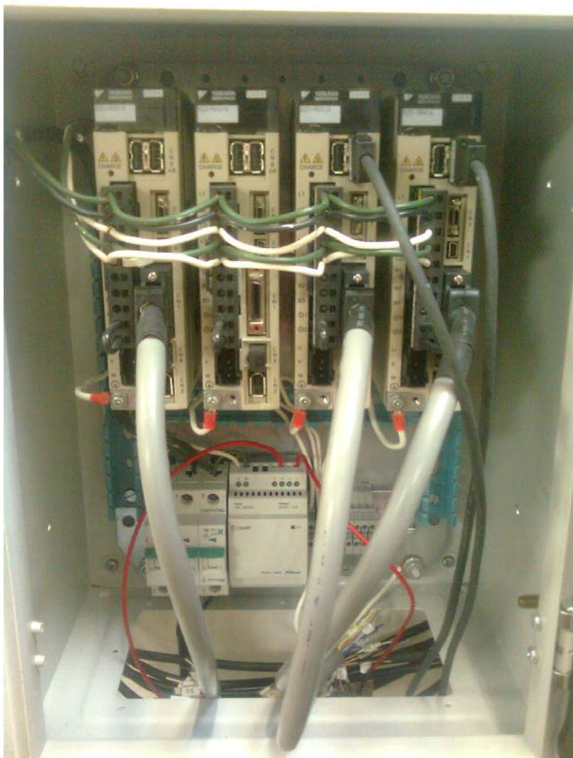
Figura 6.15 Gabinete que contiene los Servopacks.
