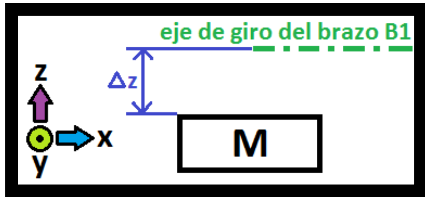
Figura 3.14 Ajuste de la altura de la muestra mediante el mecanismo M_7
