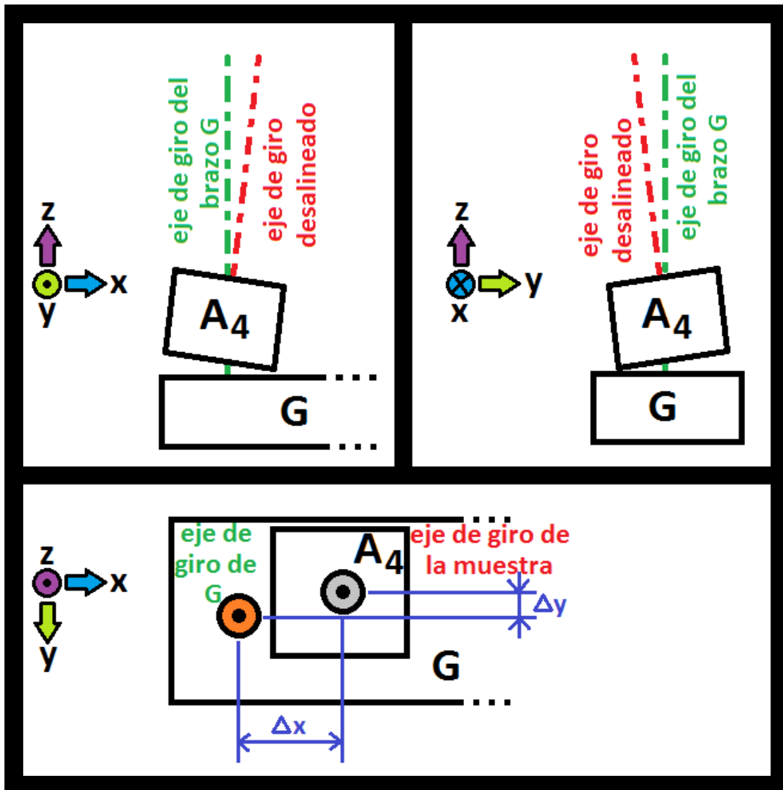
Figura 3.11 Desalineaciones que corregirá el mecanismo M_4
