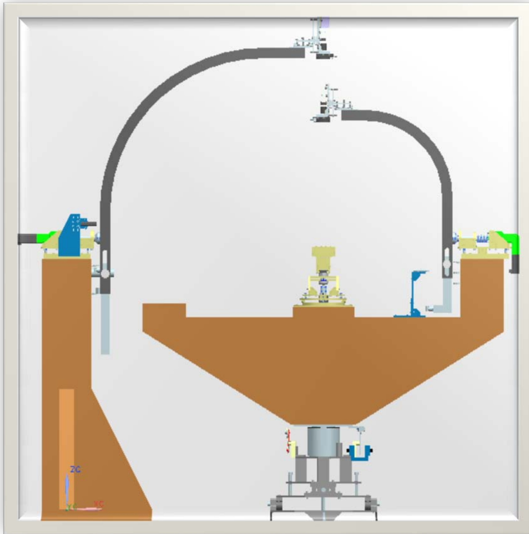
Imagen donde se pueden apreciar el ensamble completo del diseño.
