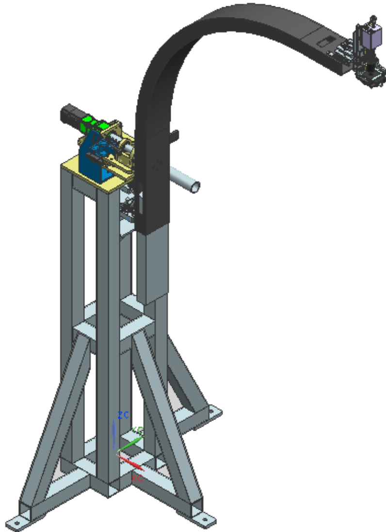
Figura 4.35 Ensamble del conjunto lateral del esparcímetro
