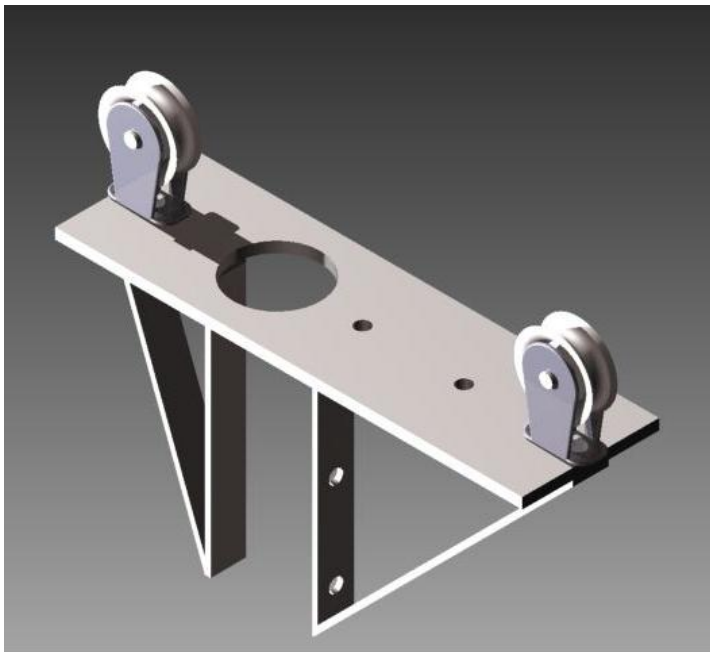
Figura 5.27 Soporte de las poleas
