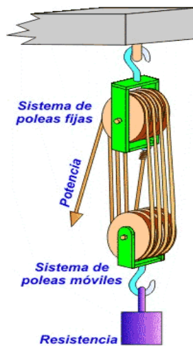
Figura 5.15 Variante de polipasto factorial
