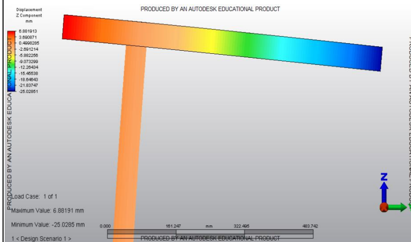
Figura 5.5 Desplazamiento de la estructura en el eje Z
