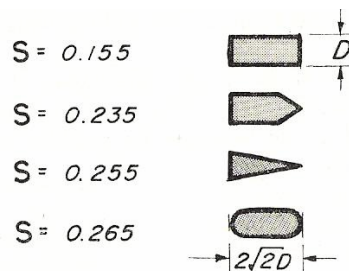
Fig. 4.1 Número de Strouhal para diferentes secciones.
