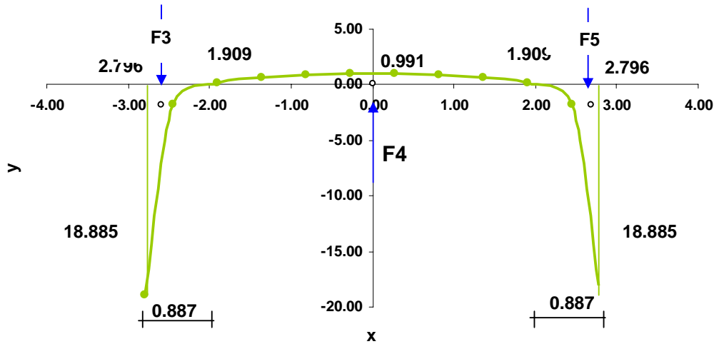
FIG. 7.9 Variación de C_p en la base de la sección triangular a 90^\circ
