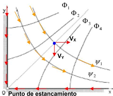
Fig. 1.21 Flujo hiperbólico de velocidad variable, con un punto de estancamiento.
