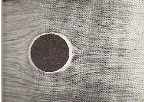
Fig. 3.6.- Flujo alrededor de un cilindro inmediatamente después de comenzar (flujo potencial).
