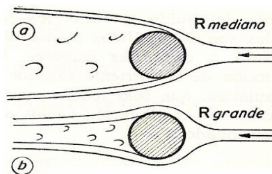
Fig. 3.4 Forma de la estela en flujo Laminar y turbulento
