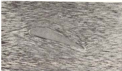
Fig. 3.53.- Líneas de corriente en una superficie aerodinámica en el primer momento después de comenzar.
