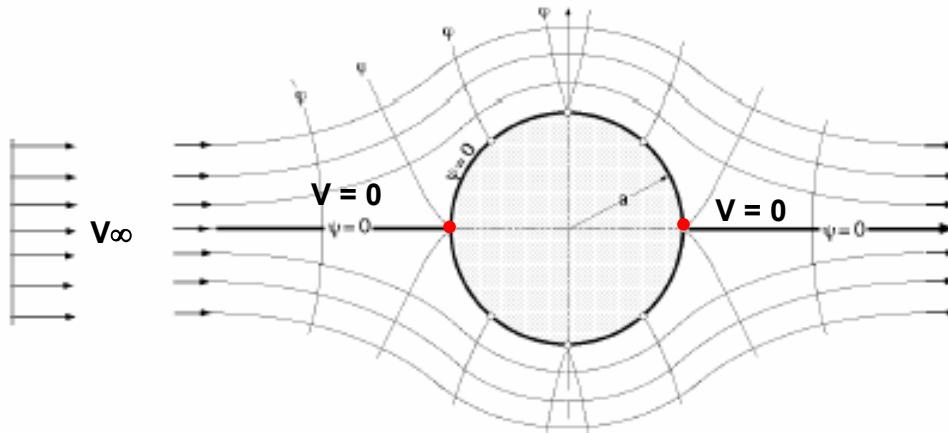
Fig. 1.38 Combinación de un Flujo Constante y un Doblete
