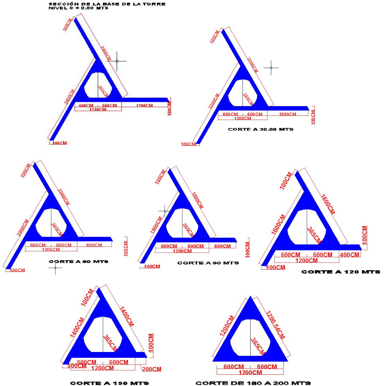
FIG. 7.1 Cortes transversales de la torre principal de soporte
