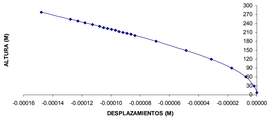
FIG. 7.7 CONFIGURACION MODAL DE LA TORRE CON CARGAS
