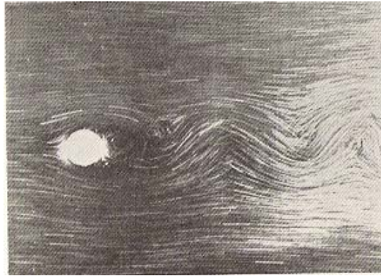
Fig. 3.64.- Estela de von Kármán wd/v = 250 . La cámara esta en reposo con respecto a el cilindro.
