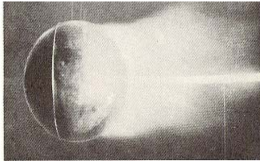
Fig. 3.40.- Debido a un anillo fino alrededor de la esfera, el flujo pasa a ser de otro tipo con capa de límite turbulenta. (Wieselsberger.)
