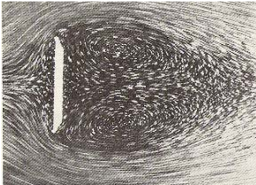
Fig. 3.67.- wb/v = 10.0
