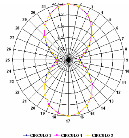
Fig. 6.18. Cp para una Separación de 3D
