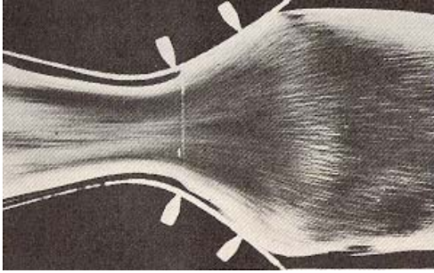
Fig. 3.43.- La vena fluida es succionada hacia ambas paredes. El flujo es de izquierda a derecha.
