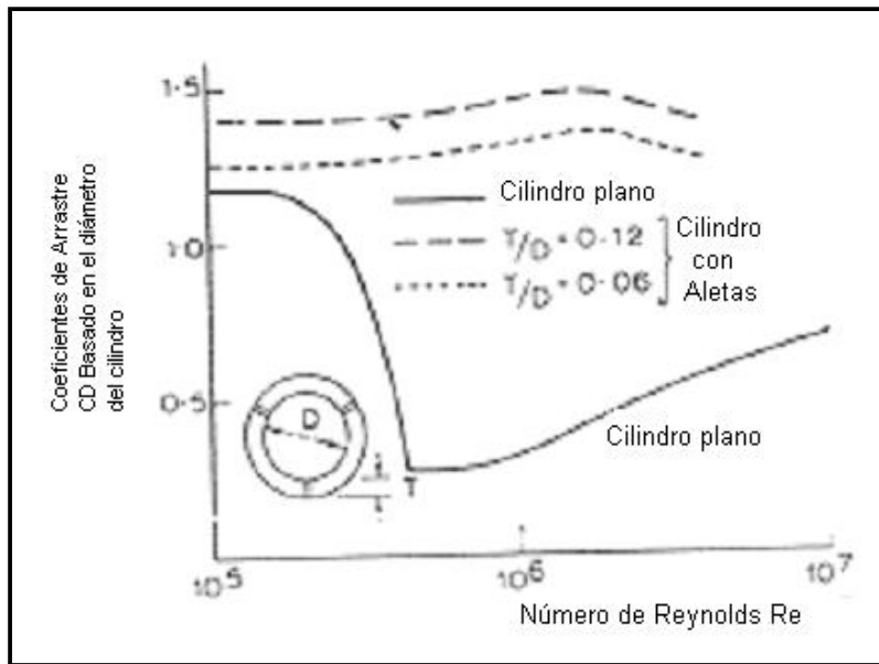
Fig. 5.7 Número de Reynolds contra Coeficiente de arrastre para un cilindro con barras contra vórtices.
