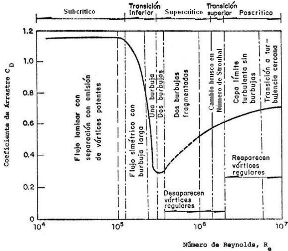
Fig. 2.3 Intervalos conocidos de flujos alrededor de un cilindro
