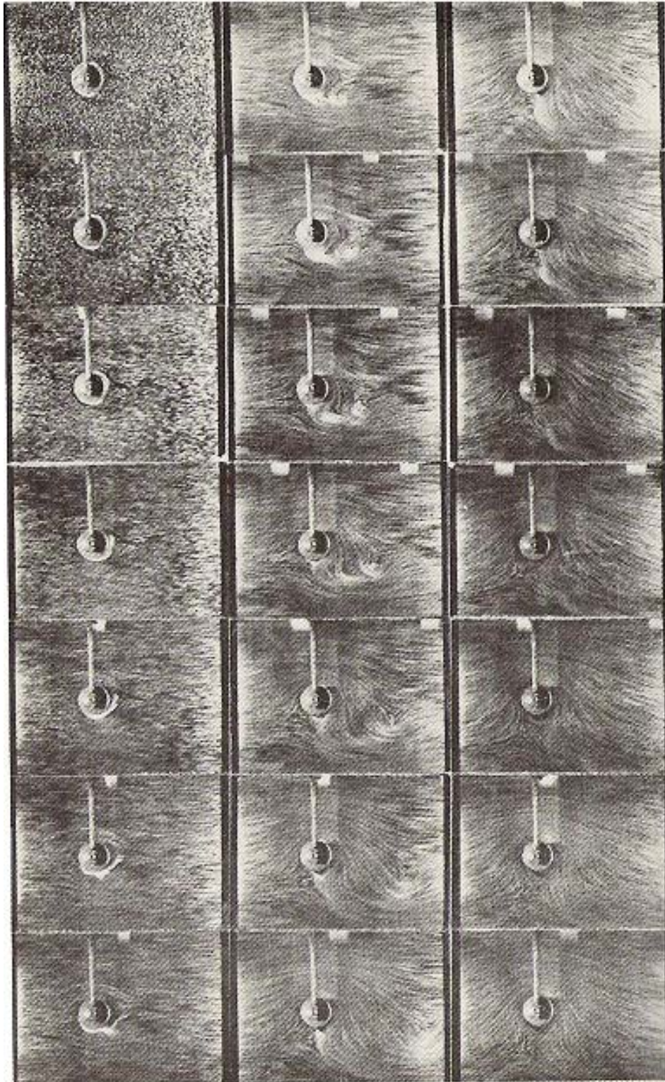
Figura 3.14. Igual que la figura 3.13, excepto que u/v = 6 , (ref. 1).
