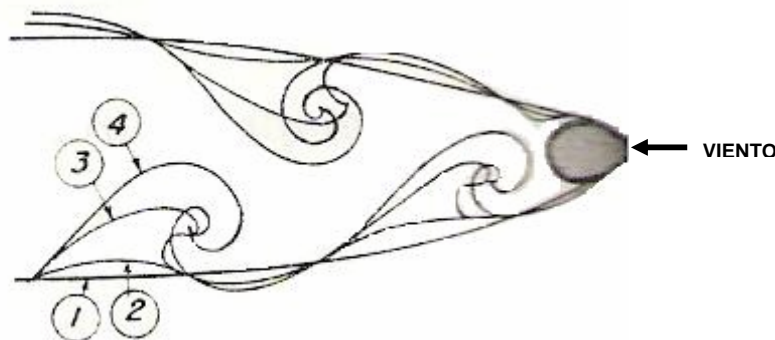
Fig. 3.5 Estela con vórtices alternados
