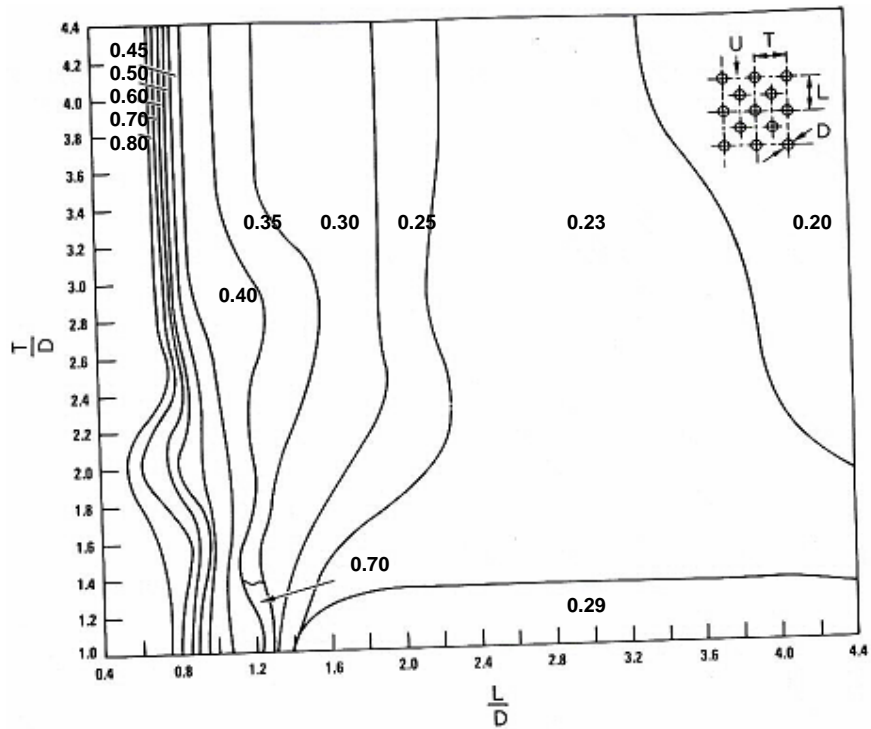
Fig. 4.4.- Número Strouhal para arreglos de cilindros escalonados
