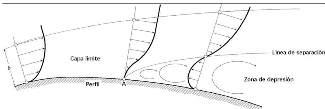
Fig. 3.2 Proceso de separación y desprendimiento de la capa límite.
