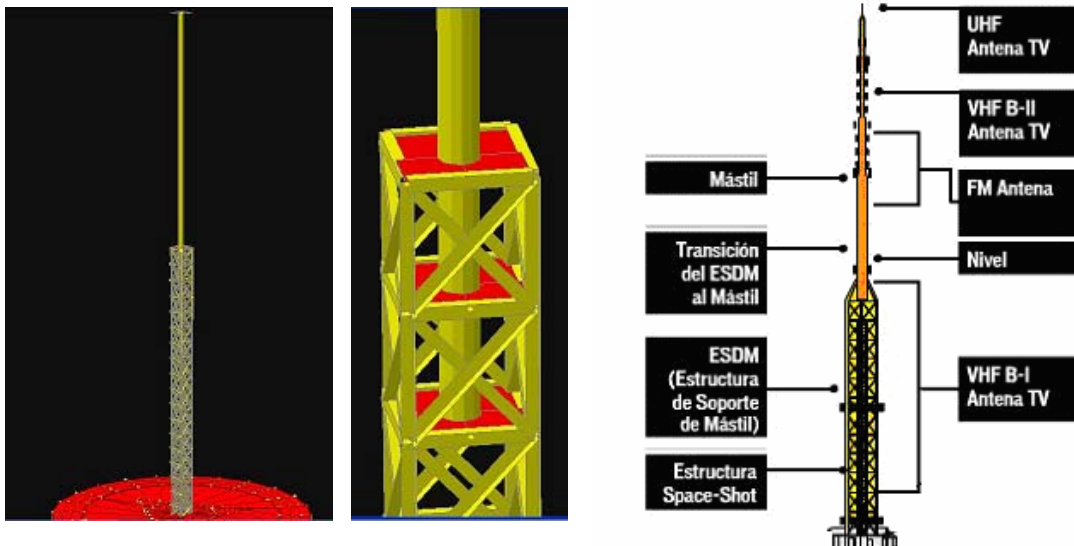
FIG. 7.3 Aspectos de la antena superior de la torre.
