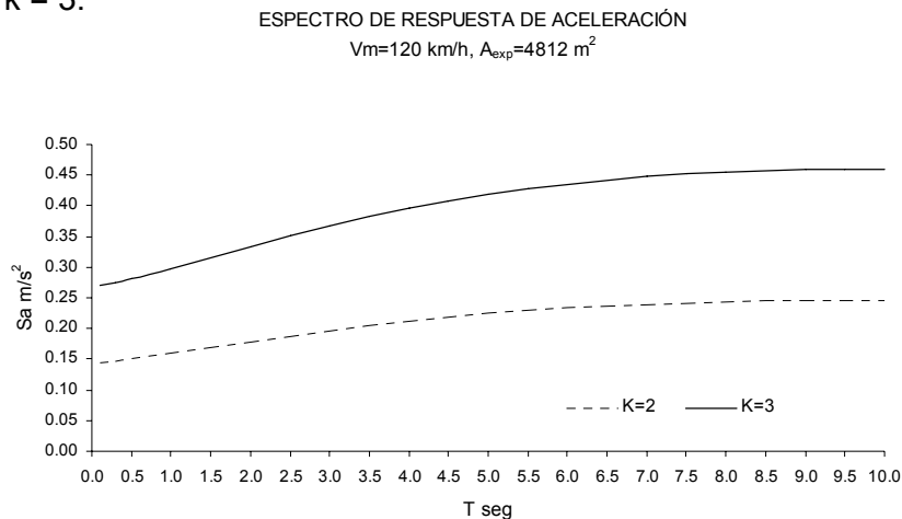
FIG. 7.12 Espectro de Aceleraciones de respuesta producidos por el viento.
