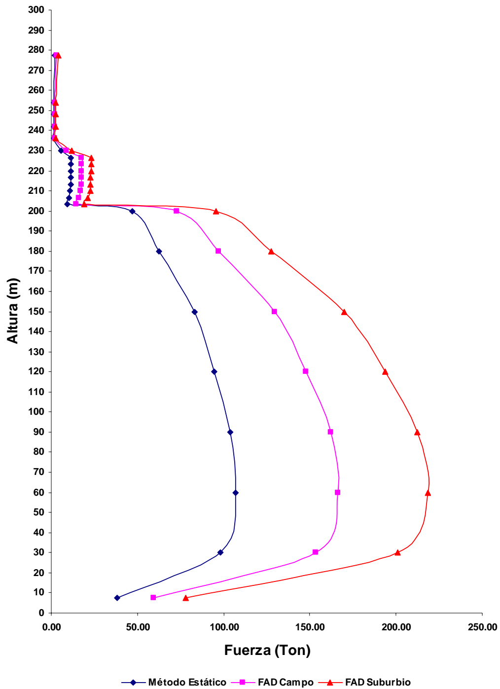
FIG. 7.14 Variación de las fuerzas inducidas por el viento en la torre.
