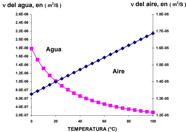
Fig. 1.7 Viscosidad Cinemática del agua y del aire a presión atmosférica al nivel del mar 4 .
