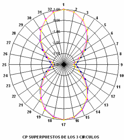
Fig. 6.18. Cp para una Separación de 3D
