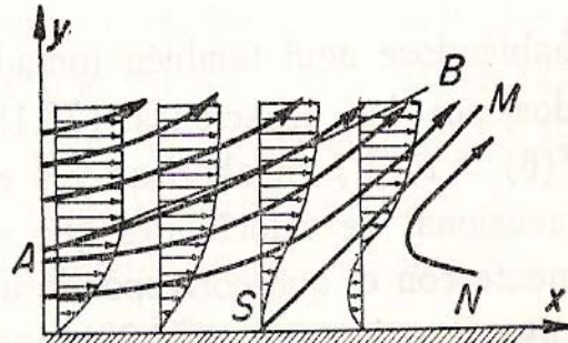
Fig. 3.1 Proceso de separación.
