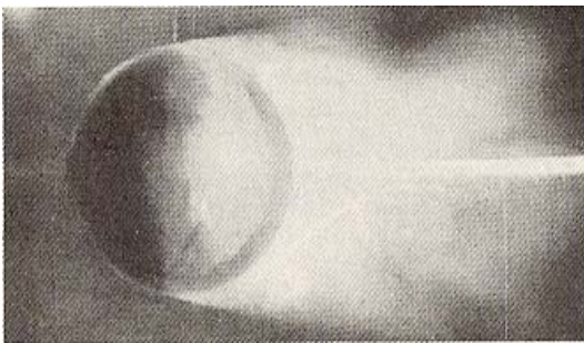
Fig. 3.39.- Flujo alrededor de la esfera debajo del punto crítico (Wieselsberger.)
