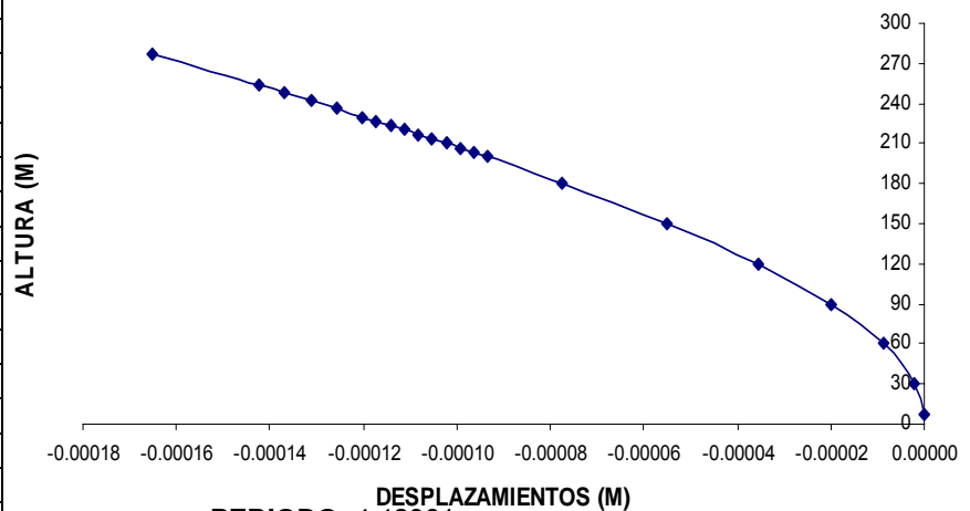
FIG. 7.6 CONFIGURACION MODAL DE LA TORRE CON TIRANTES
