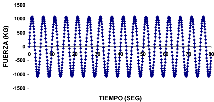
FIG. 7.16 Fuerza Senoidal correspondiente a cada nodo de la proyección transversal de la cabina.
