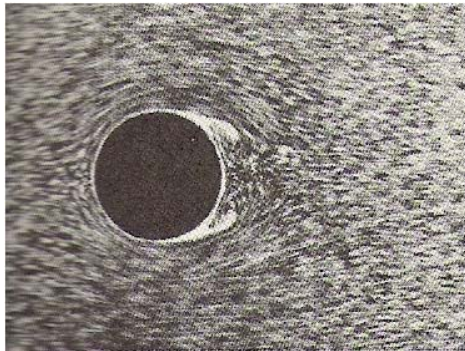
Fig. 3.8.- Formación de dos vórtices; flujo que se rompe flojamente del cilindro.
