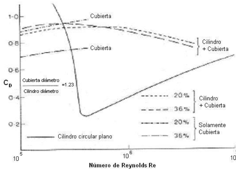
Fig. 5.4 Coeficiente de arrastre C_D contra número de Reynolds en los intervalos Supercríticos y Poscríticos
