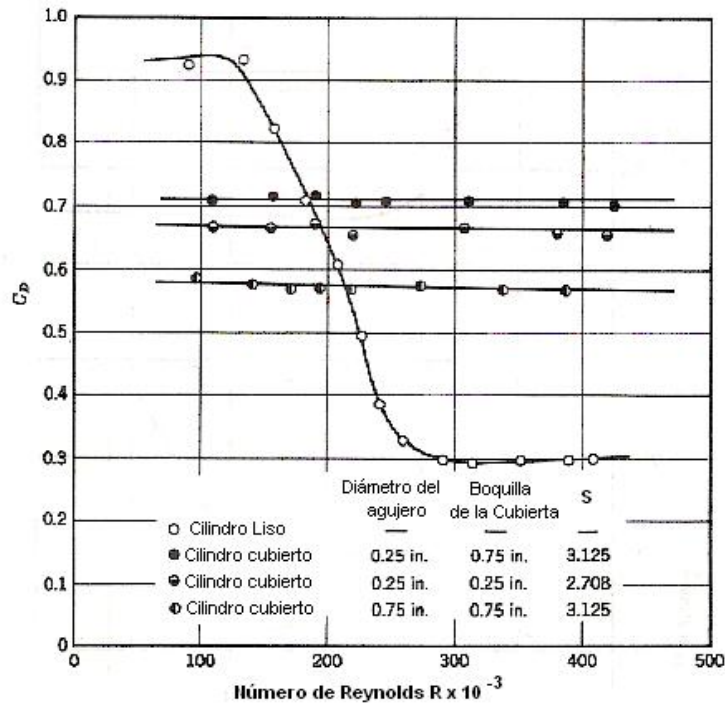
Fig. 5.3 Coeficiente de arrastre C_D para cilindros contra número de Reynolds con diámetro de 6 in
