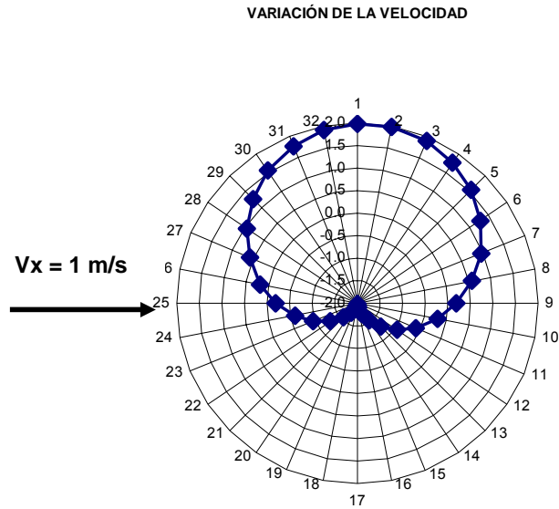
Fig. 6.6 Variación de la velocidad en un cilindro con flujo laminar en dirección (V_x, 0) .
