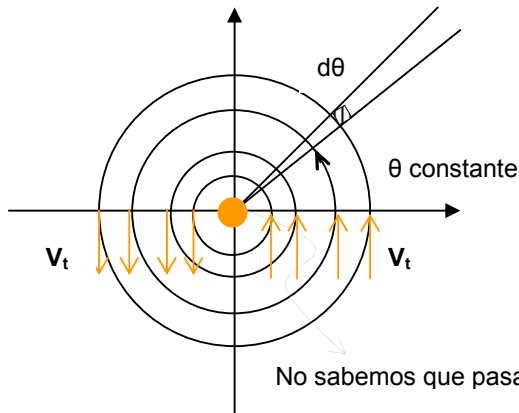
Fig. 1.25 A este flujo se le conoce como "Vórtice libre".
