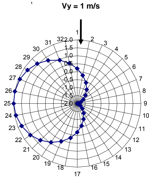
Fig. 6.8 Variación de la velocidad en un cilindro con flujo laminar en dirección (0, -V_y) .
