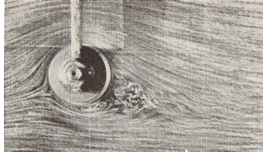
Fig. 3.18.- u/v = 2.0
