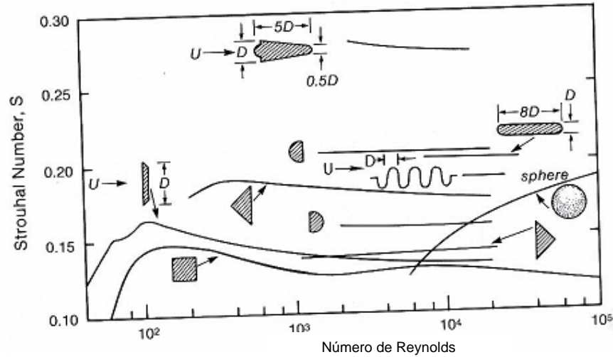
Fig. 4.5.- Número Strouhal para secciones no circulares. El Flujo es de izquierda a derecha.
