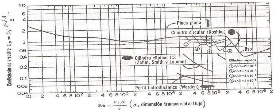
Fig. 2.4 Coeficientes de arrastre total para cuerpos bidimensionales
