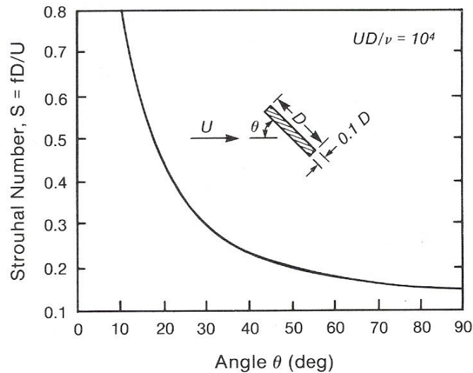
Fig. 4.6.- Número Strouhal para una placa plana inclinada.
