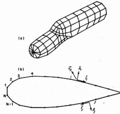
Fig. 6.2. Discretización de la superficie del cuerpo. (a) Cuerpo tridimensional con fuentes elementos de frontera bidimensionales. (b) Cuerpo bidimensional con líneas rectas como elementos de frontera.
