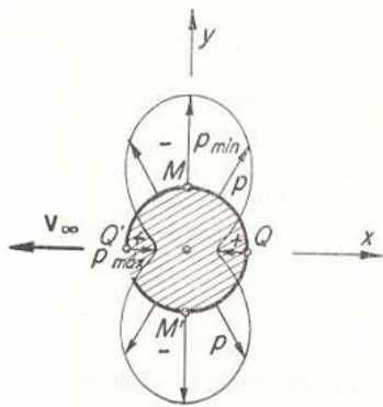
Fig. 1.39 Distribución del C_p para un cilindro inmerso en Flujo Irrotacional.
