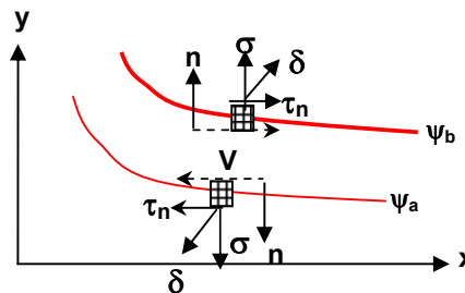
Fig. 1.14 Esfuerzos de interacción entre el fluido en movimiento y las líneas de corriente.
