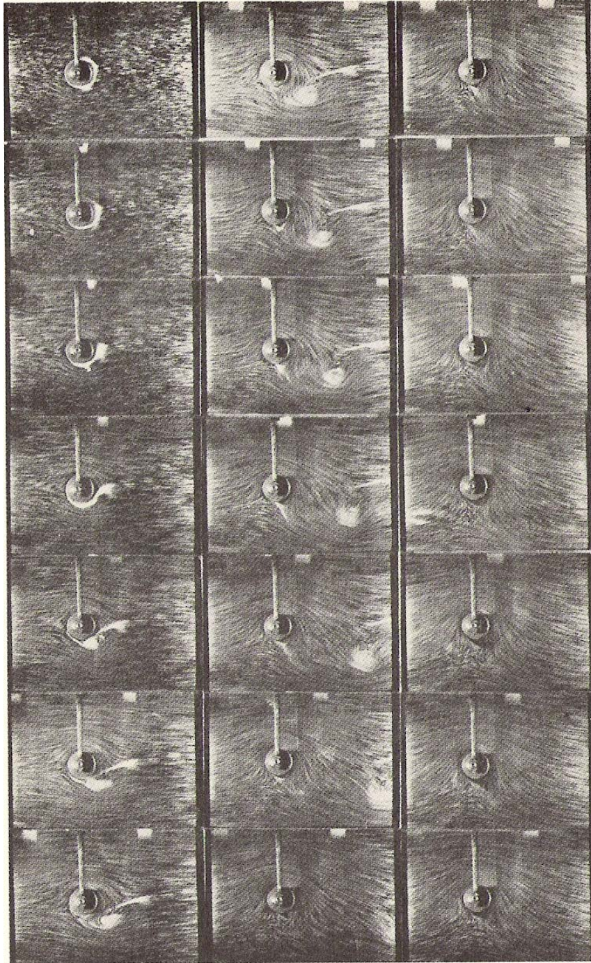
Fig. 3.13.- Fotografías consecutivas del flujo alrededor de un cilindro que rota (con circulación) que empieza del reposo. La relación de la velocidad periférica de rotación u a la velocidad delantera v es u/v = 4.0 , (ref. 1).
