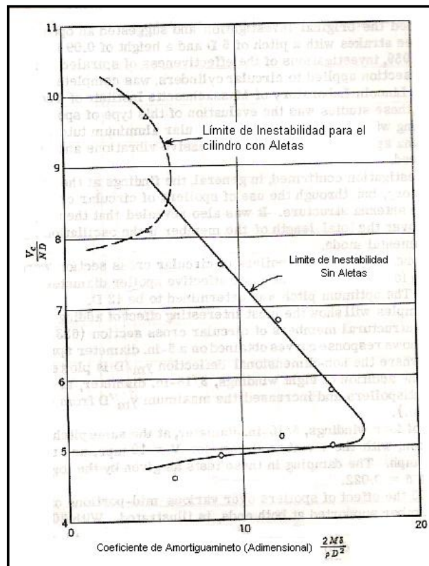
Fig. 5.6 Límite de Inestabilidad para un tubo con y sin aletas
