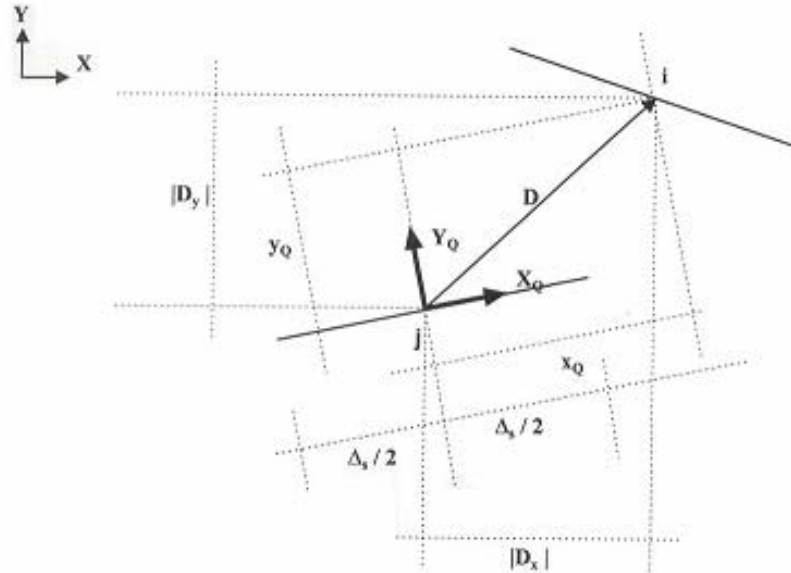
Fig. 6.3 Relación entre las coordenadas globales X, Y y las locales de cada panel.
