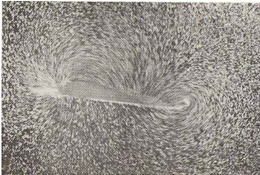
Fig. 3.57.- Como la Fig. 3.54; pero la cámara fotográfica esta quieta con respecto al fluido no perturbado.
