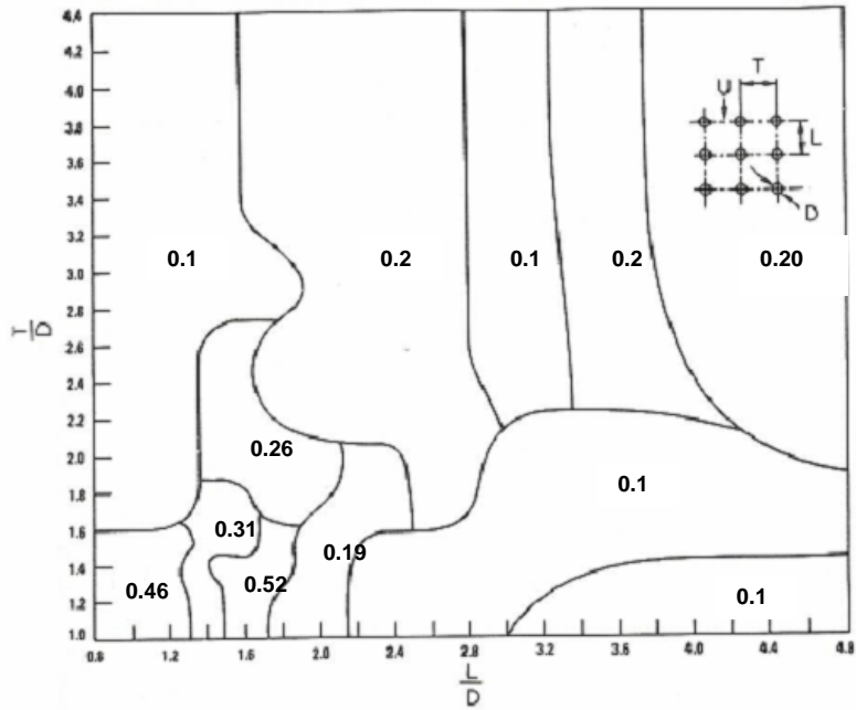
Fig. 4.3.- Número de Strouhal para arreglos de cilindros en línea (Fitzhugh, 1973).
