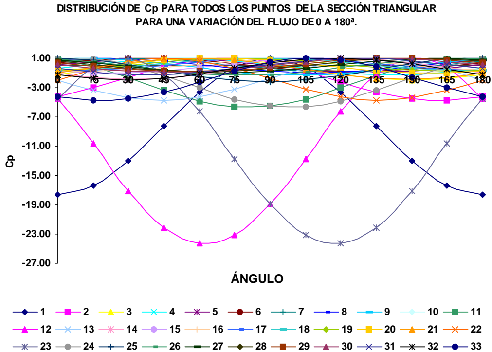
FIG. 7.11 Variación de coeficientes locales de presión, con la dirección del viento
