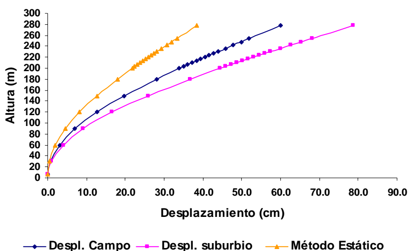
FIG. 7.13 Desplazamientos medios producidos por el viento en la torre.
