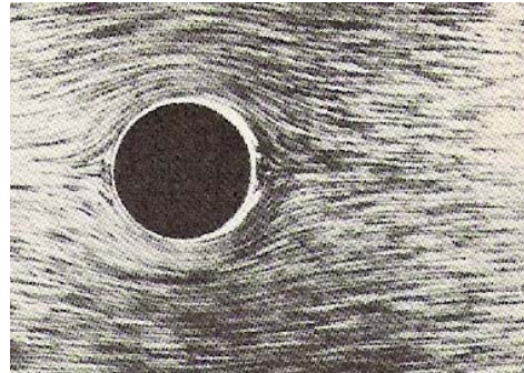
Fig. 3.7.- Flujo posterior en la capa límite detrás del cilindro; acumulación del material de la capa límite.
