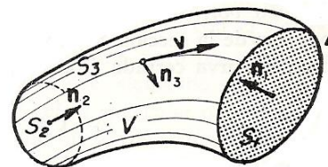
Fig. 1.8 Tubo de flujo.
