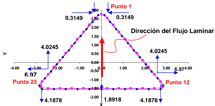
FIG. 7.10 Distribución de las fuerzas de arrastre en el semicuerpo de sección transversal triangular.
