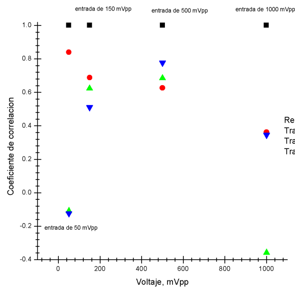
Fig 44. Coeficiente de correlación cruzada en función del voltaje de entrada del pulso senoidal de 1 ciclo al amplificador RF.
