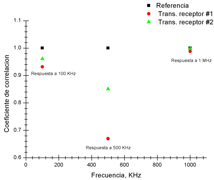
Fig 39. Coeficiente de correlación en función de la frecuencia de tres señales adquiridas, variando la frecuencia del pulso senoidal emitido de un ciclo de duración en 0.1, 0.5 y 1 MHz
