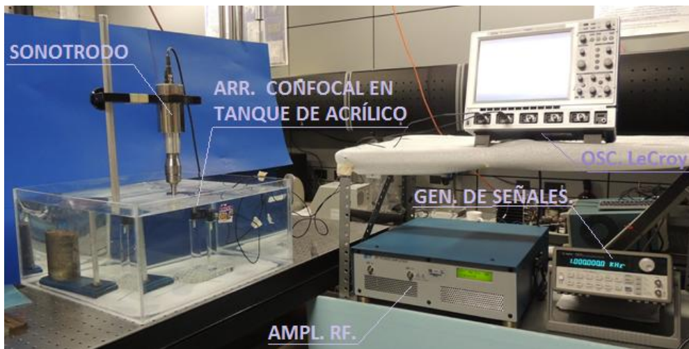
Fig 26. Arreglo experimental empleando el Sonotrodo como emisor de frecuencia variable.
