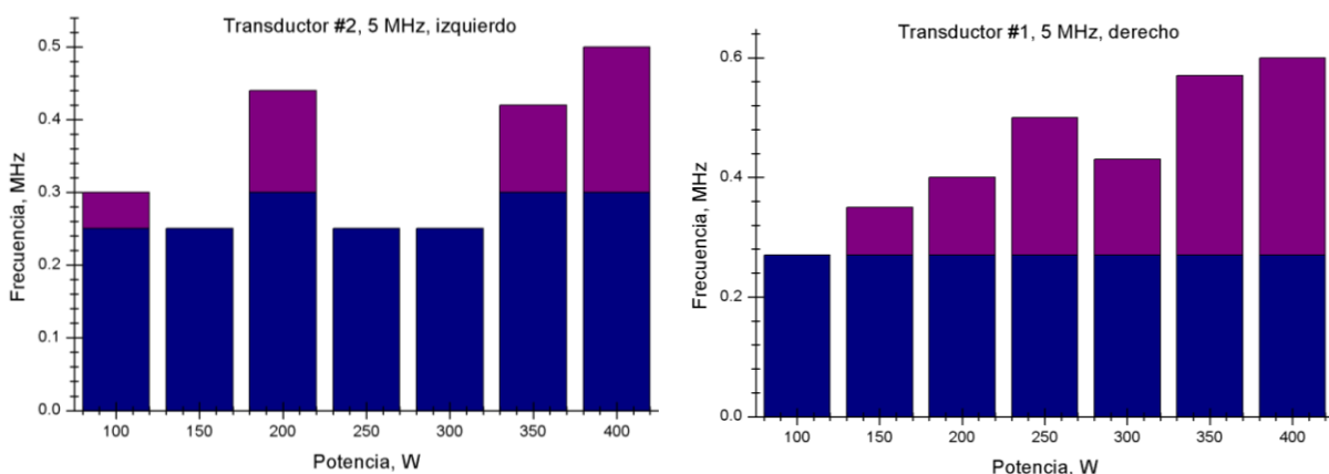
Fig 56. Curvas de frecuencia en función de la potencia suministrada al Sonotrodo, para los transductores de recepción.
