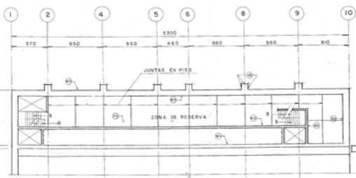
PLANTA NIVEL 166.40 y 166.00
