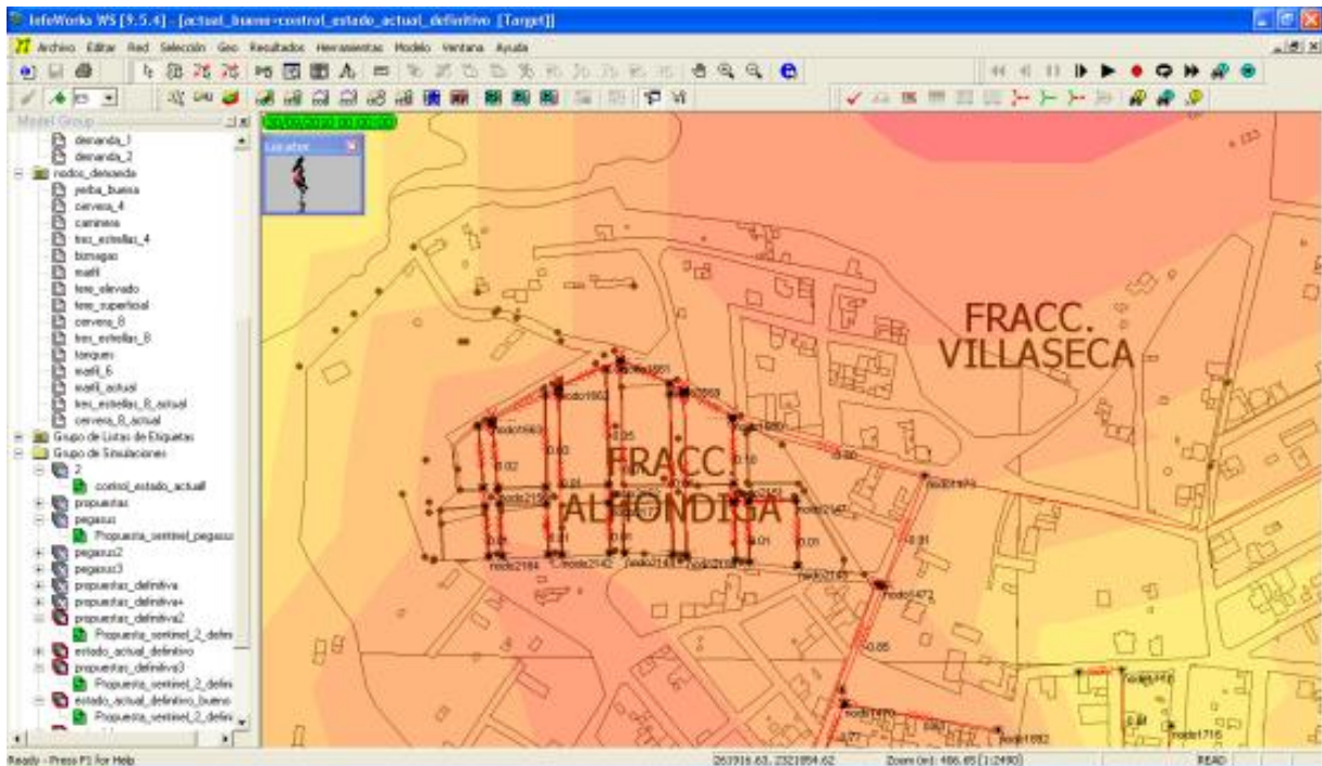
Figura 4.45 Contorno de presiones mayores a 5 Kg/cm 2
