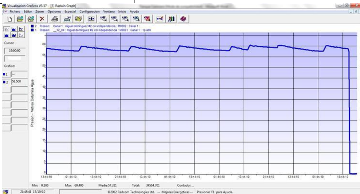
Figura 4.13 Medición de presión en Miguel Domínguez, Col. Independencia
