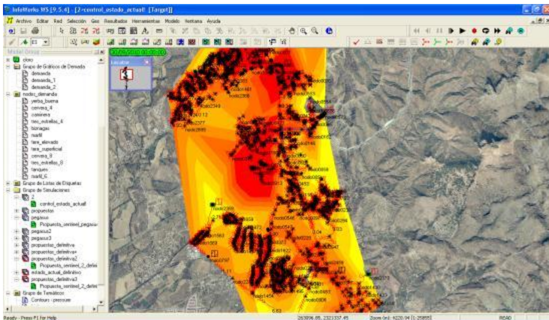
Figura 4.44 Contorno de presiones
