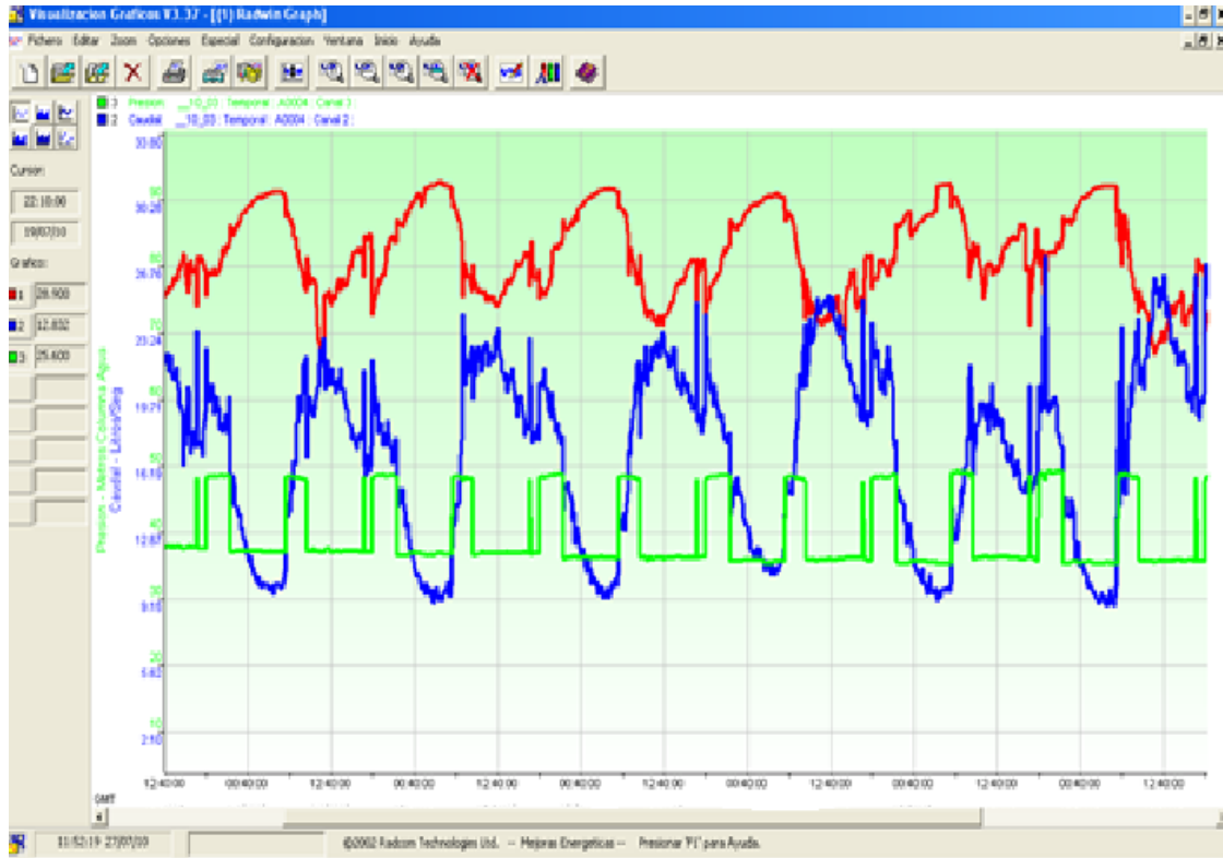
Figura 5.10 Cambios que realiza el controlador inteligente
