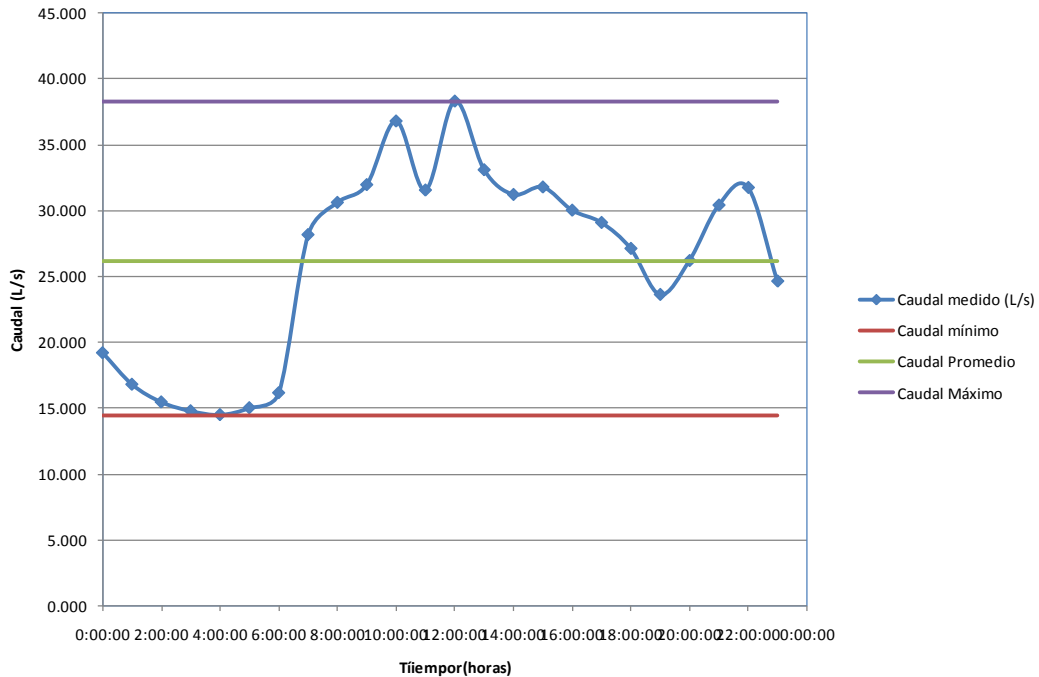
Figura 4.2 Curva de demanda de la salida de 8" del Tanque Tres estrellas
