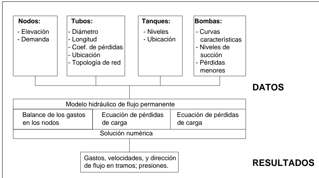
Figura 3.4 Diagrama de un modelo hidráulico de flujo permanente
