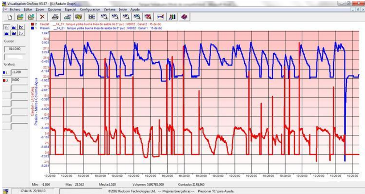
Figura 4.10 Medición de presión en calle La Quinta, Fracc.M de la Hacienda
