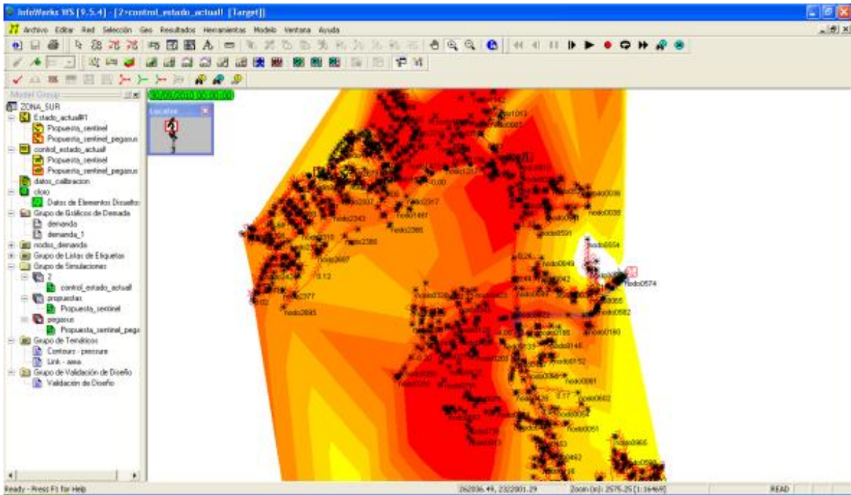
Figura 4.32 Simulación inicial
