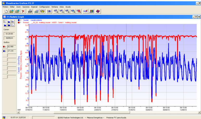
Figura 5.5 Gráfico en la primera Etapa de Medición
