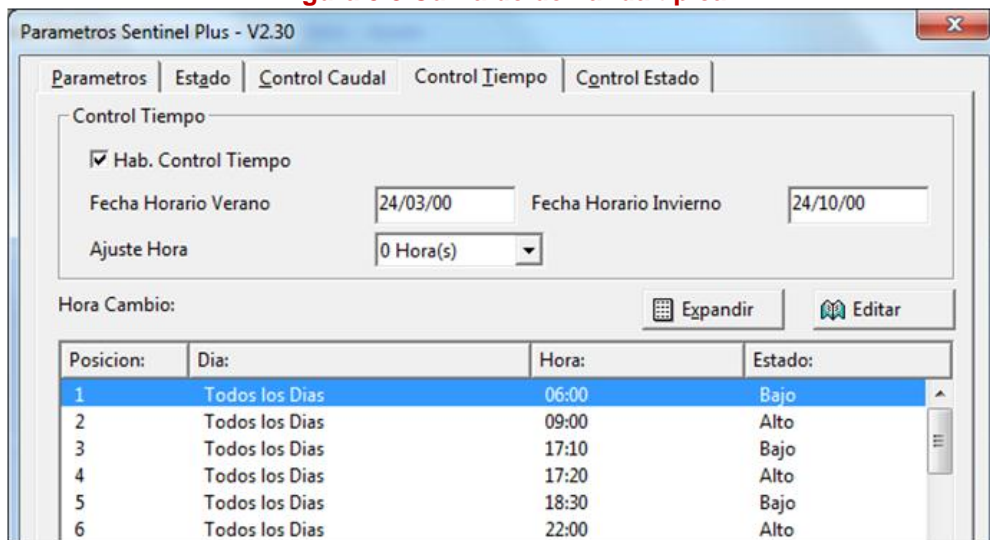
Figura 5.9 Parámetros del controlador
