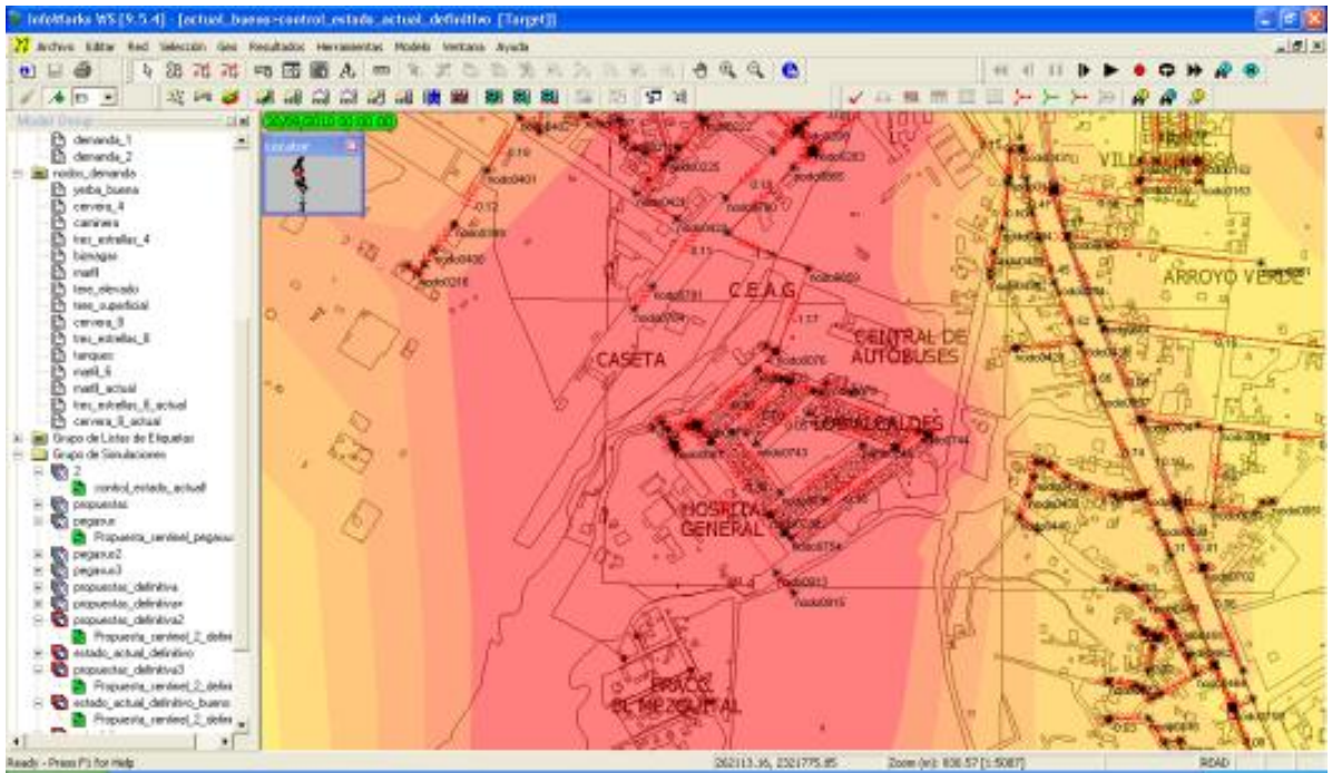
Figura 4.46 Contorno de presiones mayores a 5 Kg/cm 2
