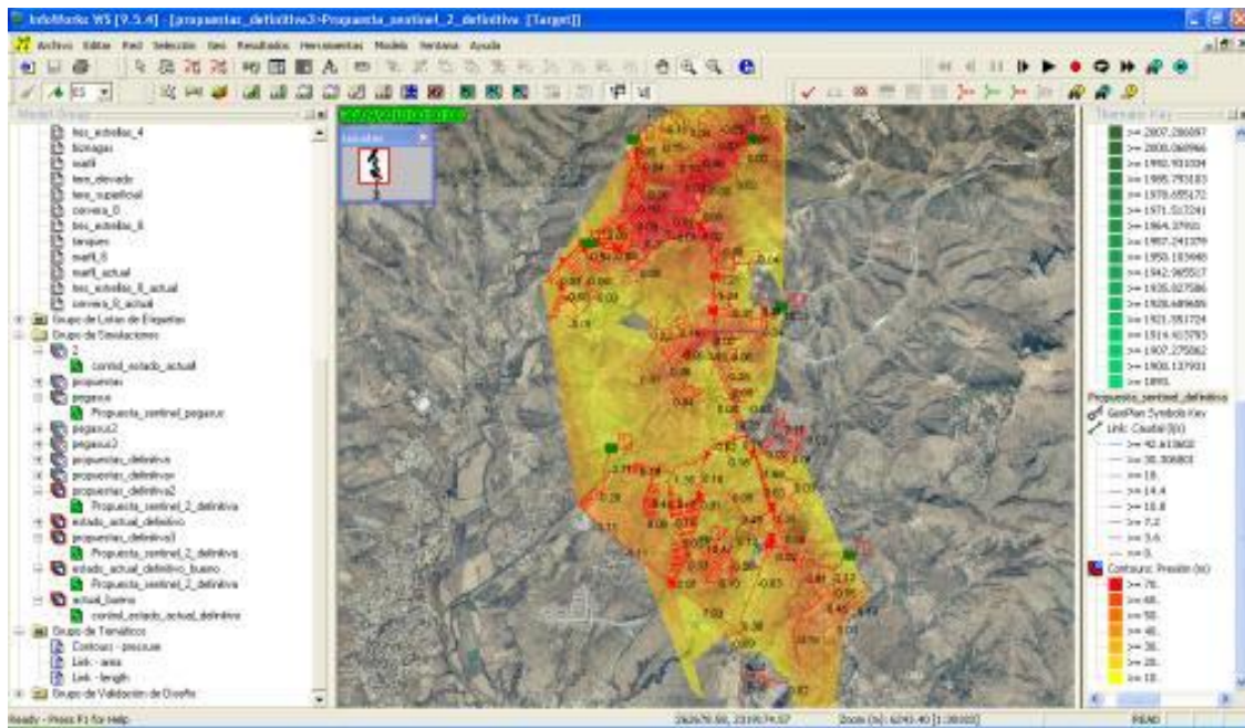
Figura 4.53 Contorno de presiones propuesto para la zona sur
