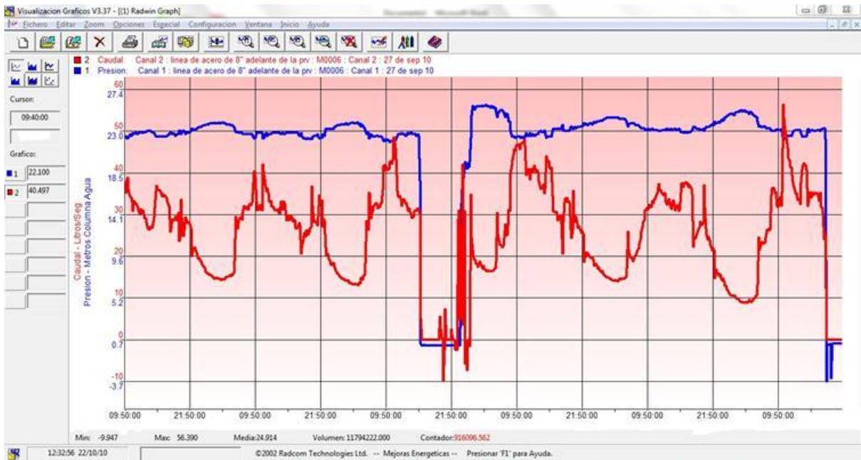
Figura 4.7 Medición de caudal y presión a la salida del tanque Tres Estrellas
