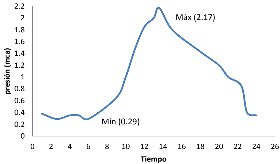
Figura 3.1. Medición de distritos hidrométricos
