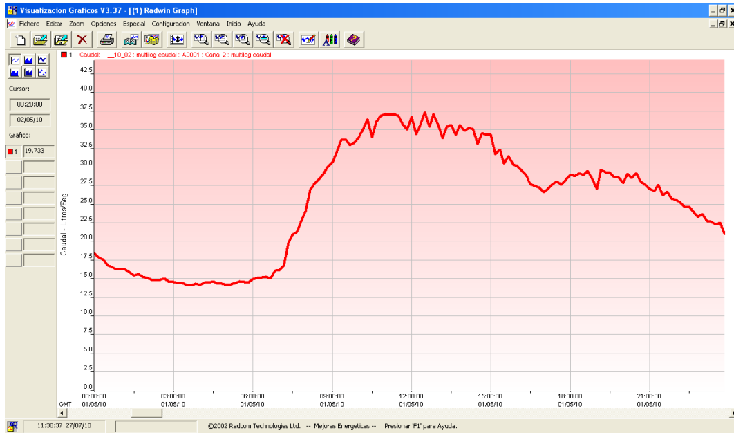
Figura 5.8 Curva de demanda típica
