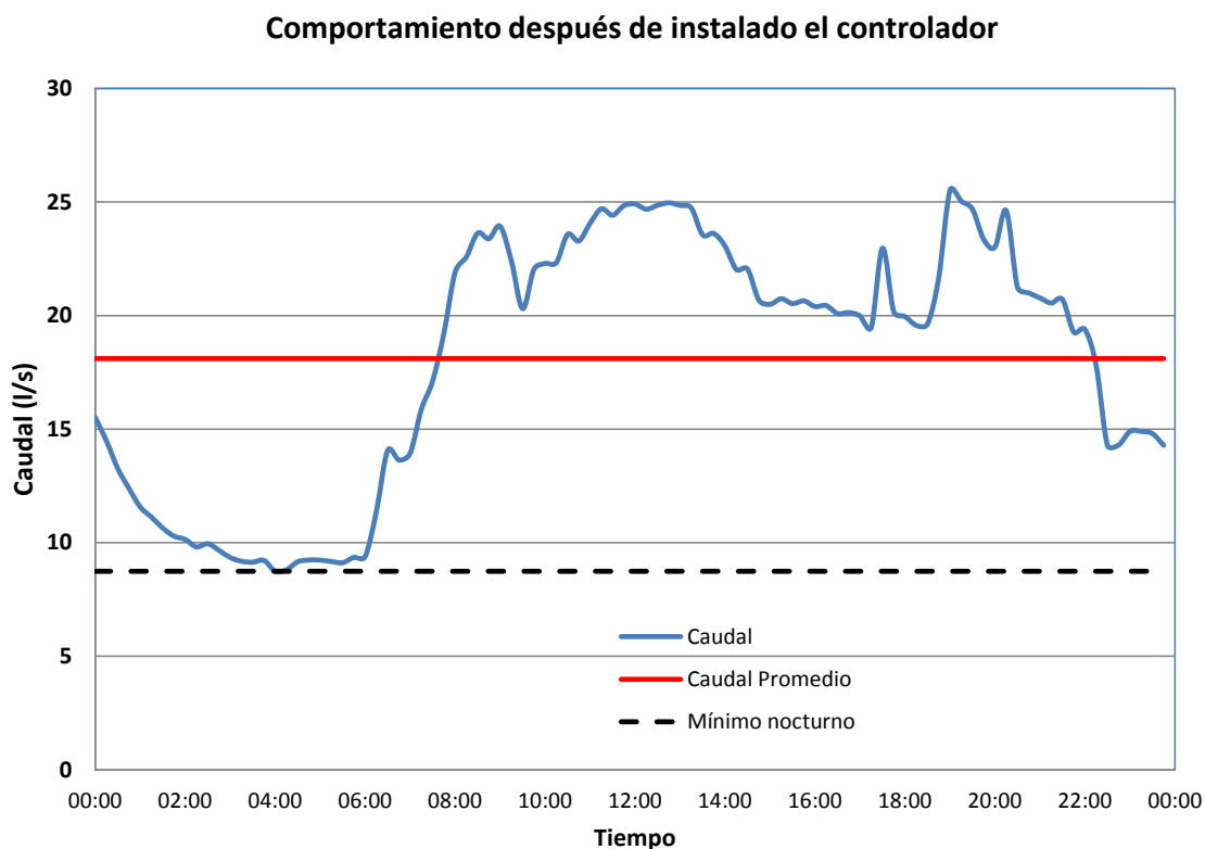
Figura 5.13 Gráfica después de la instalación del controlador
