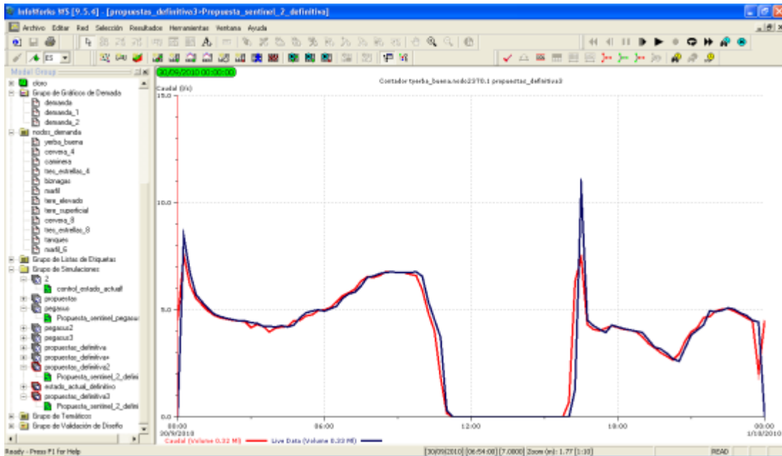
Figura 4.43 Tanque Yerba Buena, tubería de 6"
