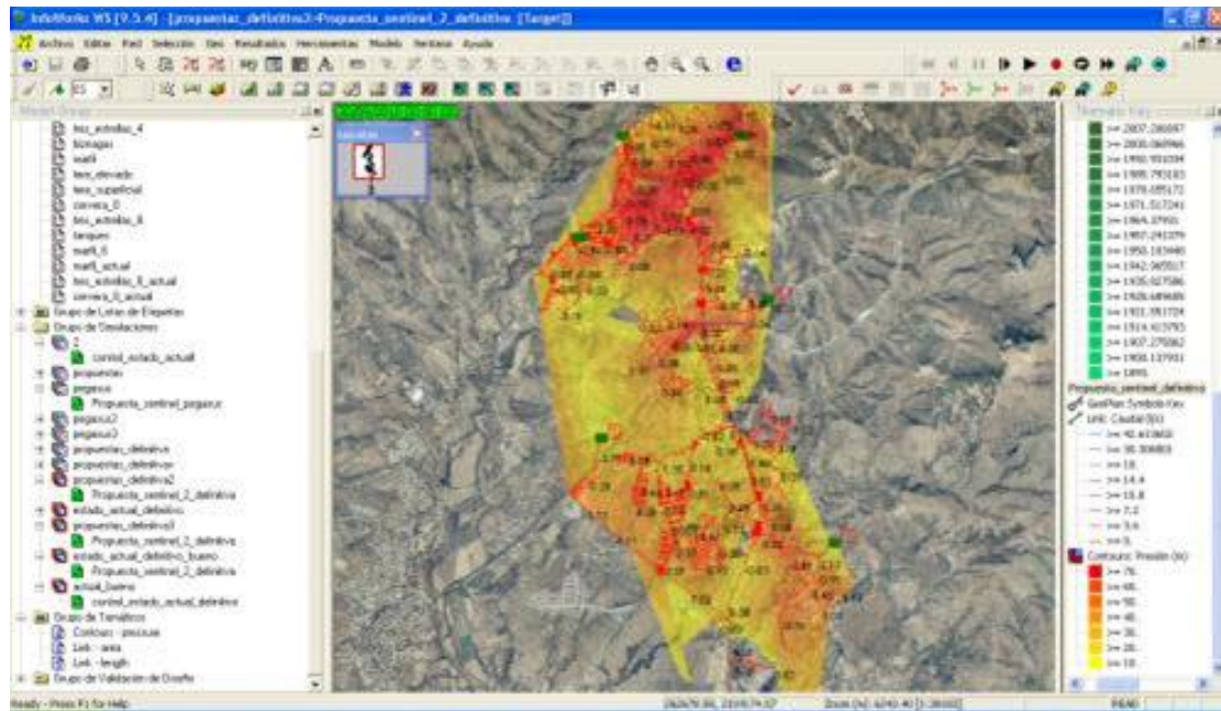
Figura 6.2 Contorno de presiones propuesto para la zona sur
