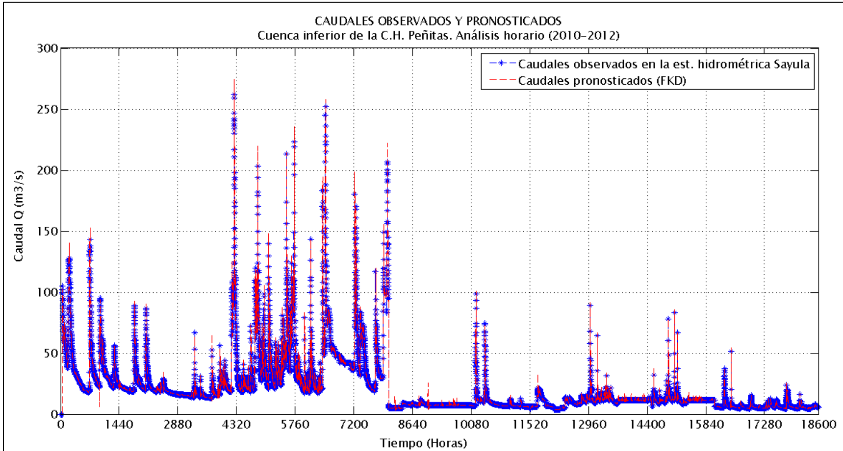
Figura 5.40 Caudales observados y pronosticados de la cuenca inferior de la C.H. Peñitas, considerando la función de respuesta modificada.
