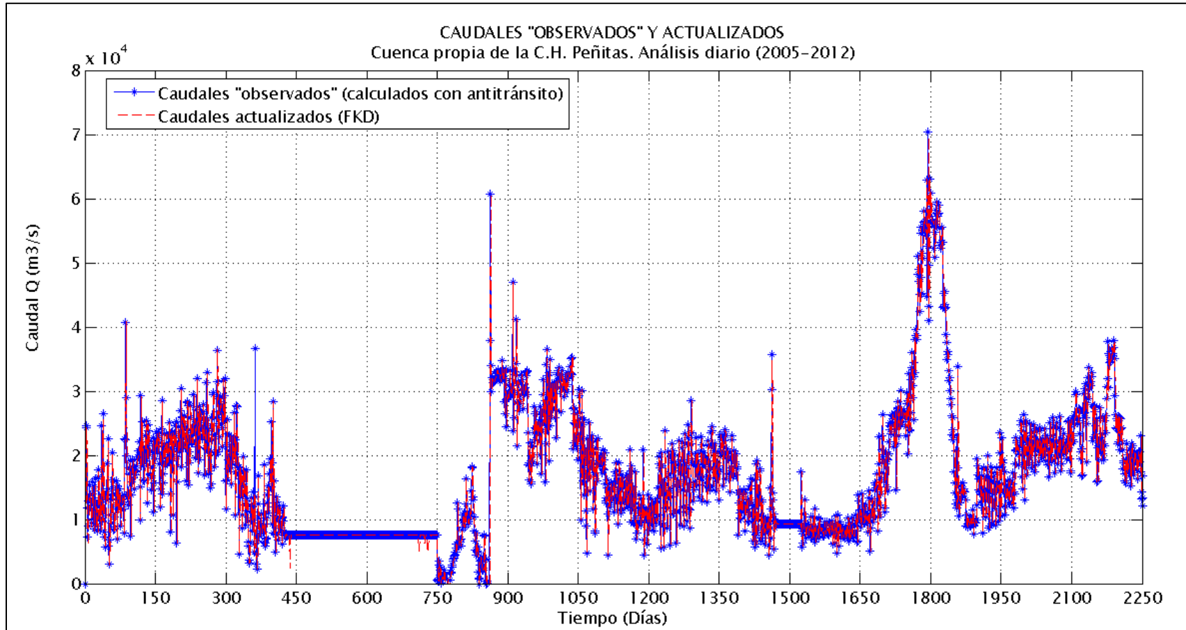
Figura 5.72 Caudales "observados" y actualizados en la cuenca propia de la C.H. Peñitas. Análisis diario, considerando la función de respuesta modificada.
