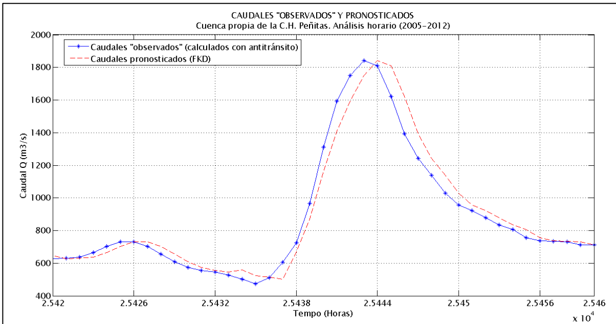
Figura 5.36 Caudal “observado” y pronosticado con FKD (Avenida B), aplicado a la cuenca propia de la C.H. Peñitas, considerando la función de respuesta igual al HUI, y S = Desv. est. (X_f - X_u) \cdot [I]_{n \times n} .
