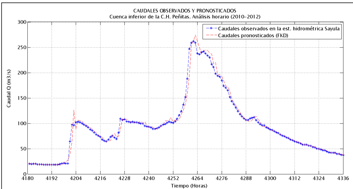
Figura 5.51 Caudal observado y pronosticado con FKD (Avenida A) para la cuenca inferior de la C.H. Peñitas, considerando la función de respuesta modificada.
