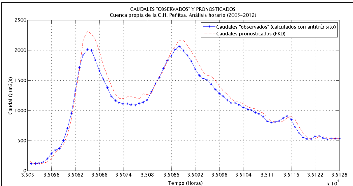
Figura 5.37 Caudal “observado” y pronosticado con FKD (Avenida C), aplicado a la cuenca propia de la C.H. Peñitas, considerando la función de respuesta igual al HUI, y S = Desv. est. (X_f - X_u) \cdot [I]_{n \times n} .
