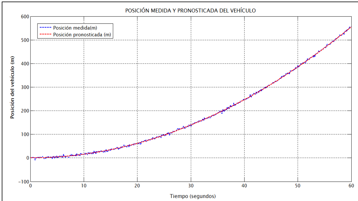
Figura 3.3 Posición medida y pronosticada de un vehículo en movimiento, aplicando el algoritmo del FKD.
