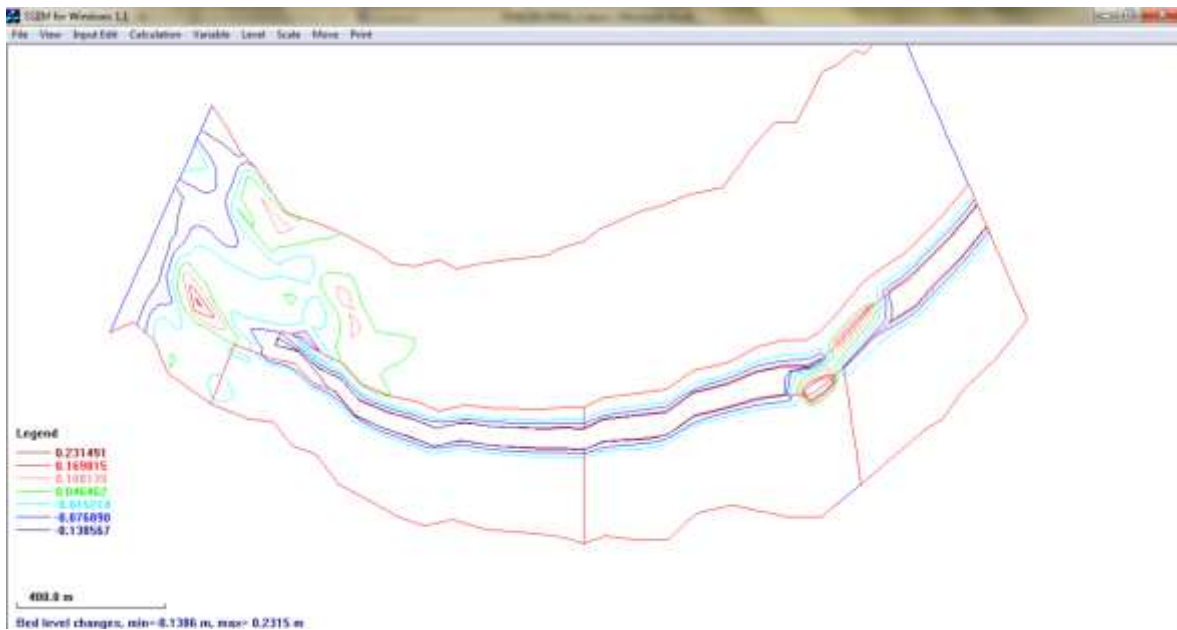
Figura 4.11 Cambios en el lecho D_{50} = 0.2 mm en condiciones iniciales
