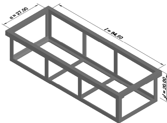
Figura III-3 Charola para la colocación del suelo dentro del canal de oleaje (Acotaciones en cm)
