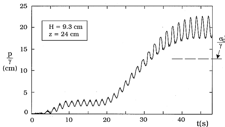
Figura II-15 Registro de presión de poro: transición de no licuefacción a licuefacción (Sumer et al. , 2012)
