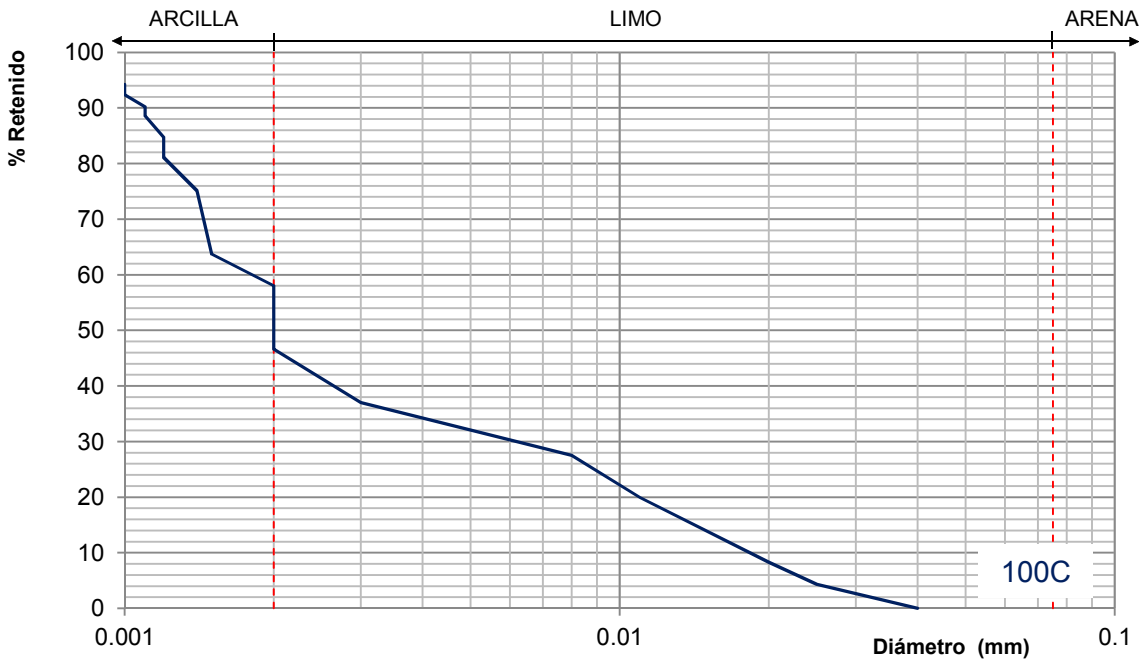
Figura III-15 Curva granulométrica del material fino: caolín comercial
