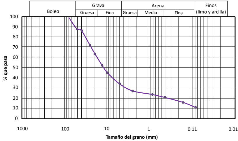
Figura 5.2. Distribución granulométrica del sitio (modificada de Rollins et al, 2005).
