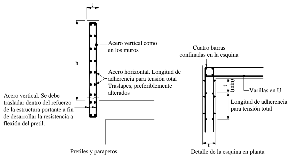
Detalle B.31 Parapetos de mampostería y pretiles (continuación) [Dowrick, 1990]
