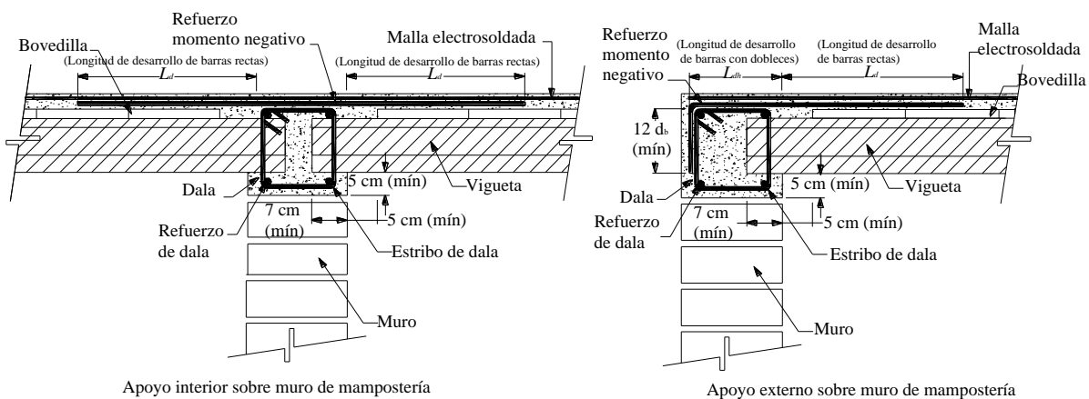
Apoyo interior sobre muro de mampostería
