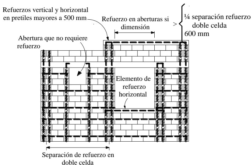
Refuerzo en aberturas y pretilas
