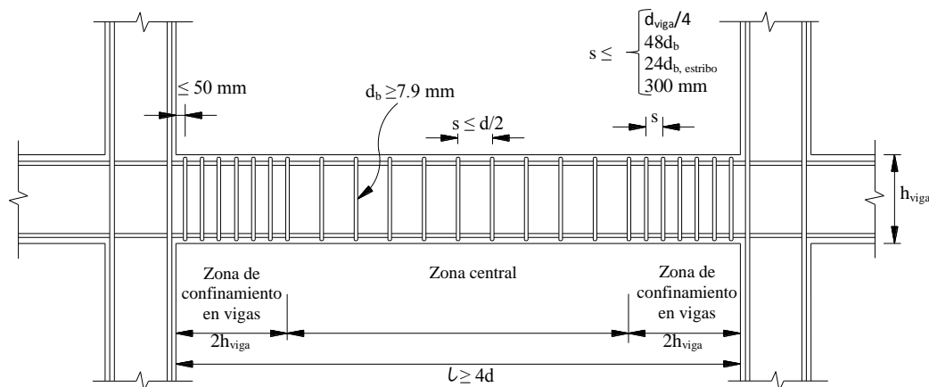
Detalle B.13 Detallado de elementos a flexión [RCDF, 2004]
