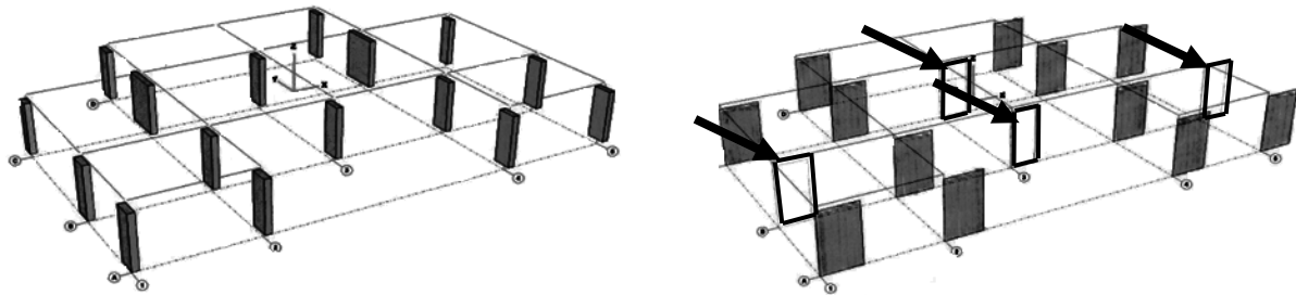
Figura 3.4 a) Distorsión de entrespacio PB-primer nivel y b) resistencia de columnas en planta baja
