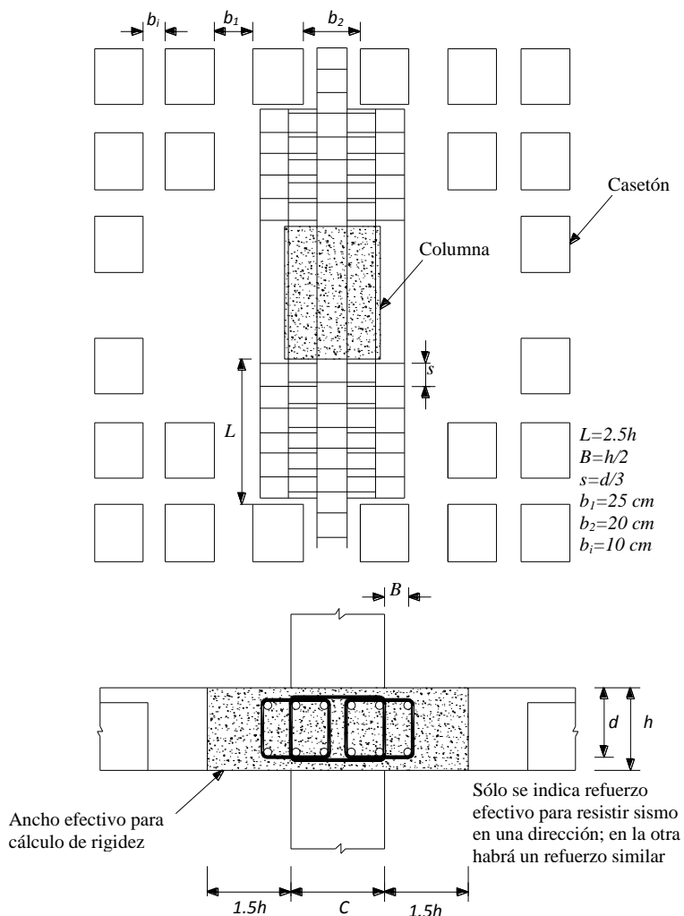
Detalle B.14 Losas aligeradas [RCDF, 2004]
