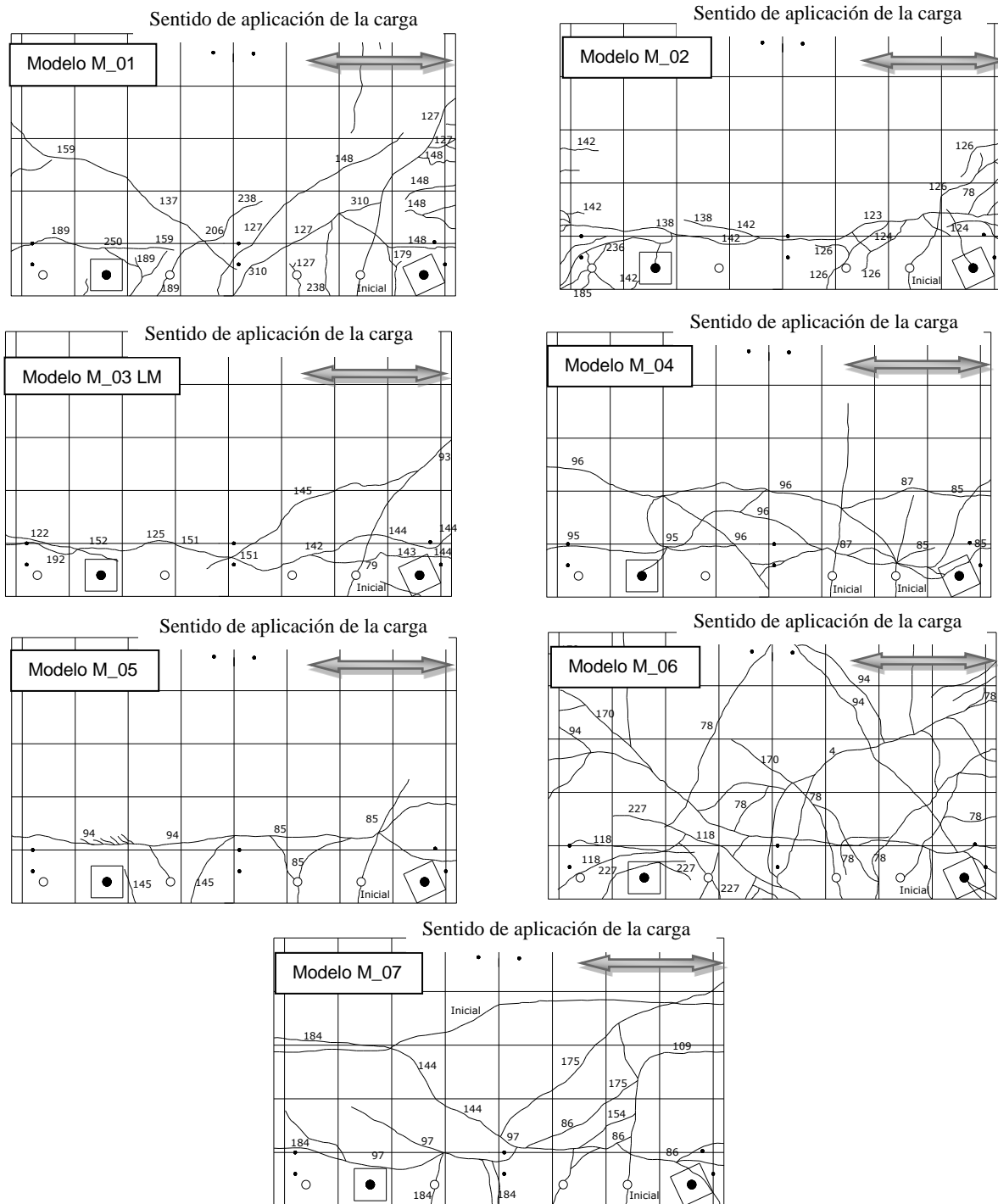
Fig.4.1. Patrones de agrietamiento final de los siete modelos (prueba a flexión)
