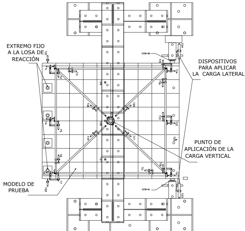
Prueba flexión-cortante.
