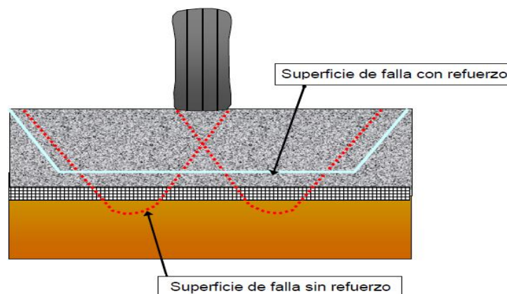
Figura 1.3. Mecanismo de reforzamiento de capacidad portante.
