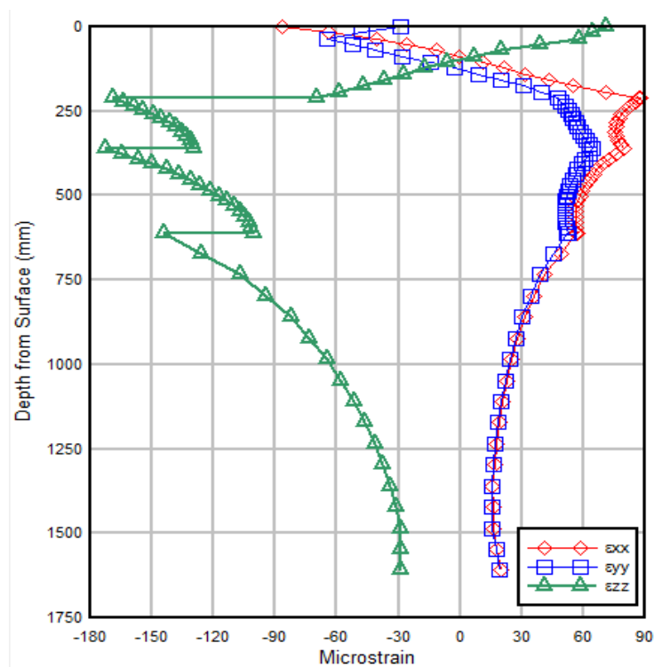
Figura 4.5. Gráfica estándar de deformaciones unitarias sección uno.
