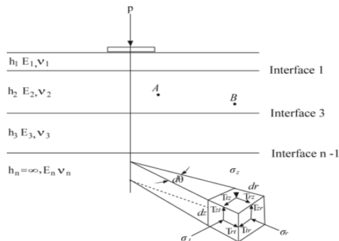
Figura 3.2. Sistema general del sistema multicapa elástico. 45
