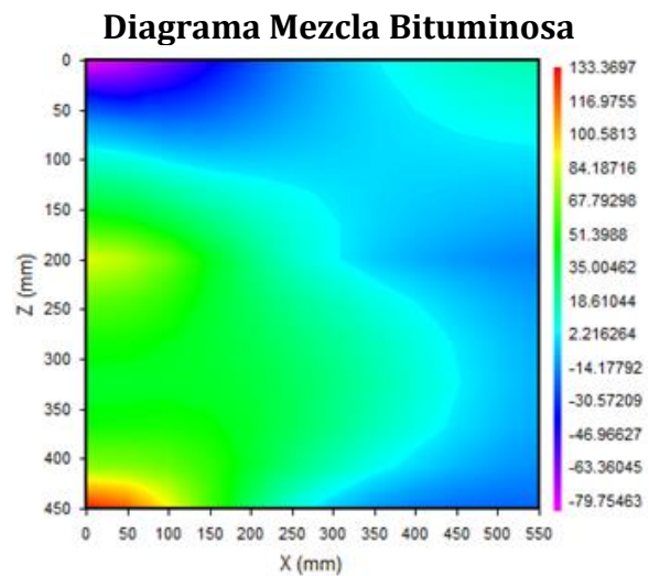
Figura 4.8. Diagrama de deformaciones tangenciales de la mezcla bituminosa de sección 2.
